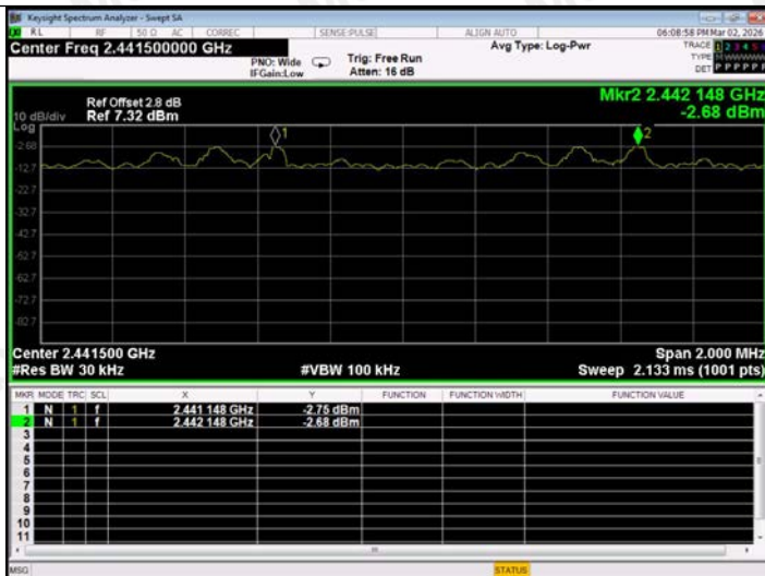
\pi/4 DQPSK
