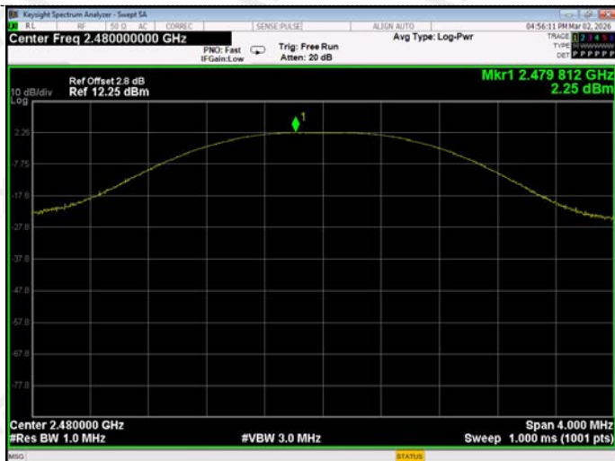
GFSK(CH78)
