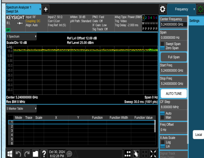
NTNV-11N20MIMO-Ant1-5240
