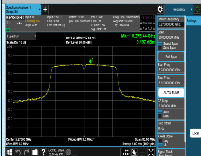
11N40SISO-Ant1-5270-PASS
