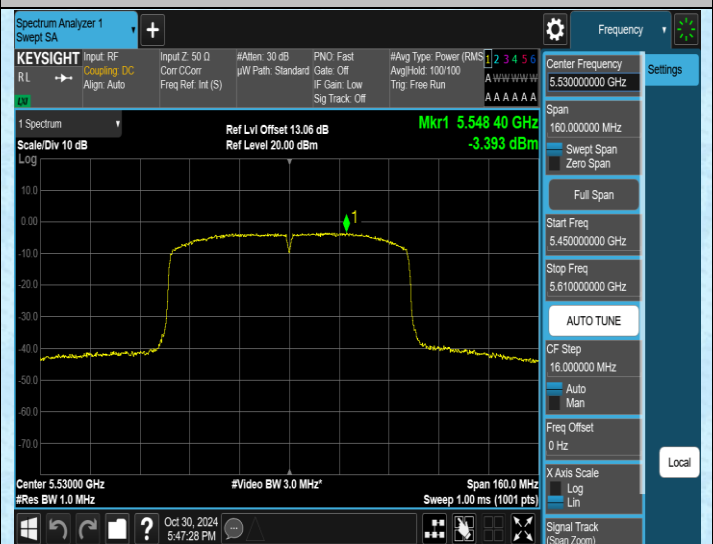
11AC80SISO-Ant2-5530-PASS
