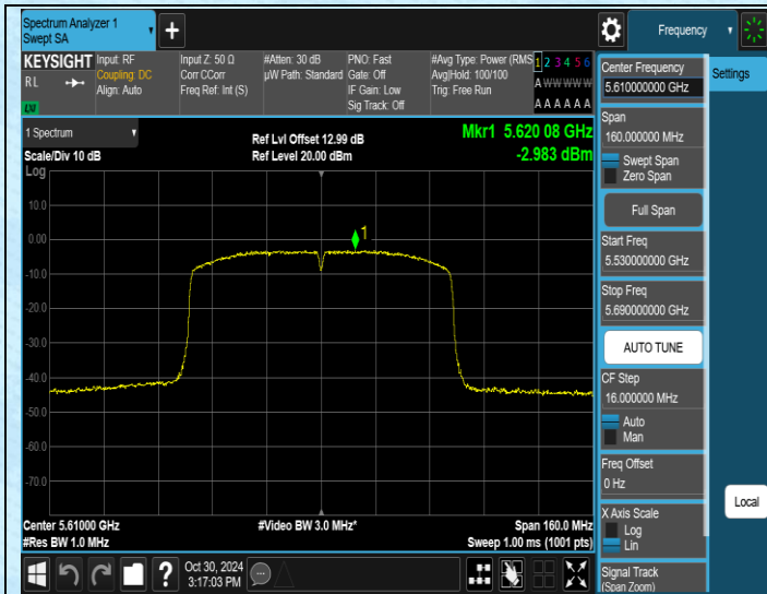
11AC80SISO-Ant1-5610-PASS
