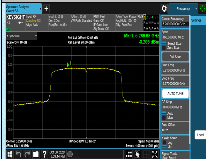
11AC80SISO-Ant1-5290-PASS
