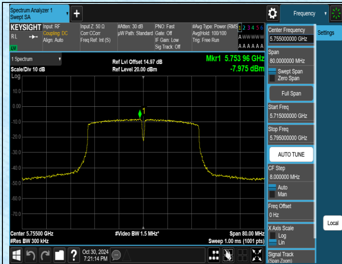
11N40MIMO-Ant1-5755-PASS
