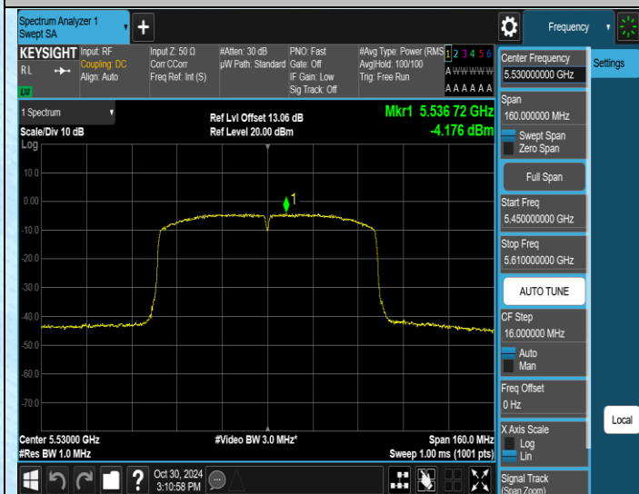
11AC80SISO-Ant1-5530-PASS
