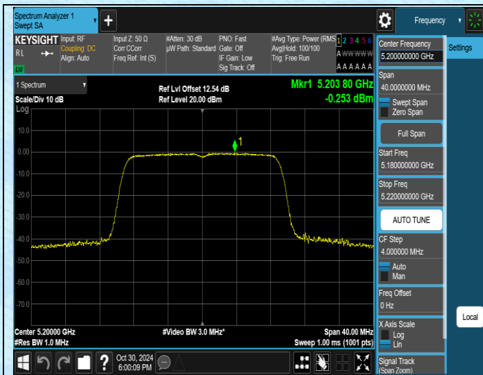
11N20MIMO-Ant1-5200-PASS
