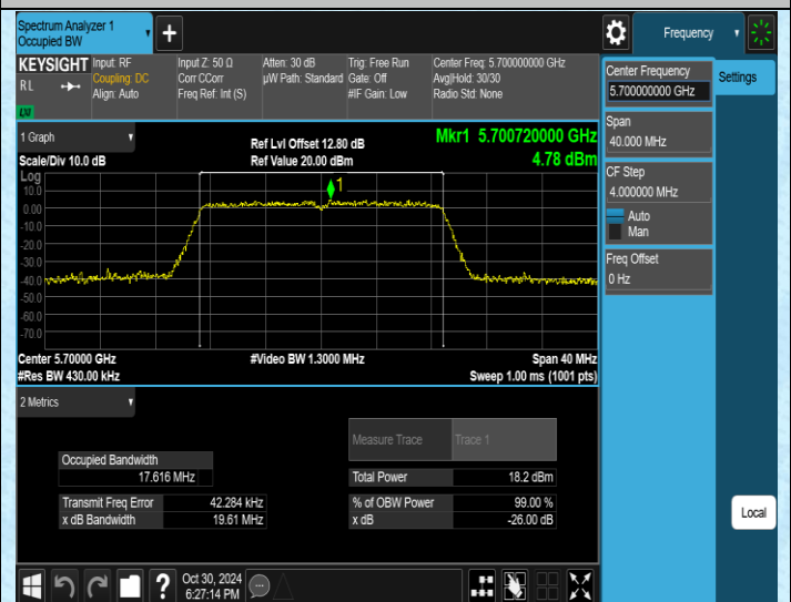
11N20MIMO-Ant2-5700
