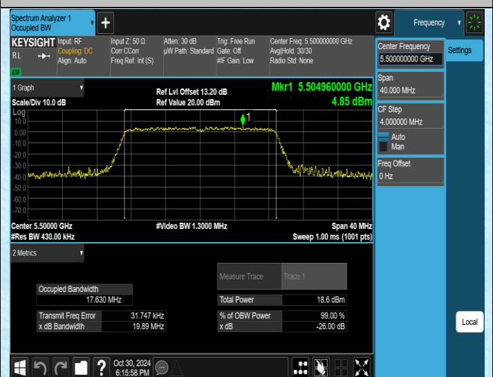
11N20MIMO-Ant2-5500
