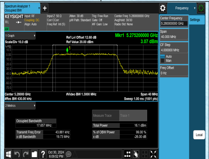
11N20MIMO-Ant2-5280
