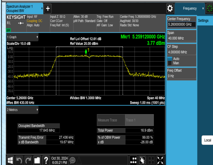
11N20MIMO-Ant1-5260
