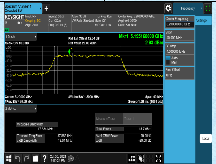
11N20MIMO-Ant2-5200
