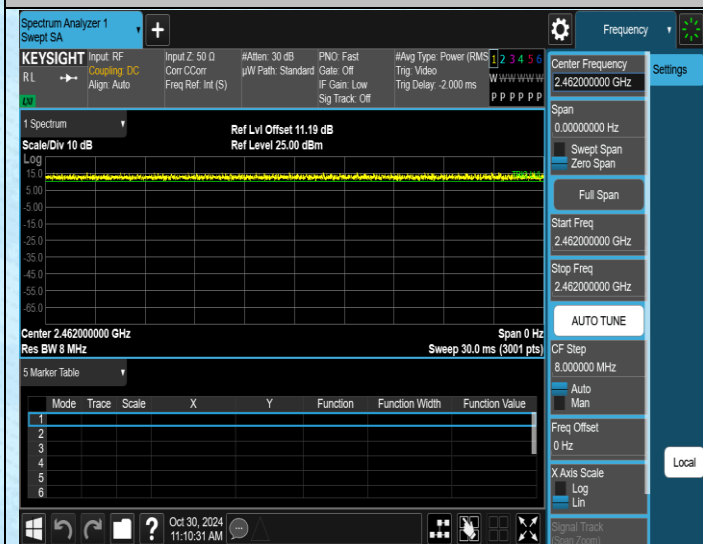
NTNV-11N20MIMO-Ant1-2462
