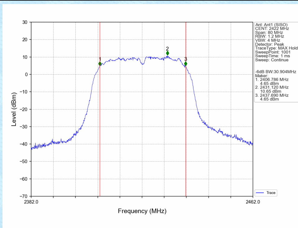
802.11n(HT40)_LCH_2422MHz_Ant1 (SISO)_NTNV
