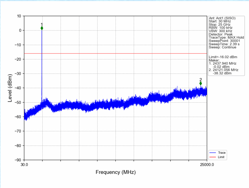
802.11g_MCH_2437MHz_Ant1 (SISO)_NTNV
