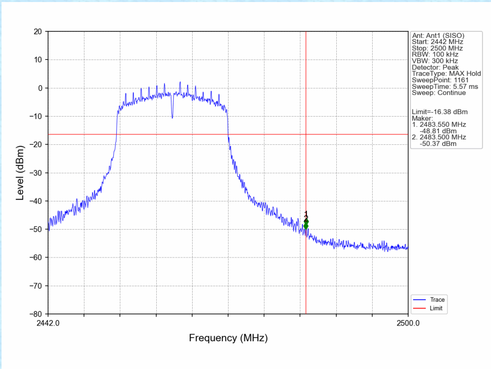
802.11n(HT20)_HCH_2462MHz_Ant1 (SISO)_NTNV
