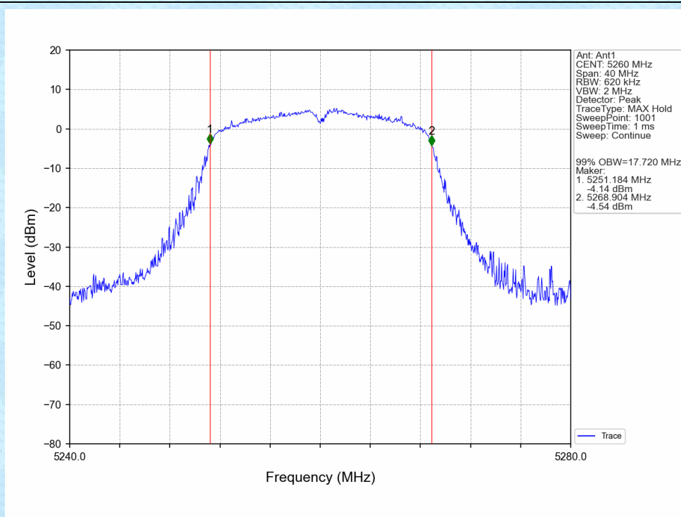
802.11n(HT20)_LCH_5260MHz_Ant1_NTNV
