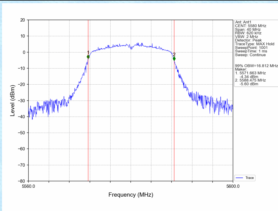
802.11a_MCH_5580MHz_Ant1_NTNV
