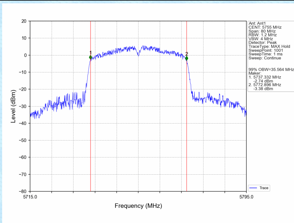
802.11n(HT40)_LCH_5755MHz_Ant1_NTNV
