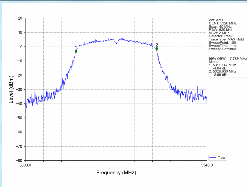
802.11n(HT20)_HCH_5320MHz_Ant1_NTNV
