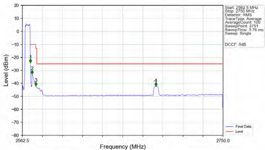
n7_15kHz_SISO_NTNV_5MHz_DFT-s-OFDM_PI/2_BPSK_2567.5MHz_Outer_Full_Ant1
