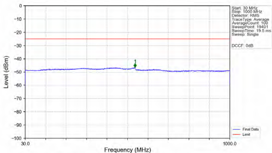
n7_15kHz_SISO_NTNV_50MHz_DFT-s-OFDM_PI/2_BPSK_2535MHz_Edge_1RB_Left_Ant1
