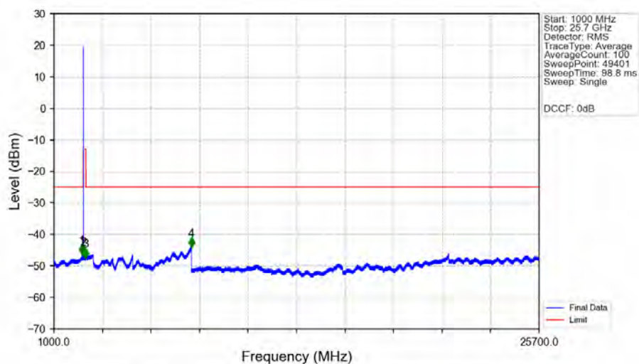
n7 15kHz SISO NTNV 50MHz DFT-s-OFDM QPSK 2525MHz Edge 1RB Left Ant1
