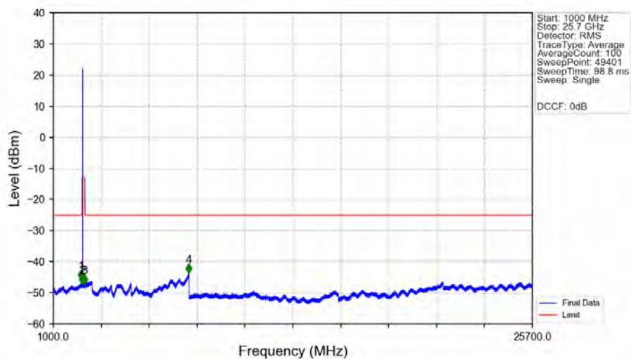
n7_15kHz_SISO_NTNV_50MHz_DFT-s-OFDM_PI/2_BPSK_2535MHz_Edge_1RB_Left_Ant1
