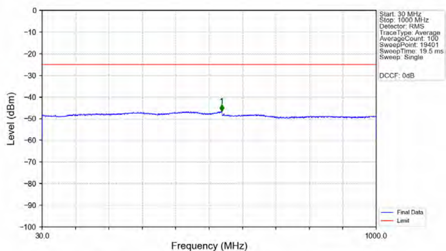
n7_15kHz_SISO_NTNV_5MHz_DFT-s-OFDM PI/2 BPSK_2535MHz_Edge_1RB_Left_Ant1
