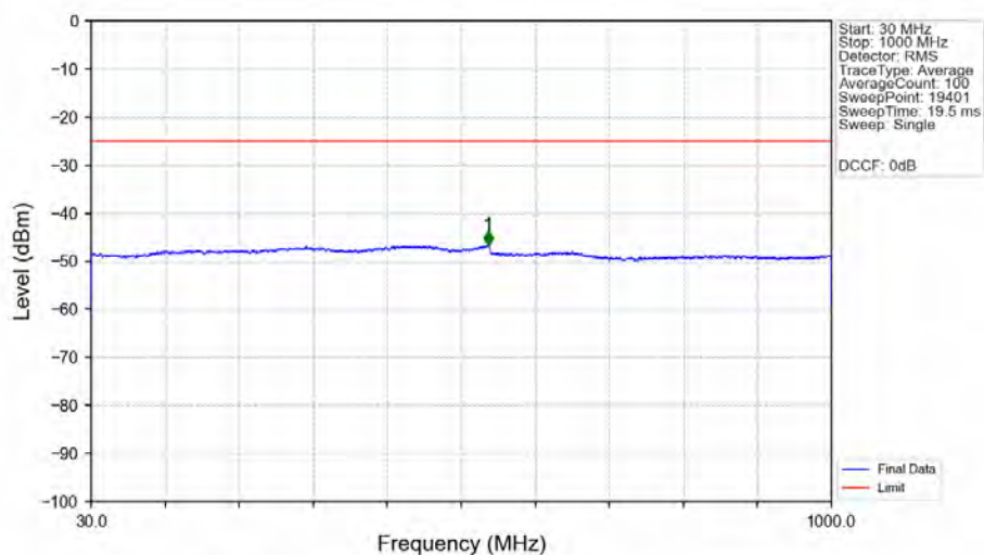
n7_15kHz_SISO_NTNV_25MHz_DFT-s-OFDM_PI/2_BPSK_2535MHz_Edge_1RB_Left_Ant1
