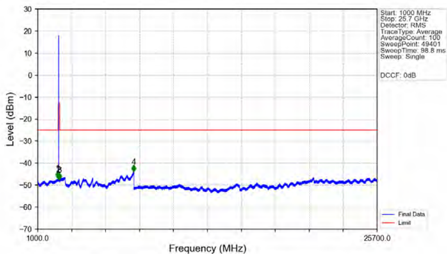
n7_15kHz_SISO_NTNV_25MHz_DFT-s-OFDM_PI/2_BPSK_2535MHz_Edge_1RB_Left_Ant1
