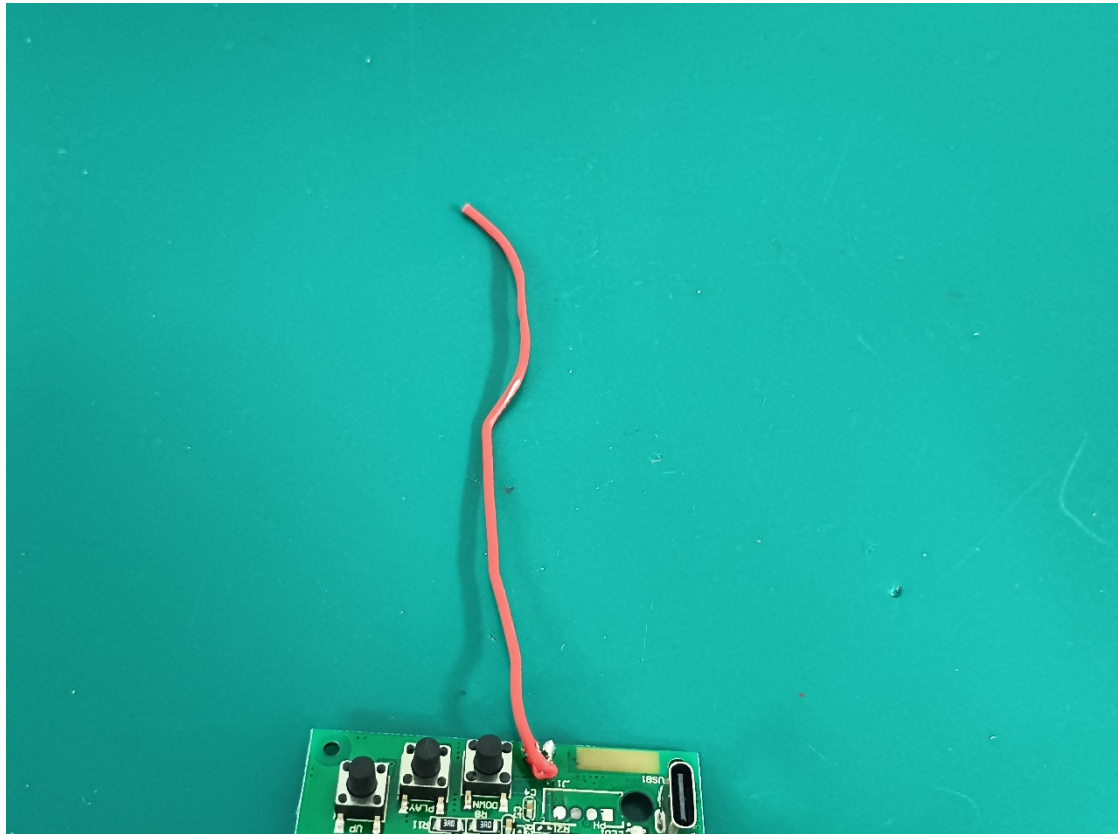
FM ANT
