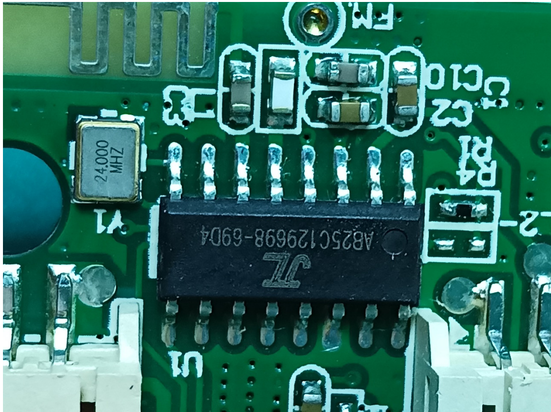
BT ANT
