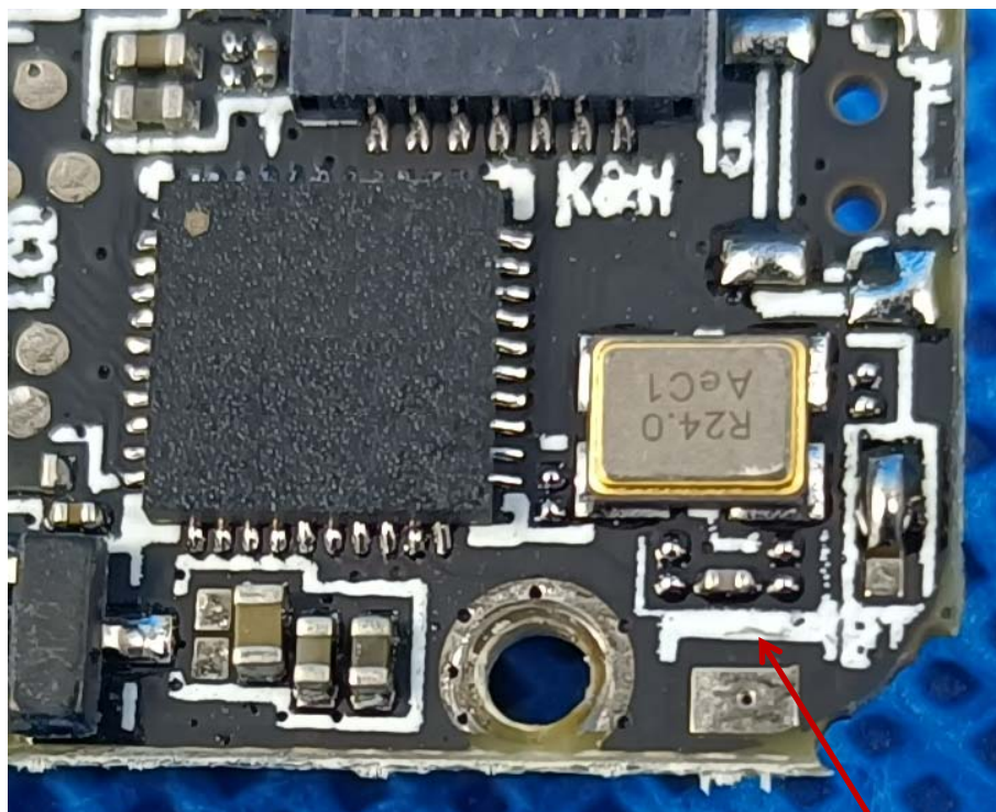
PCB ANT
