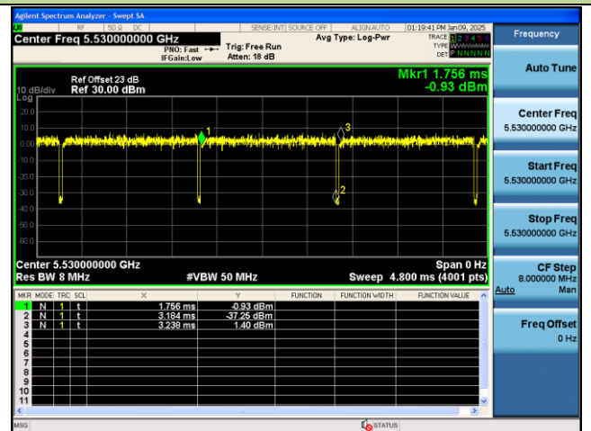
802.11ax-HE20
