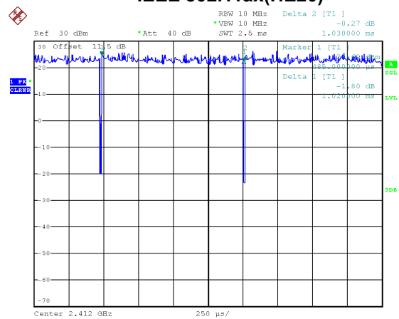
IEEE 802.11ax(HE20)
