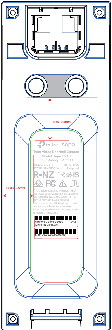
尺寸图
