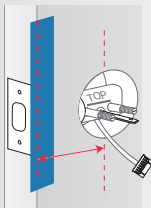
Backset 2-3/8" (60 mm)
