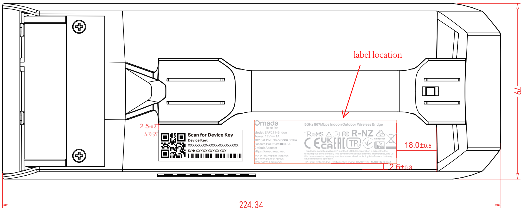
尺寸图
