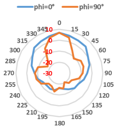
5250MHz_phi=0°&phi=90°
