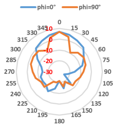
5750MHz_phi=0°&phi=90°
