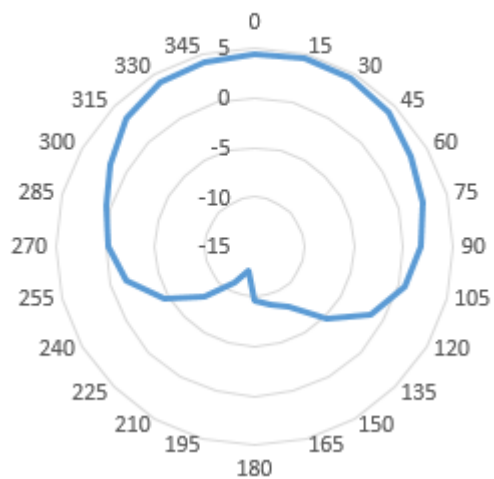
2450MHz Theta=90°
