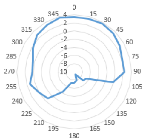
5250MHz Theta=90°
