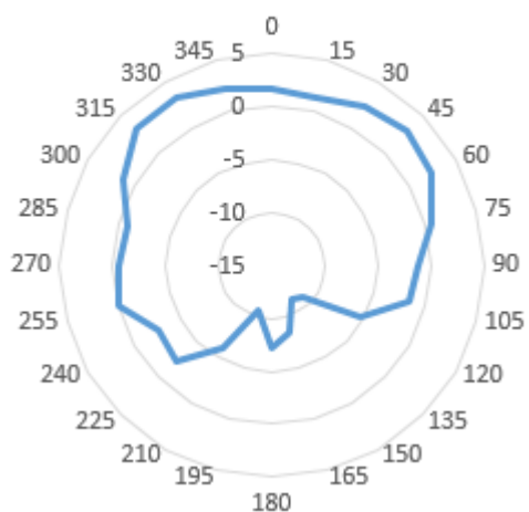
5750MHz Theta=90°
