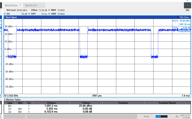
802.11ax(HE40)
