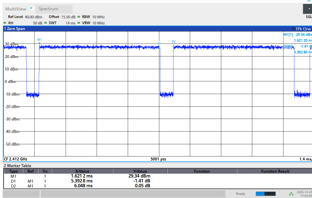
802.11ax(HE20)
