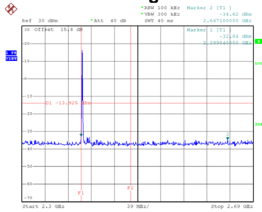
Bandedge-CH00
