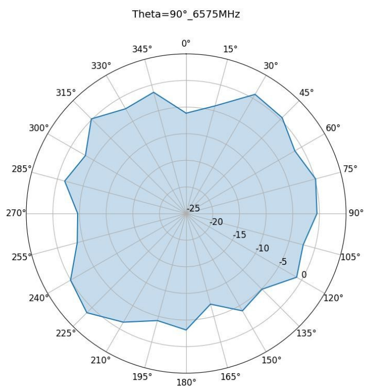
Ant1
