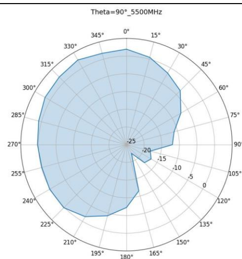
Ant4
