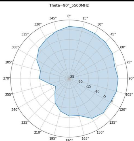
Ant4
