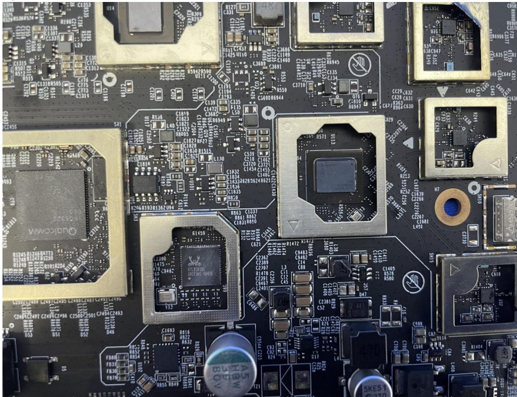
(20) EUT Photo
