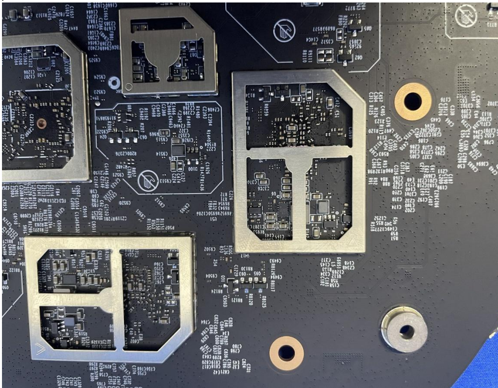
(12) EUT Photo
