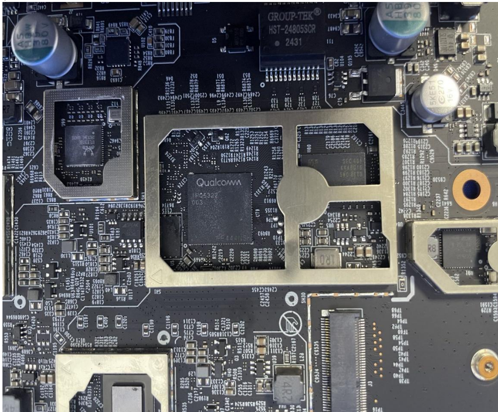
(18) EUT Photo
