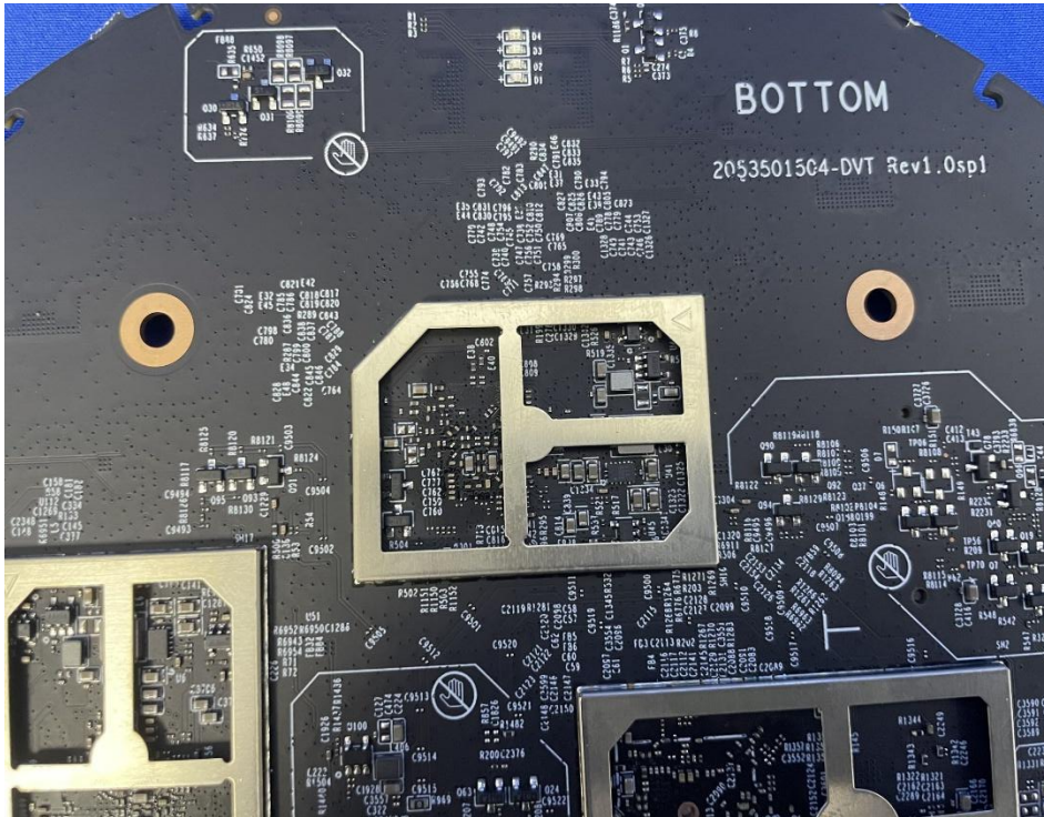
(10) EUT Photo
