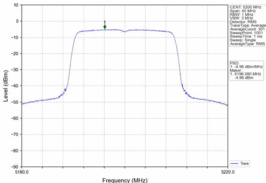
802.11ax(HE20)_MCH_5200MHz_RU242_Left_Ant2_NTNV
