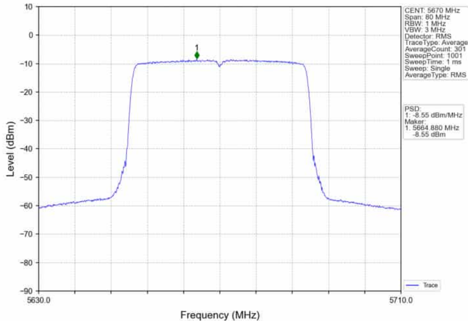
802.11ax(HE40)_HCH_5670MHz_RU484_Left_Ant1_NTNV
