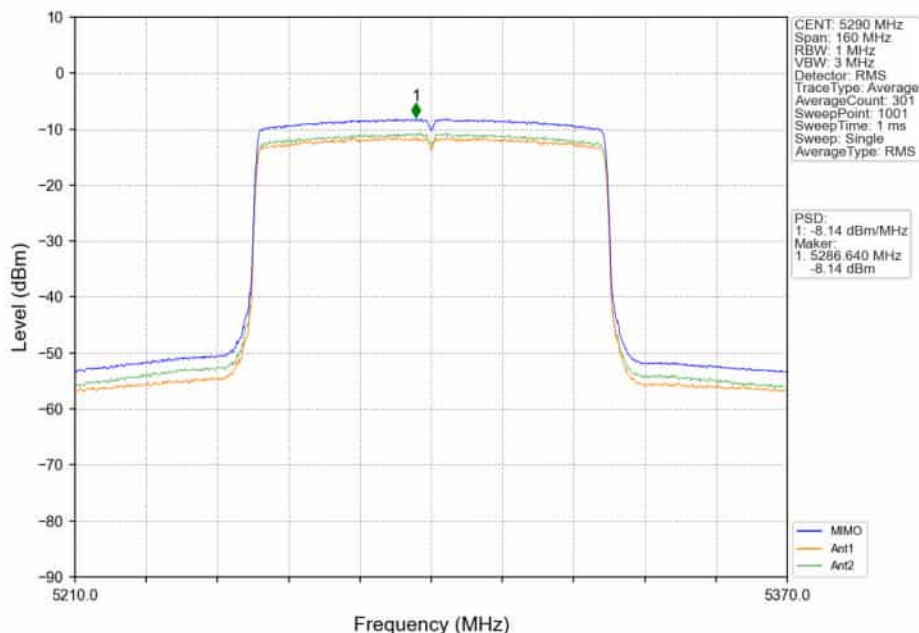
802.11ax(HE80)_MCH_5290MHz_RU996_Left_MIMO_NTNV
