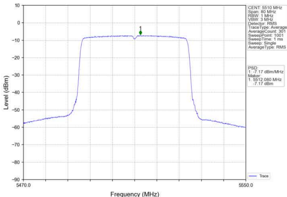
802.11ax(HE40)_LCH_5510MHz_RU484_Left_Ant2_NTNV
