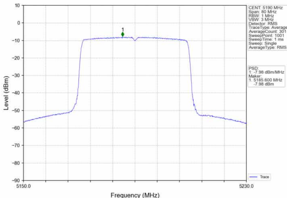
802.11ax(HE40)_LCH_5190MHz_RU484_Left_Ant2_NTNV
