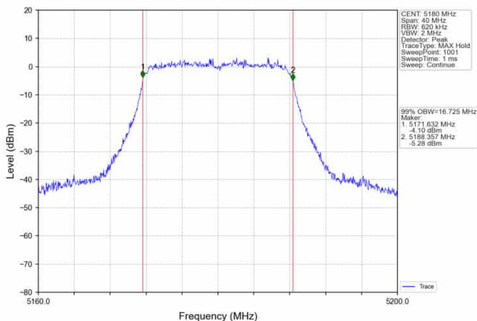
802.11a_LCH_5180MHz_Ant2_NTNV
