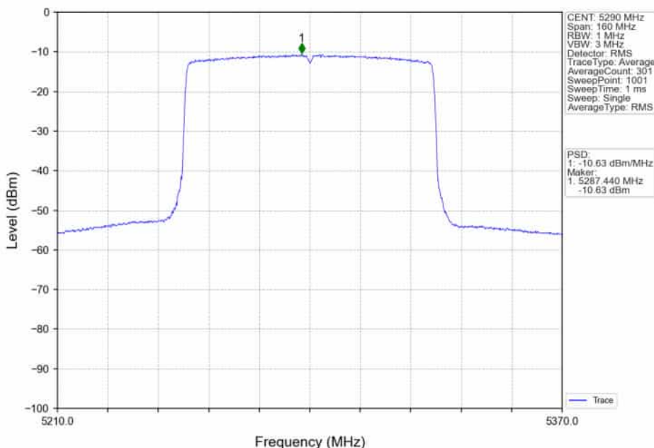
802.11ax(HE80)_MCH_5290MHz_RU996_Left_Ant2_NTNV
