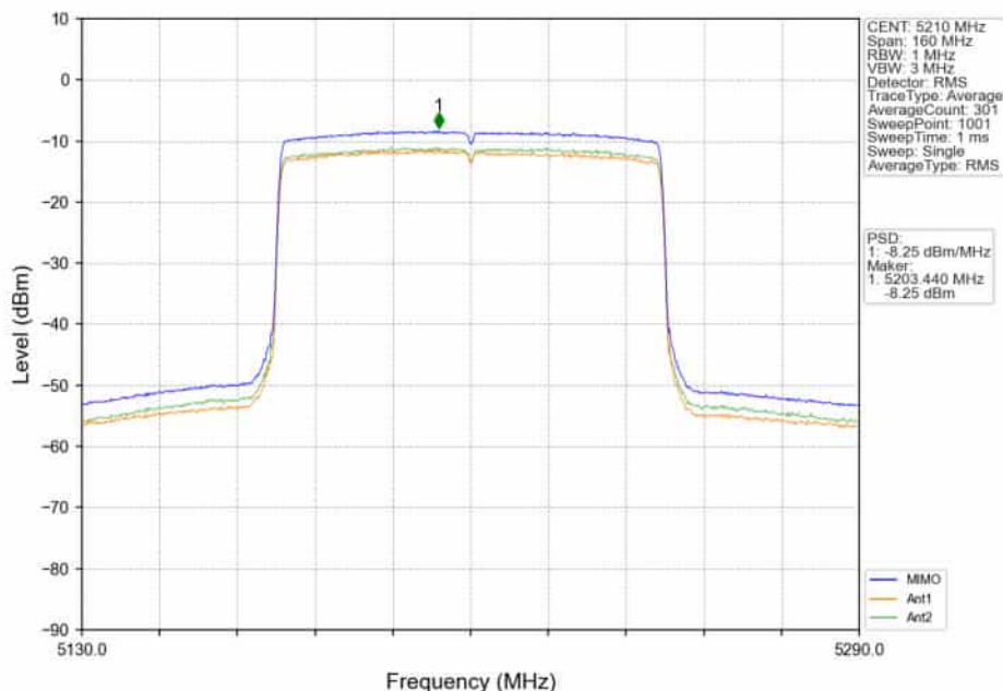
802.11ax(HE80)_MCH_5210MHz_RU996_Left_MIMO_NTNV
