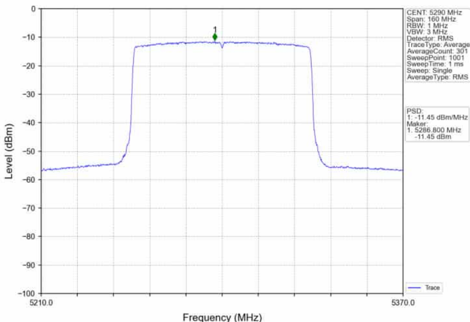
802.11ax(HE80)_MCH_5290MHz_RU996_Left_Ant1_NTNV
