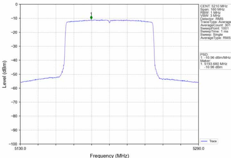
802.11ax(HE80)_MCH_5210MHz_RU996_Left_Ant2_NTNV
