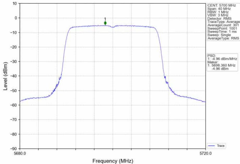
802.11ax(HE20)_HCH_5700MHz_RU242_Left_Ant2_NTNV
