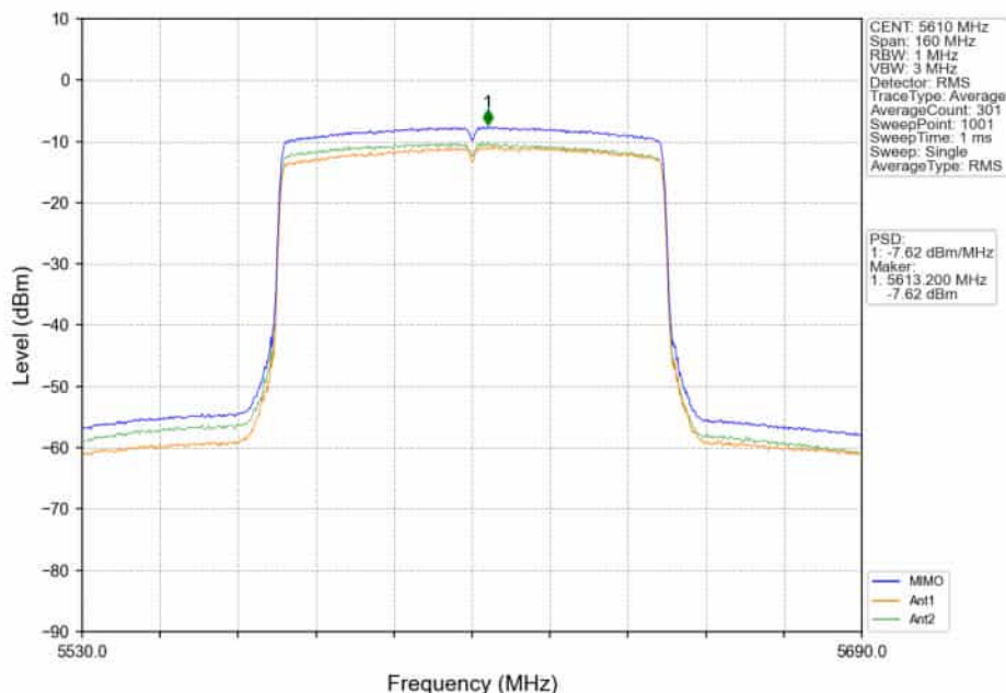
802.11ax(HE80)_HCH_5610MHz_RU996_Left_MIMO_NTNV
