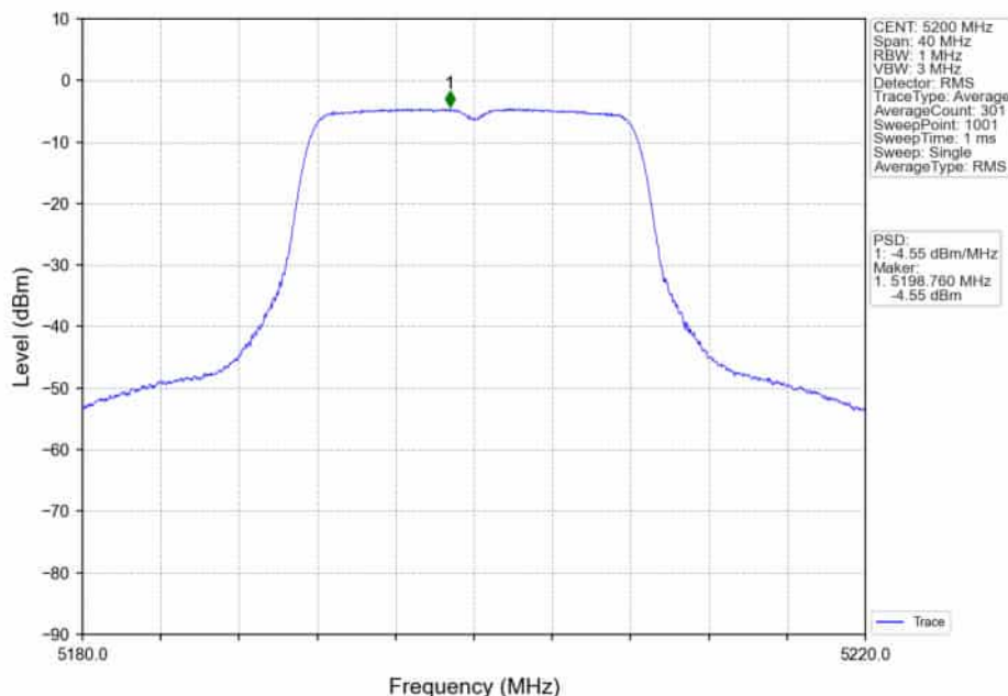
802.11a_MCH_5200MHz_Ant2_NTNV
