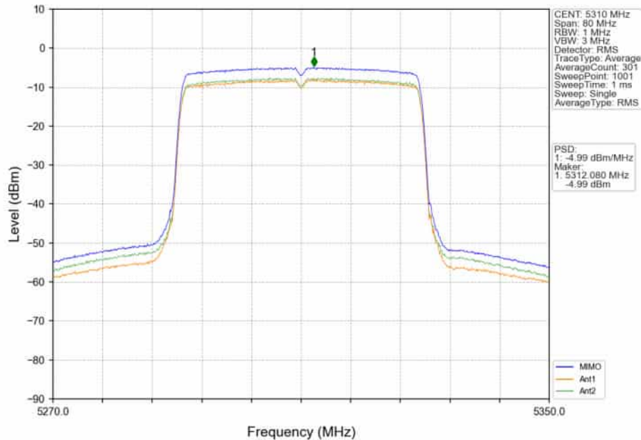
802.11ax(HE40)_HCH_5310MHz_RU484_Left_MIMO_NTNV
