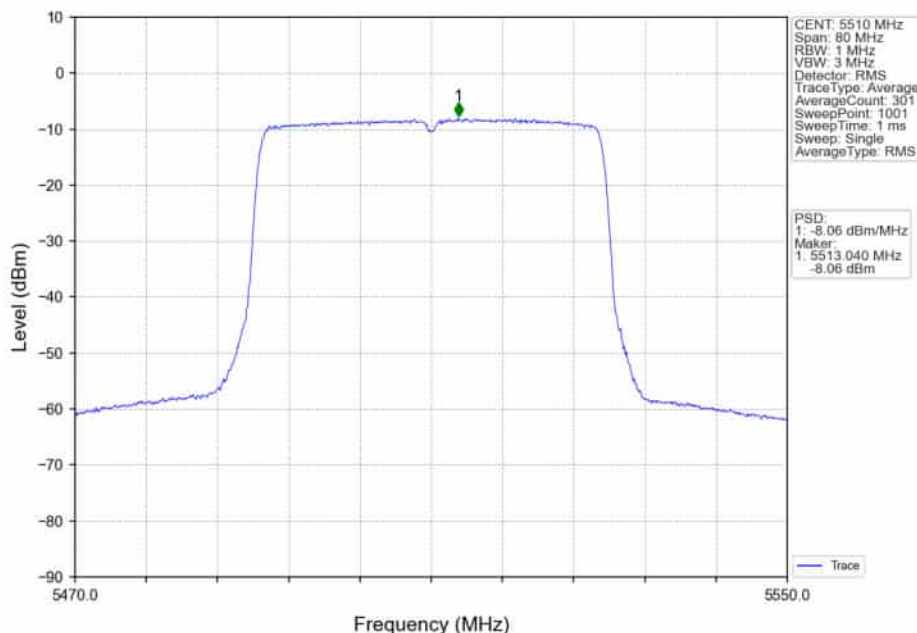
802.11ax(HE40)_LCH_5510MHz_RU484_Left_Ant1_NTNV
