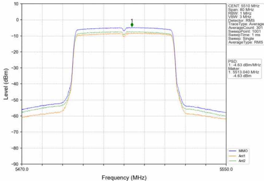
802.11ax(HE40)_LCH_5510MHz_RU484_Left_MIMO_NTNV
