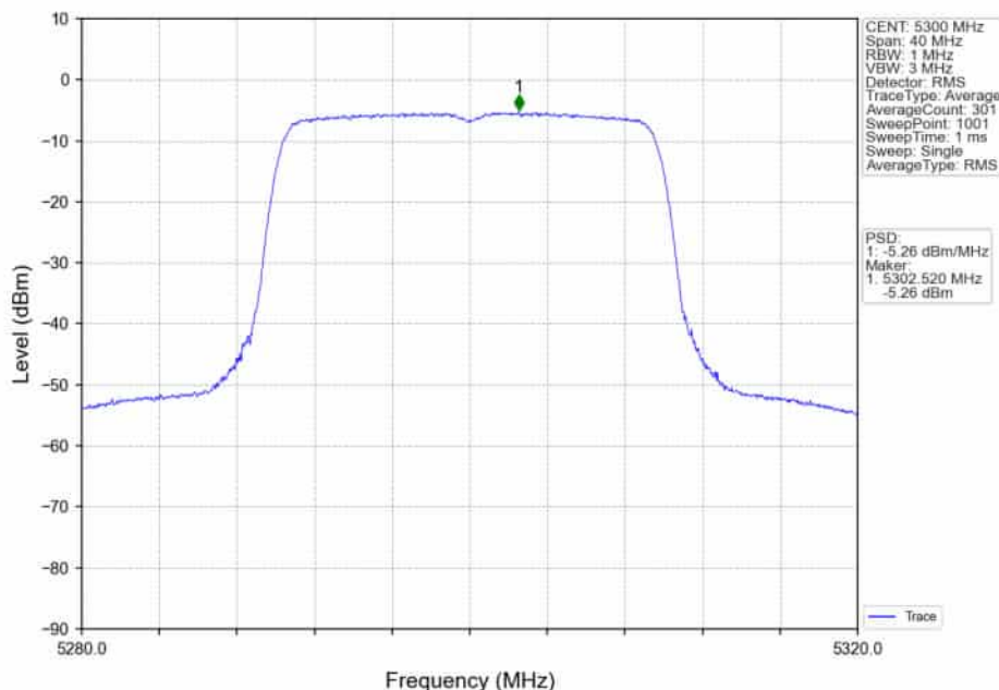
802.11ax(HE20)_MCH_5300MHz_RU242_Left_Ant1_NTNV
