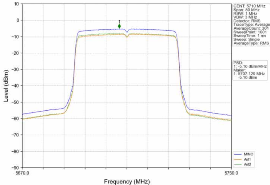
802.11ax(HE40)_HCH_5710MHz_RU484_Left_MIMO_NTNV
