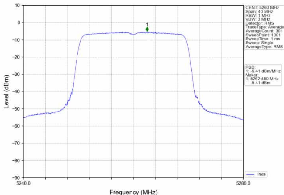
802.11ax(HE20)_LCH_5260MHz_RU242_Left_Ant1_NTNV
