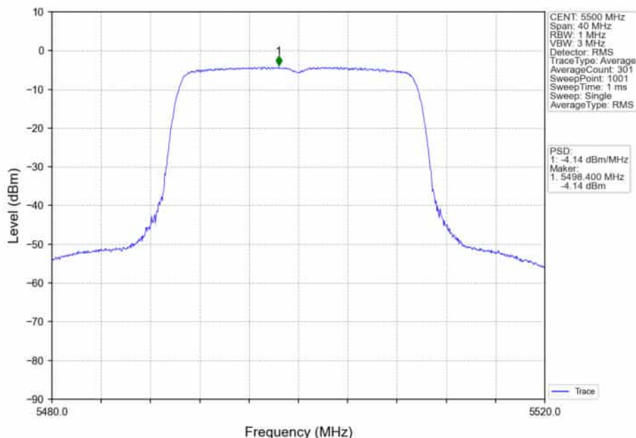
802.11ax(HE20)_LCH_5500MHz_RU242_Left_Ant2_NTNV
