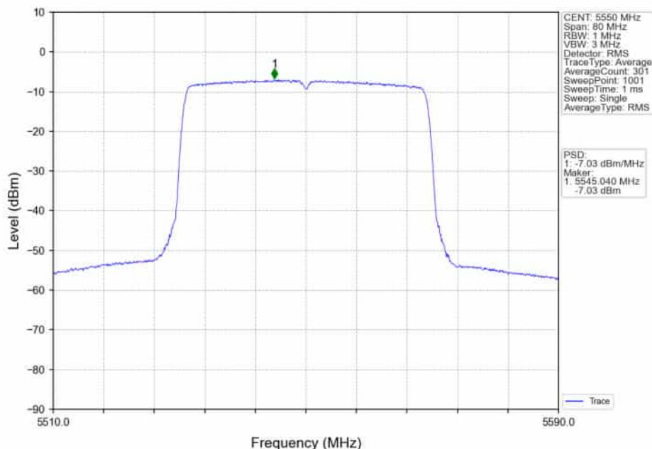
802.11ax(HE40)_MCH_5550MHz_RU484_Left_Ant2_NTNV
