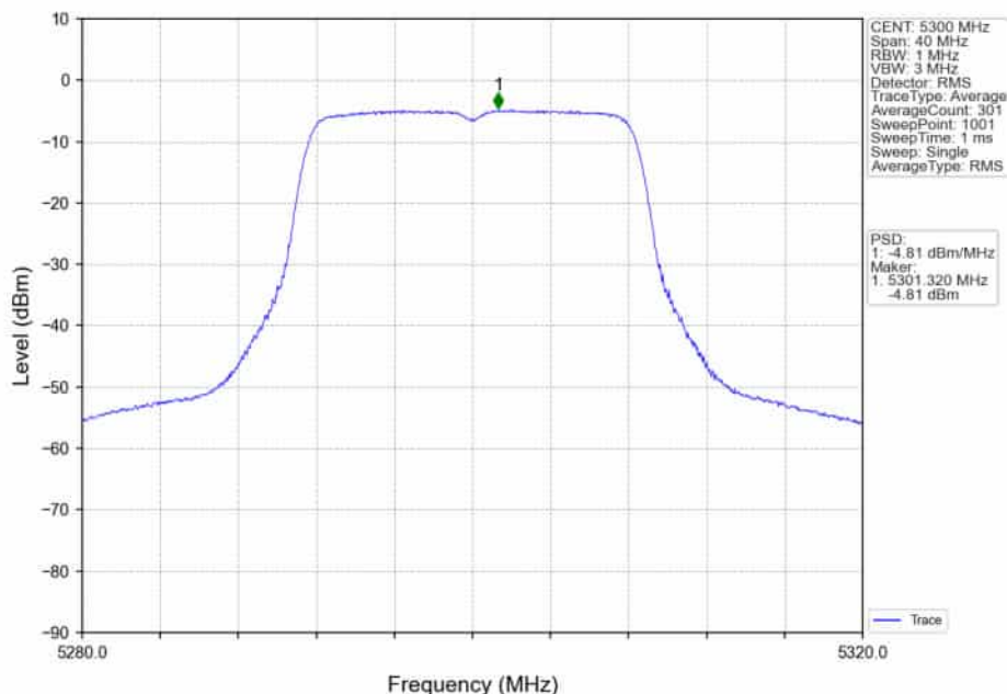
802.11a_MCH_5300MHz_Ant1_NTNV
