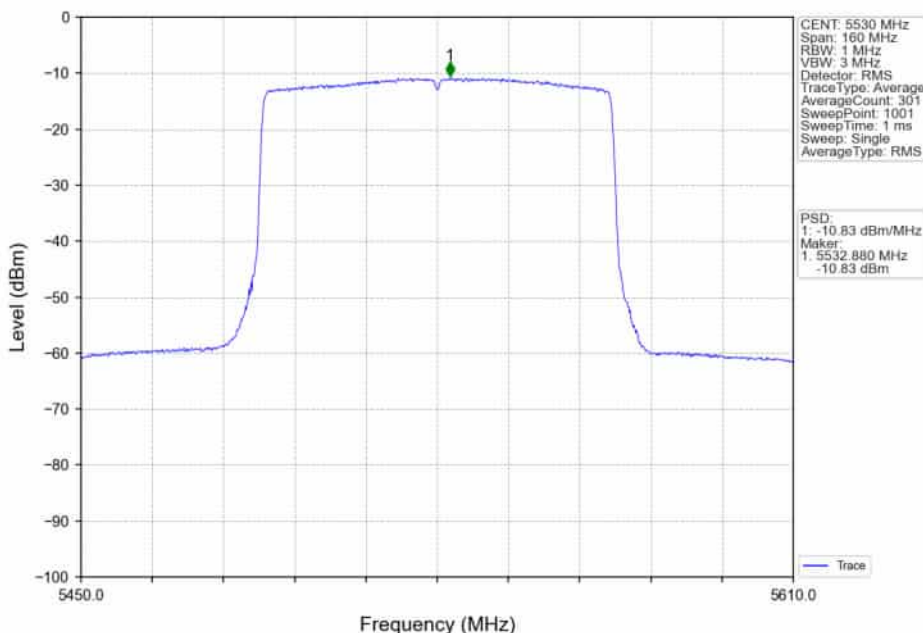
802.11ax(HE80)_LCH_5530MHz_RU996_Left_Ant1_NTNV
