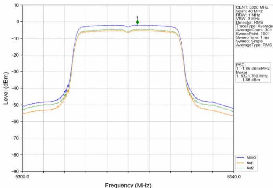
802.11ax(HE20)_HCH_5320MHz_RU242_Left_MIMO_NTNV
