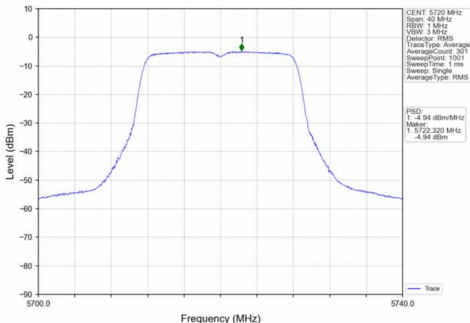
802.11a_HCH_5720MHz_Ant1_NTNV
