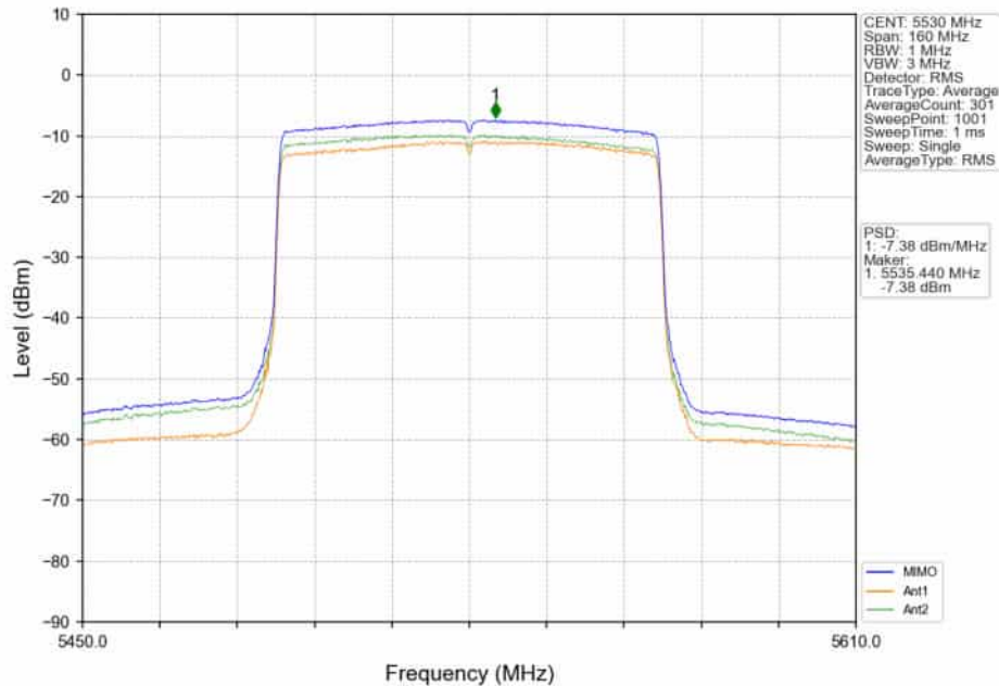
802.11ax(HE80)_LCH_5530MHz_RU996_Left_MIMO_NTNV
