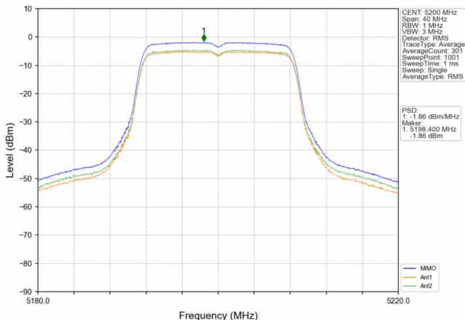
802.11a_MCH_5200MHz_MIMO_NTNV
