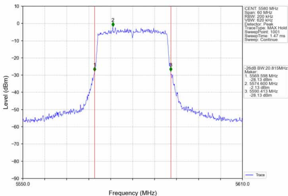
802.11ax(HE20)_MCH_5580MHz_RU242_Left_Ant1_NTNV
