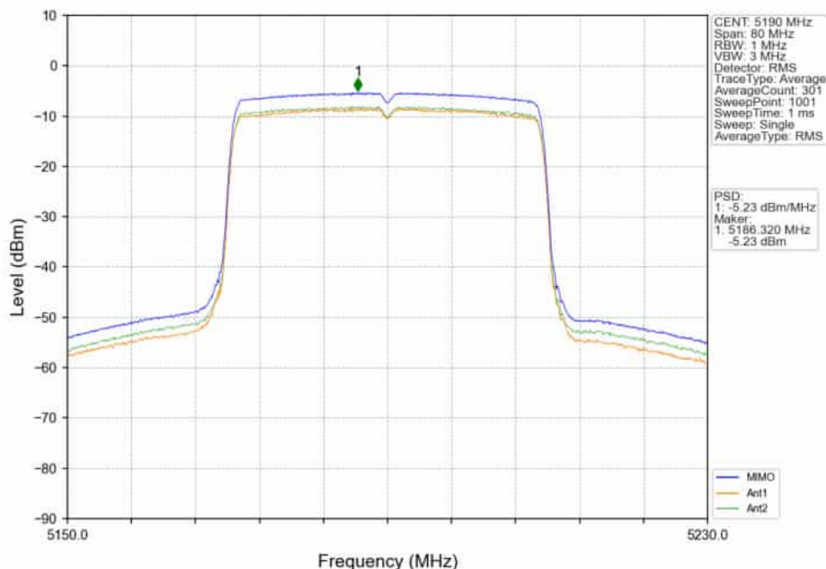
802.11ax(HE40)_LCH_5190MHz_RU484_Left_MIMO_NTNV
