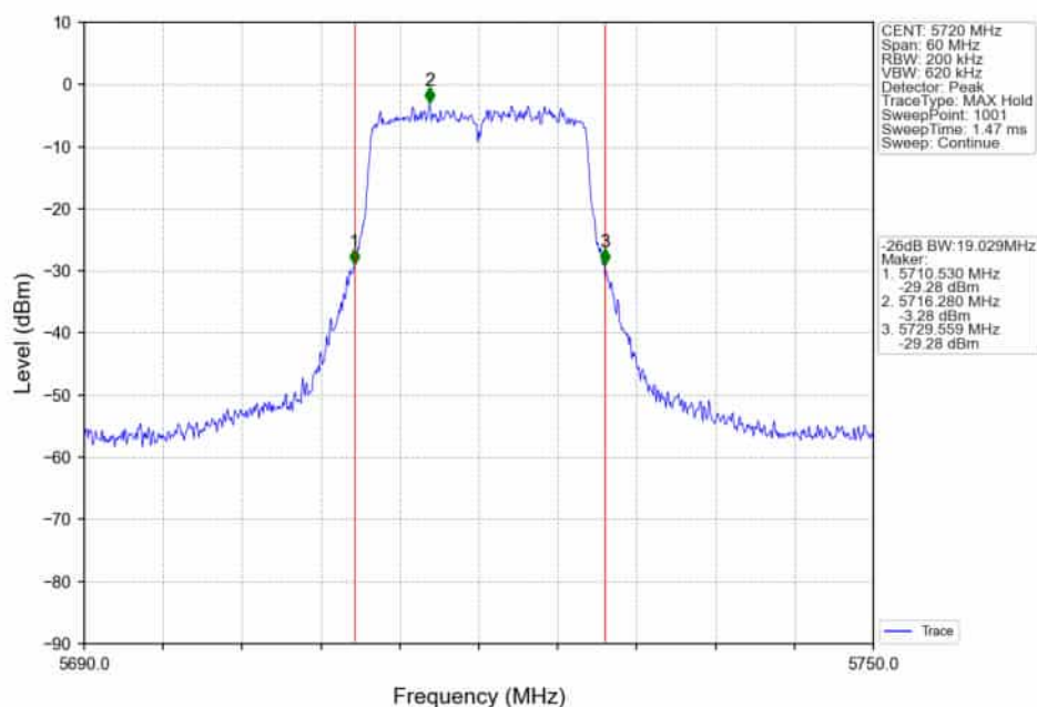
802.11a_HCH_5720MHz_Ant2_NTNV
