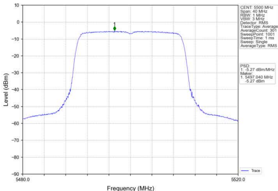
802.11ax(HE20)_LCH_5500MHz_RU242_Left_Ant1_NTNV
