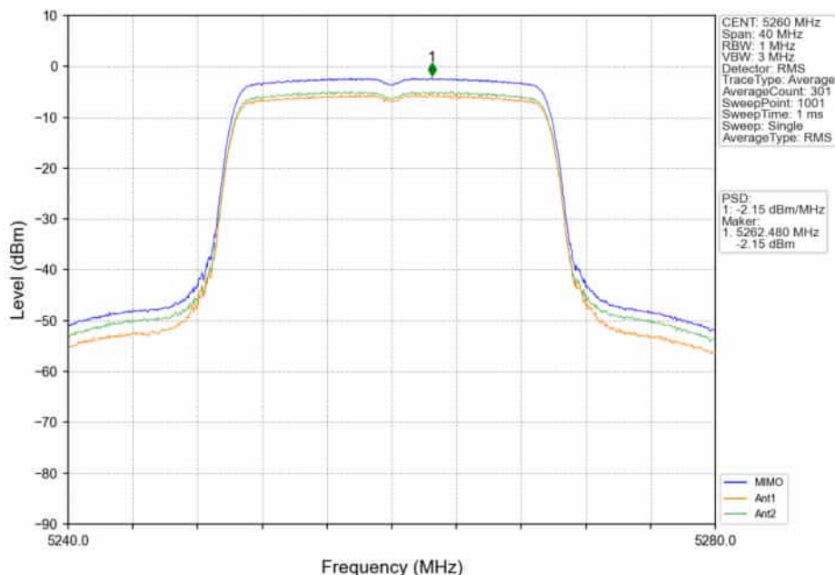
802.11ax(HE20)_LCH_5260MHz_RU242_Left_MIMO_NTNV
