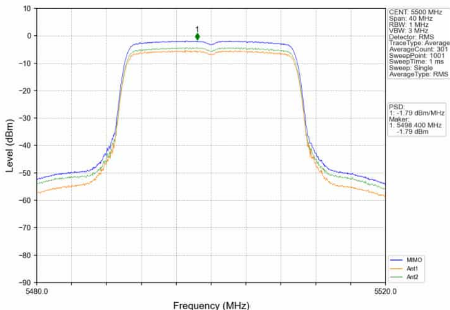
802.11ax(HE20)_LCH_5500MHz_RU242_Left_MIMO_NTNV
