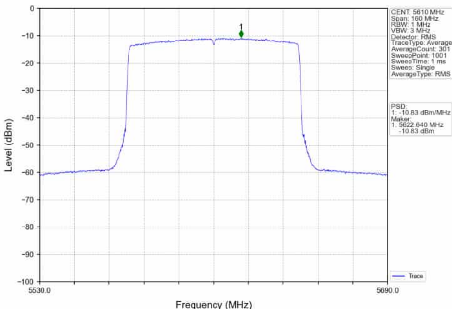
802.11ax(HE80)_HCH_5610MHz_RU996_Left_Ant1_NTNV
