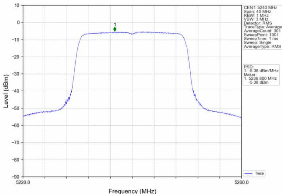
802.11ax(HE20)_HCH_5240MHz_RU242_Left_Ant1_NTNV
