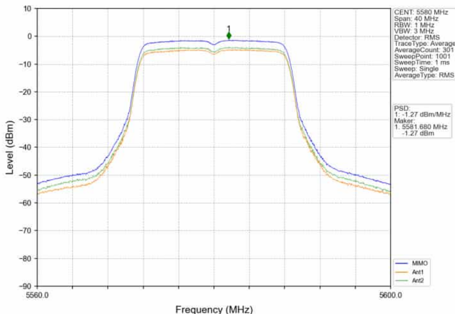
802.11a_MCH_5580MHz_MIMO_NTNV
