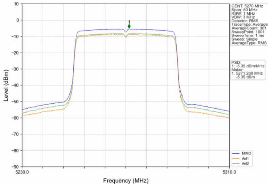
802.11ax(HE40)_LCH_5270MHz_RU484_Left_MIMO_NTNV
