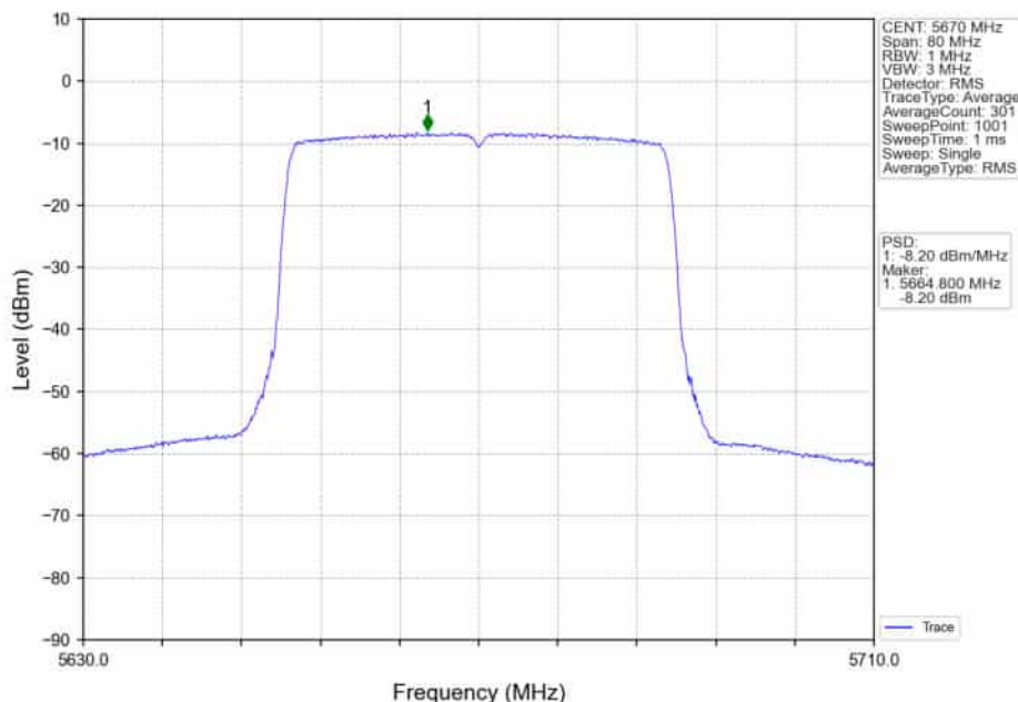
802.11ax(HE40)_HCH_5670MHz_RU484_Left_Ant2_NTNV
