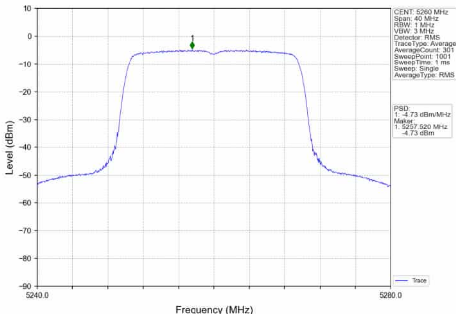
802.11ax(HE20)_LCH_5260MHz_RU242_Left_Ant2_NTNV
