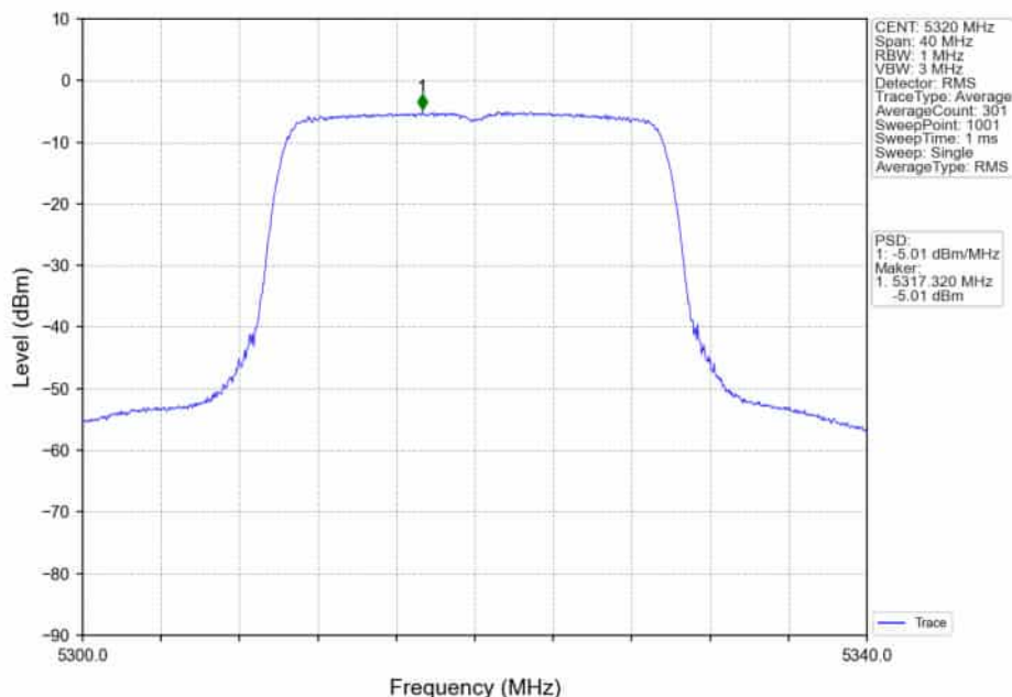
802.11ax(HE20)_HCH_5320MHz_RU242_Left_Ant1_NTNV
