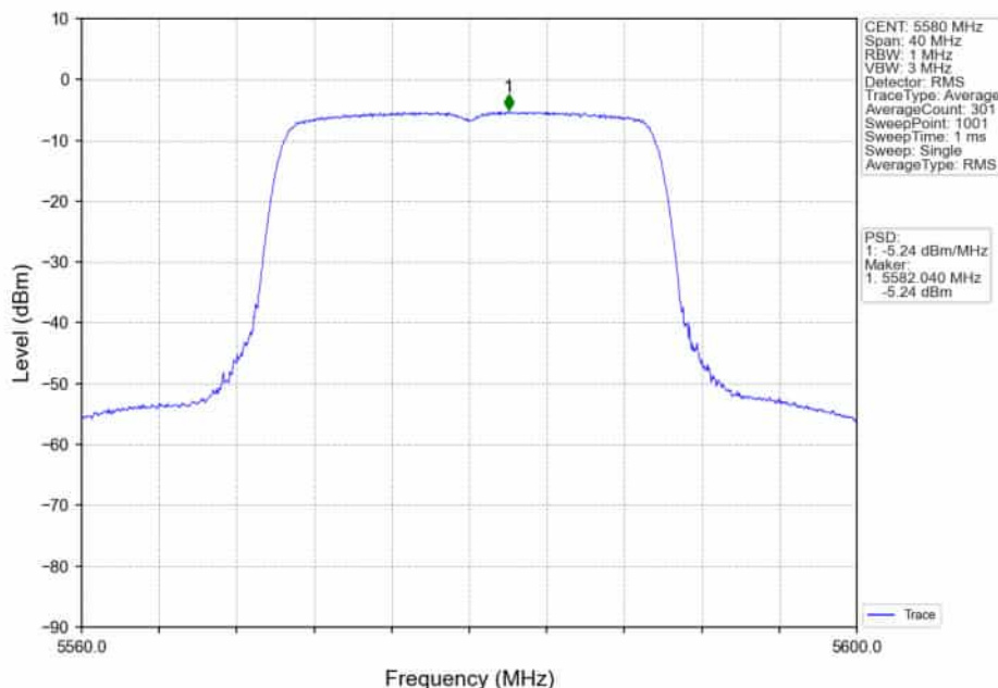
802.11ax(HE20)_MCH_5580MHz_RU242_Left_Ant1_NTNV
