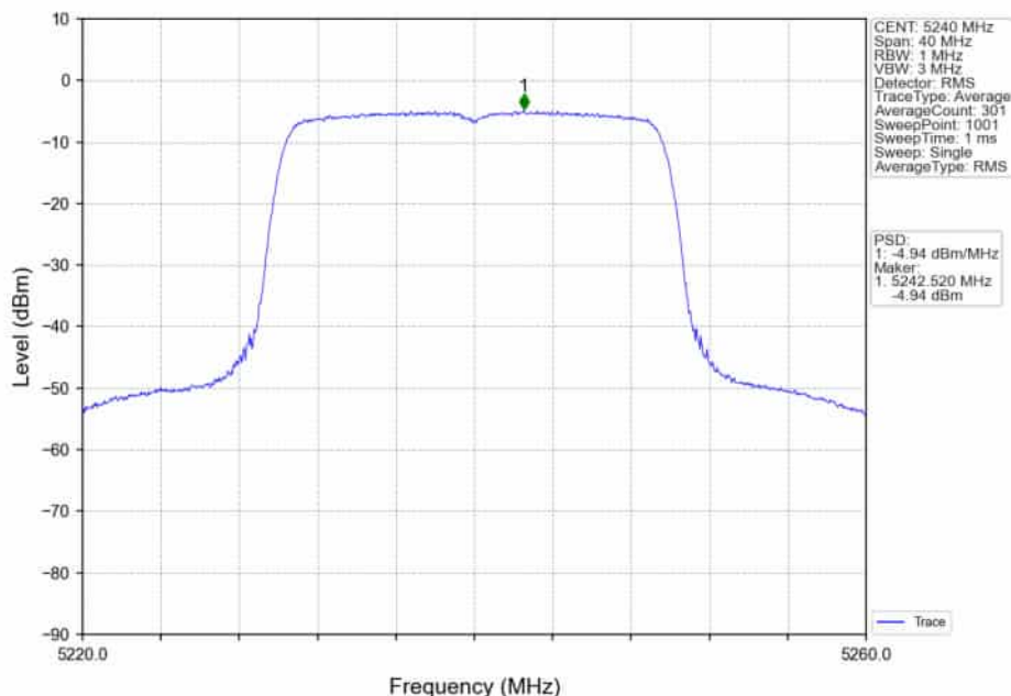
802.11ax(HE20)_HCH_5240MHz_RU242_Left_Ant2_NTNV
