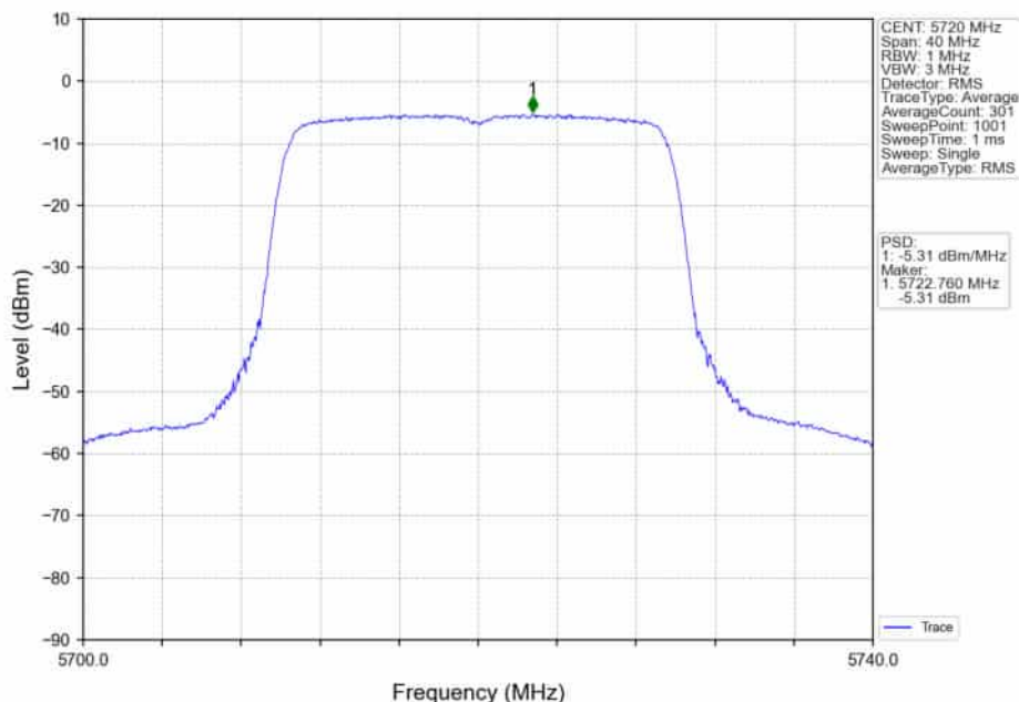
802.11ax(HE20)_HCH_5720MHz_RU242_Left_Ant1_NTNV
