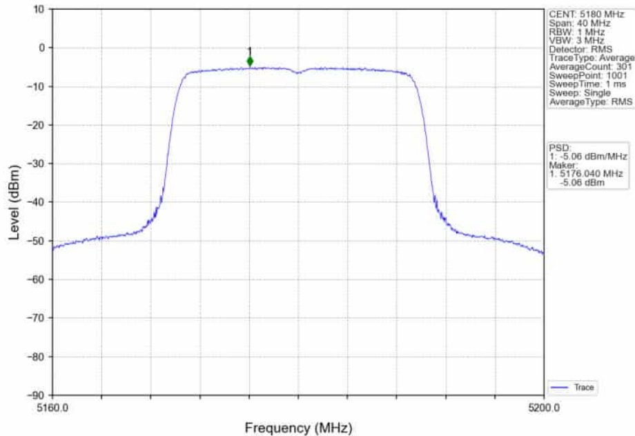
802.11ax(HE20)_LCH_5180MHz_RU242_Left_Ant2_NTNV
