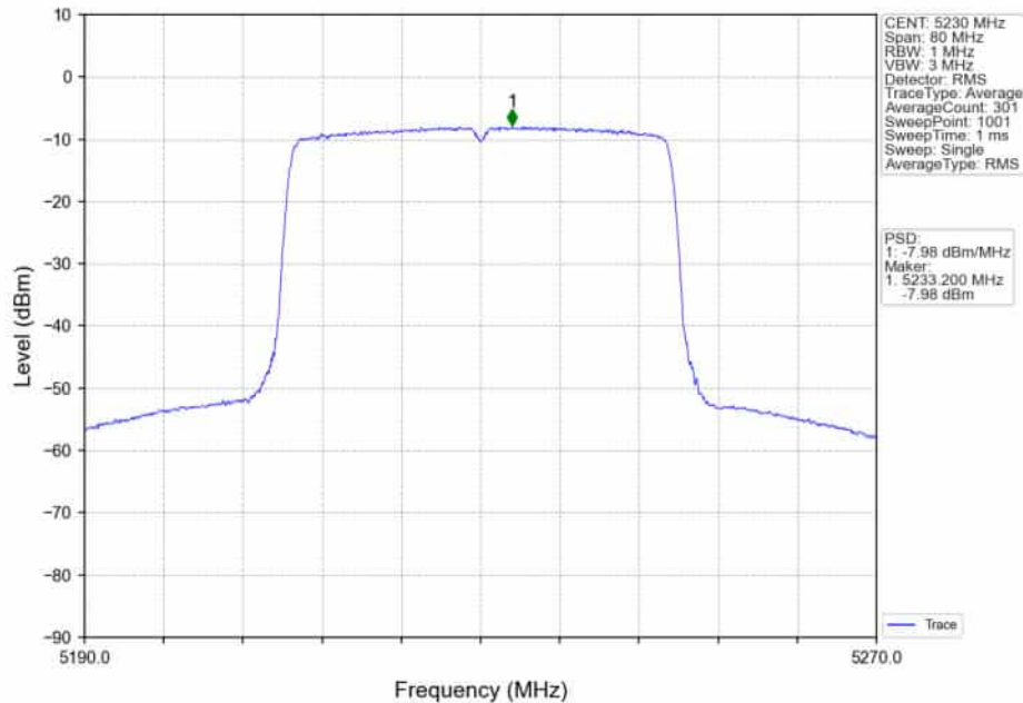
802.11ax(HE40)_HCH_5230MHz_RU484_Left_Ant2_NTNV
