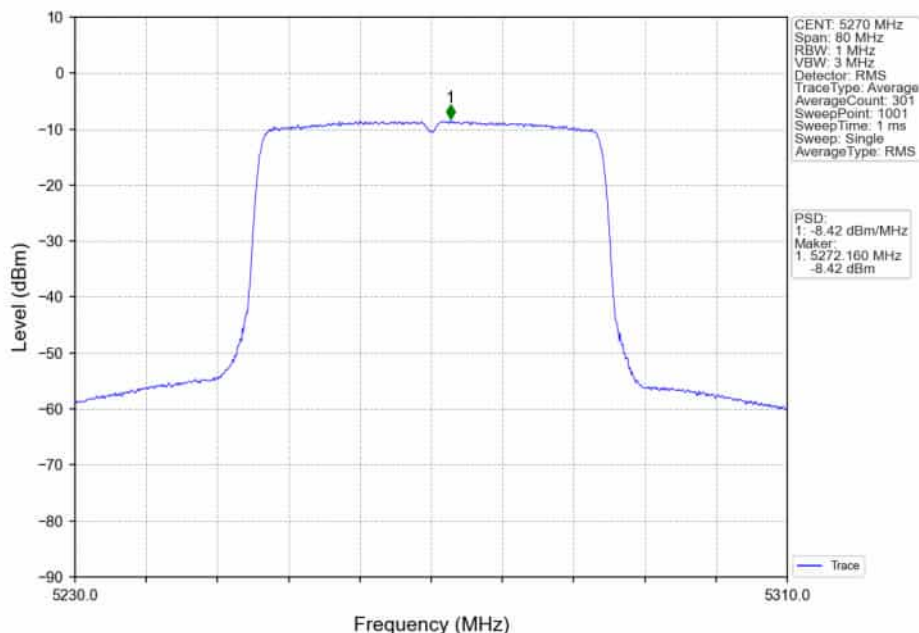
802.11ax(HE40)_LCH_5270MHz_RU484_Left_Ant1_NTNV
