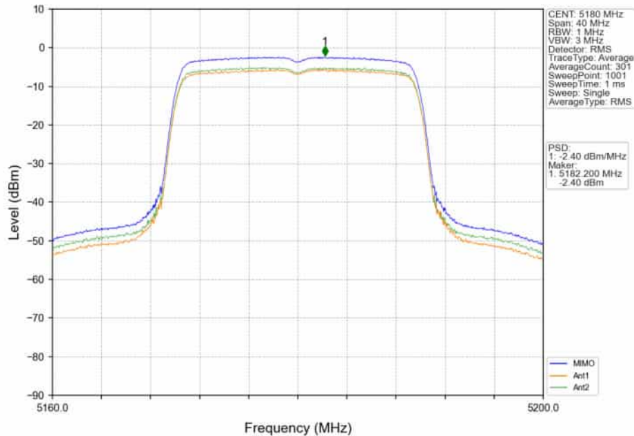
802.11ax(HE20)_LCH_5180MHz_RU242_Left_MIMO_NTNV
