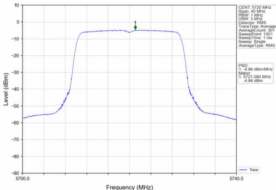
802.11ax(HE20)_HCH_5720MHz_RU242_Left_Ant2_NTNV
