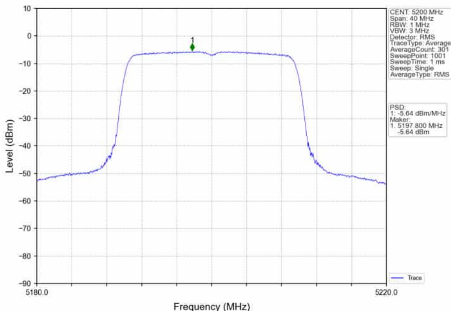
802.11ax(HE20)_MCH_5200MHz_RU242_Left_Ant1_NTNV
