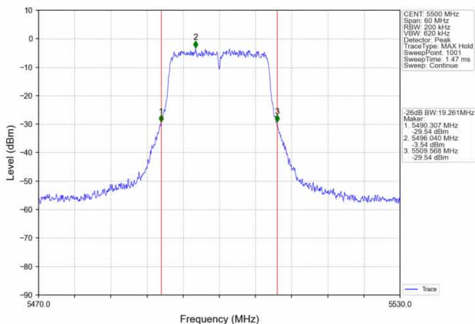
802.11a_LCH_5500MHz_Ant1_NTNV
