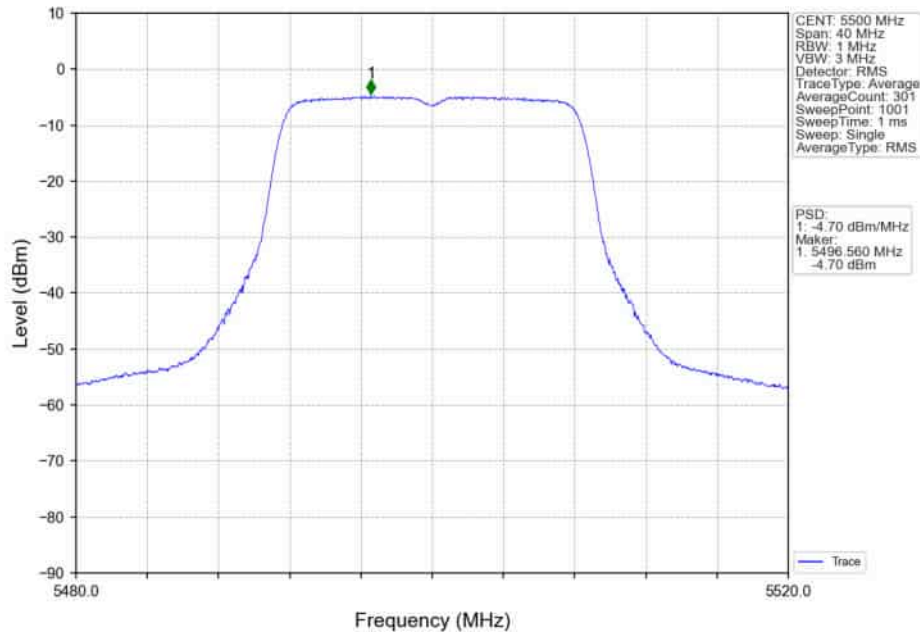
802.11a_LCH_5500MHz_Ant1_NTNV
