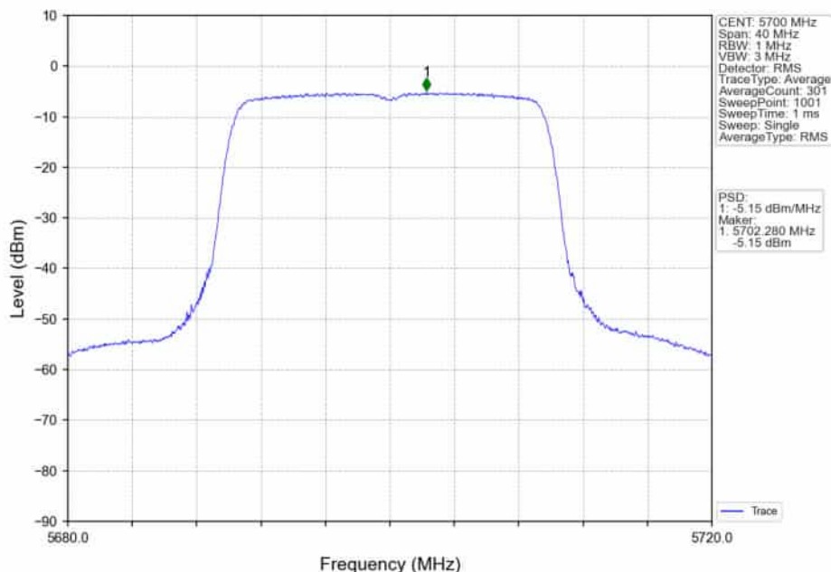
802.11ax(HE20)_HCH_5700MHz_RU242_Left_Ant1_NTNV
