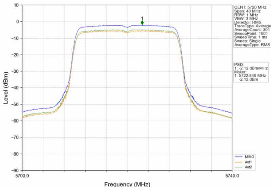
802.11ax(HE20)_HCH_5720MHz_RU242_Left_MIMO_NTNV
