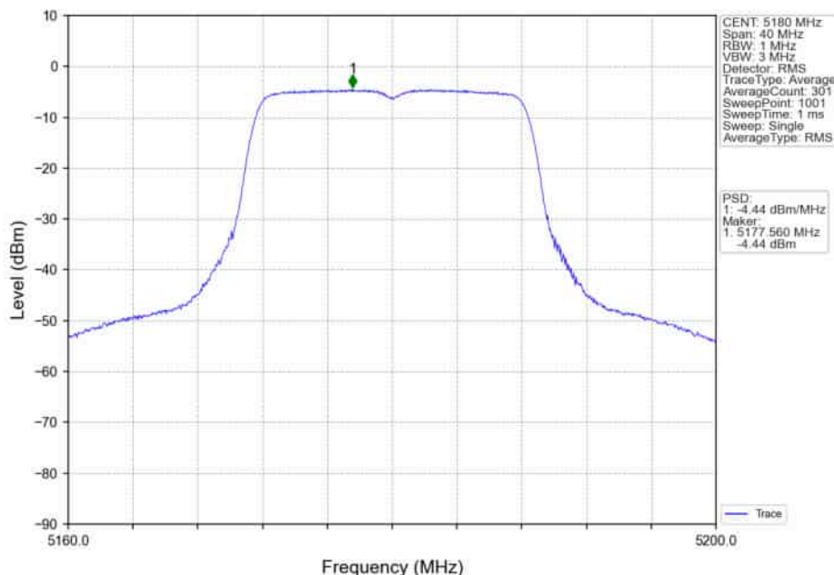
802.11a_LCH_5180MHz_Ant2_NTNV
