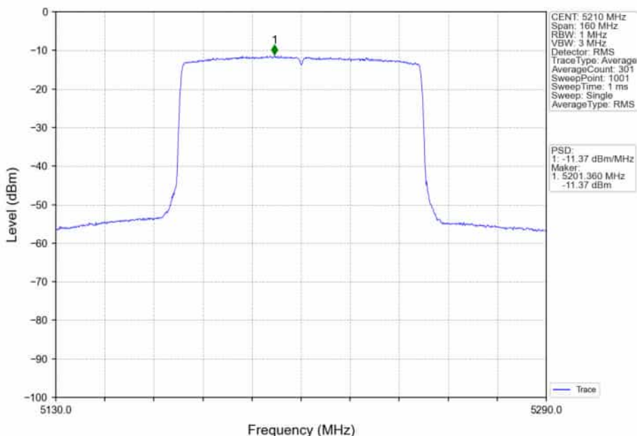
802.11ax(HE80)_MCH_5210MHz_RU996_Left_Ant1_NTNV
