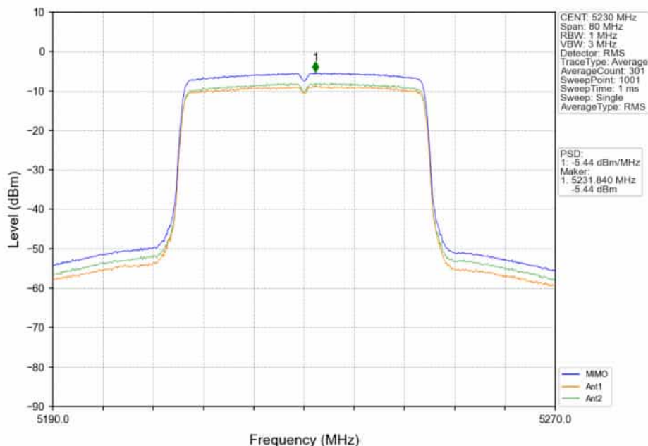
802.11ax(HE40)_HCH_5230MHz_RU484_Left_MIMO_NTNV
