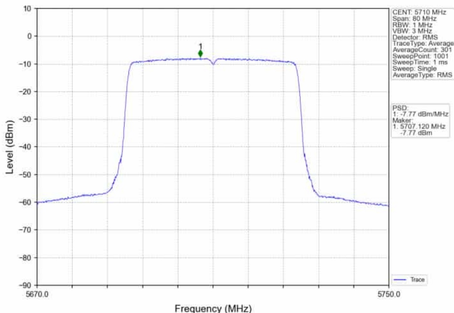
802.11ax(HE40)_HCH_5710MHz_RU484_Left_Ant2_NTNV
