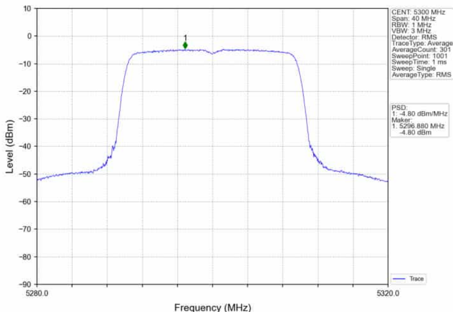
802.11ax(HE20)_MCH_5300MHz_RU242_Left_Ant2_NTNV
