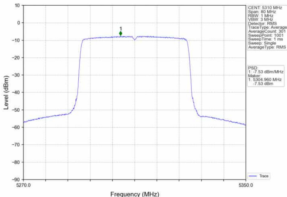
802.11ax(HE40)_HCH_5310MHz_RU484_Left_Ant2_NTNV
