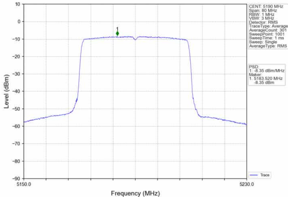
802.11ax(HE40)_LCH_5190MHz_RU484_Left_Ant1_NTNV
