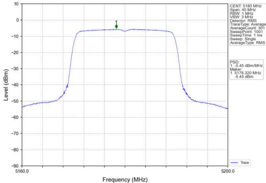
802.11ax(HE20)_LCH_5180MHz_RU242_Left_Ant1_NTNV
