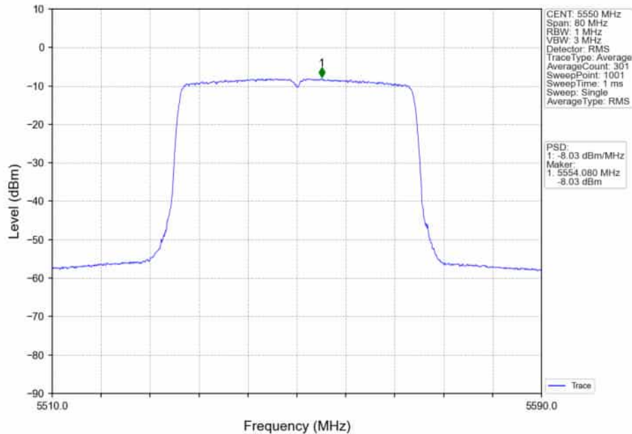
802.11ax(HE40)_MCH_5550MHz_RU484_Left_Ant1_NTNV
