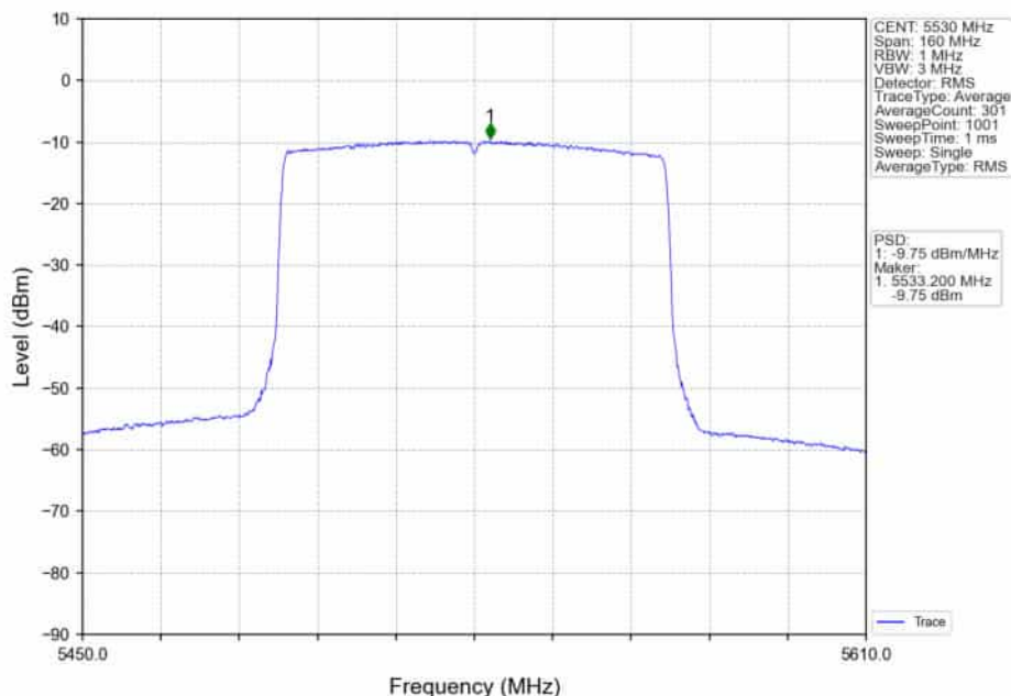
802.11ax(HE80)_LCH_5530MHz_RU996_Left_Ant2_NTNV
