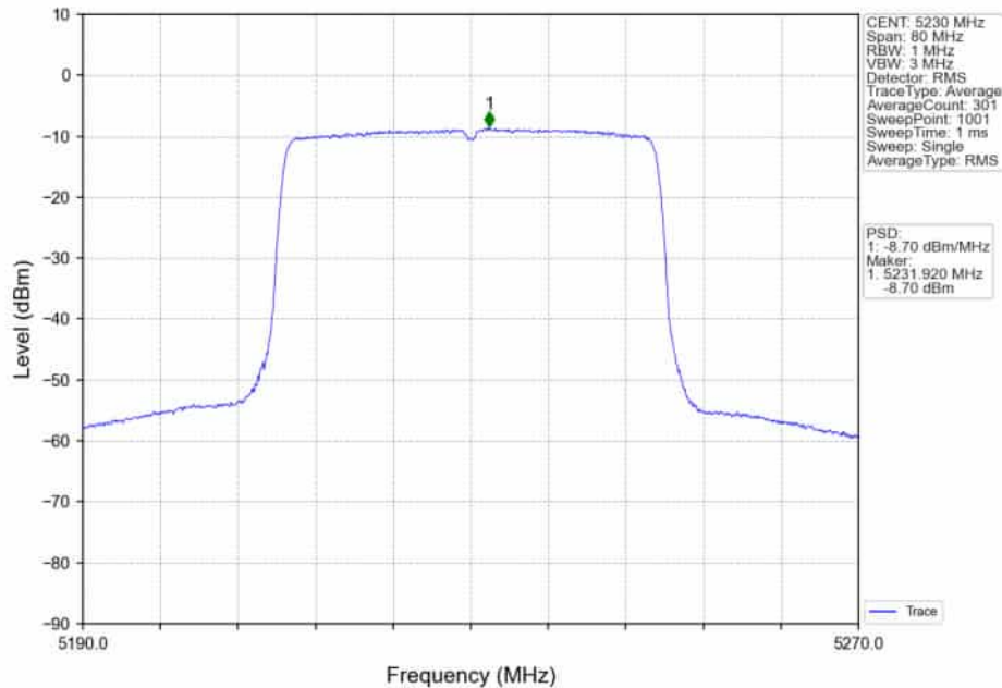
802.11ax(HE40)_HCH_5230MHz_RU484_Left_Ant1_NTNV
