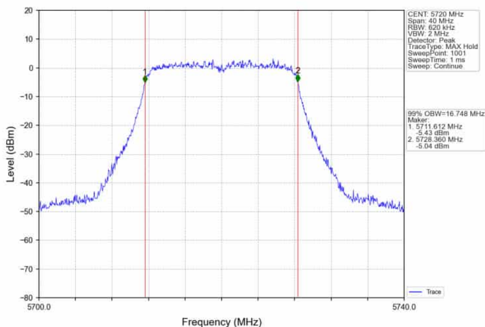
802.11a_HCH_5720MHz_Ant2_NTNV
