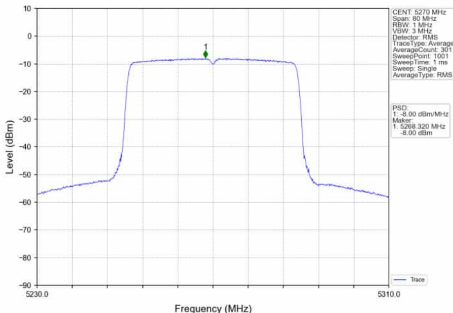
802.11ax(HE40)_LCH_5270MHz_RU484_Left_Ant2_NTNV
