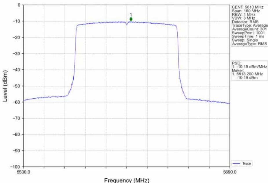
802.11ax(HE80)_HCH_5610MHz_RU996_Left_Ant2_NTNV
