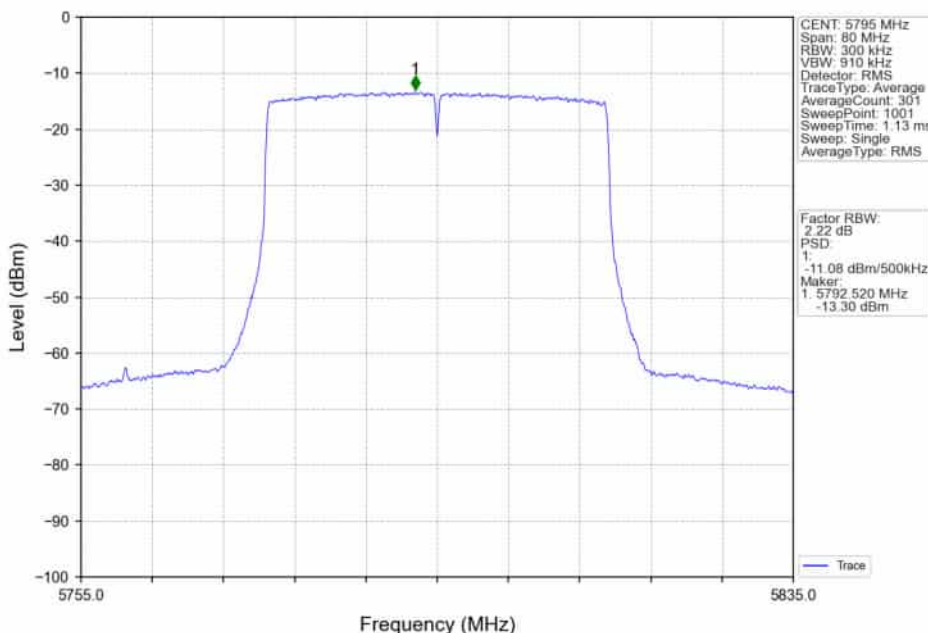
802.11ax(HE40)_HCH_5795MHz_RU484_Left_Ant2_NTNV
