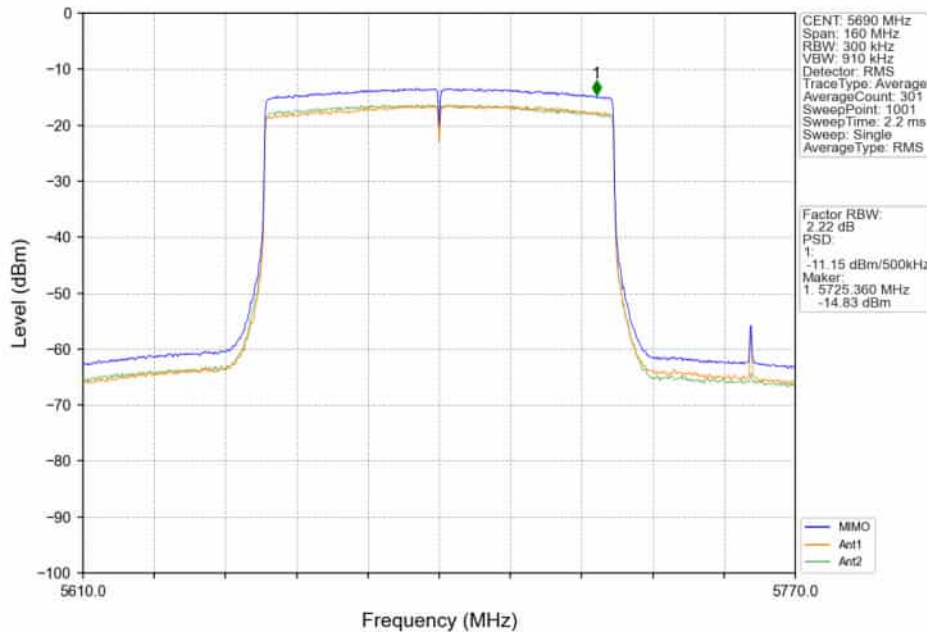
802.11ax(HE80)_HCH_5690MHz_RU996_Left_MIMO_NTNV
