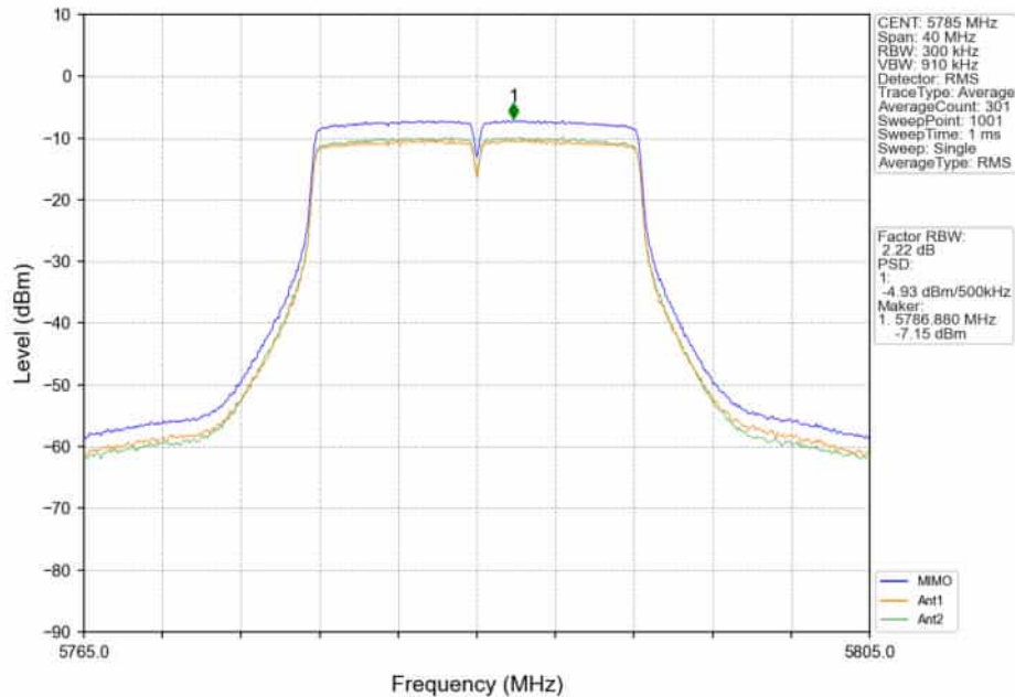
802.11a_MCH_5785MHz_MIMO_NTNV
