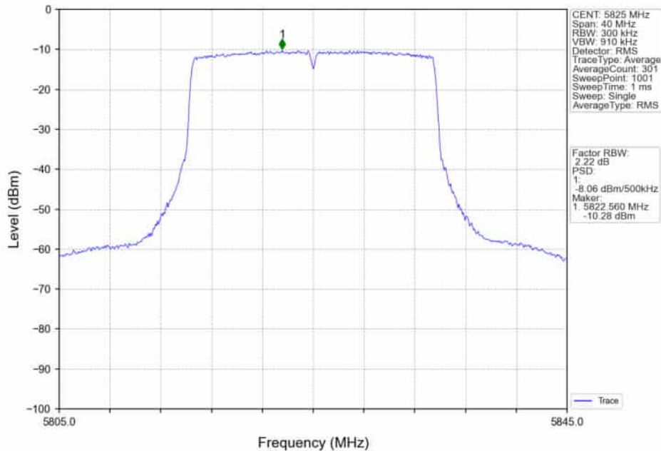
802.11ax(HE20)_HCH_5825MHz_RU242_Left_Ant2_NTNV
