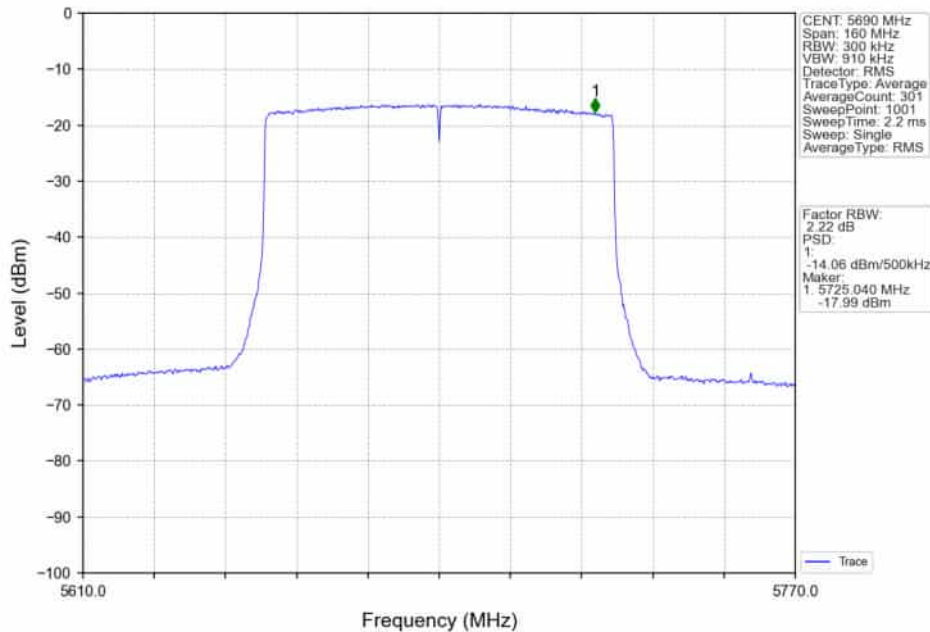
802.11ax(HE80)_HCH_5690MHz_RU996_Left_Ant2_NTNV
