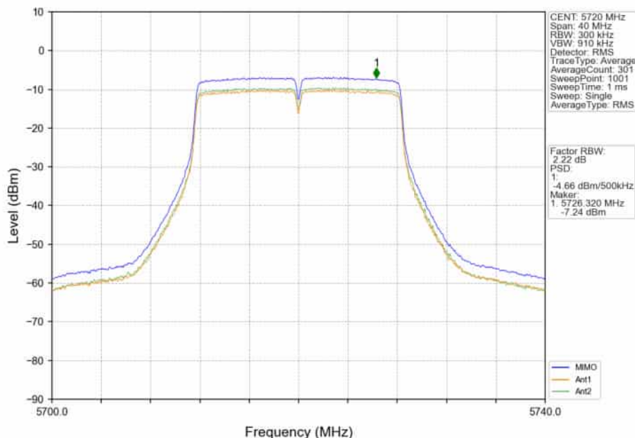
802.11a_HCH_5720MHz_MIMO_NTNV
