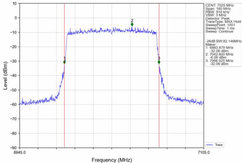
802.11ax(HEW80)_HCH_7025MHz_RU996_Left_Ant2_NTNV
