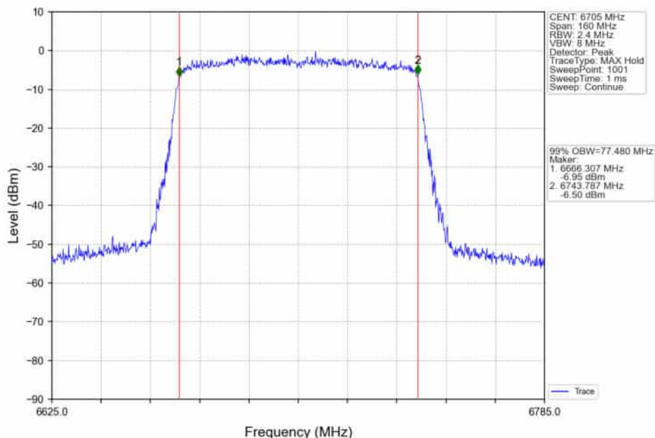
802.11ax(HEW80)_MCH_6705MHz_RU996_Left_Ant2_NTNV
