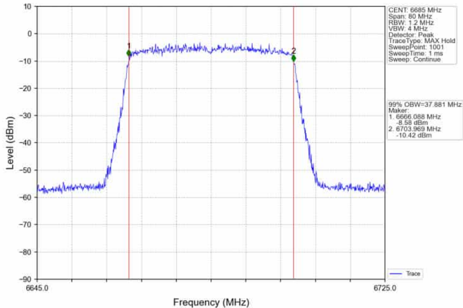
802.11ax(HEW40)_MCH_6685MHz_RU484_Left_Ant2_NTNV
