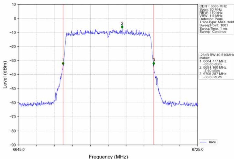
802.11ax(HEW40)_MCH_6685MHz_RU484_Left_Ant2_NTNV
