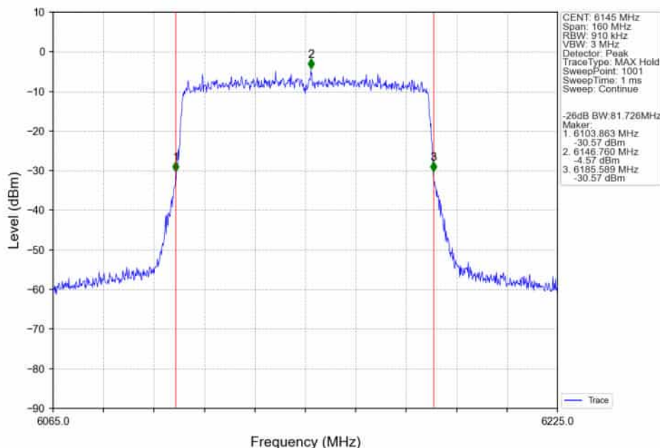
802.11ax(HEW80)_LCH_6145MHz_RU996_Left_Ant2_NTNV
