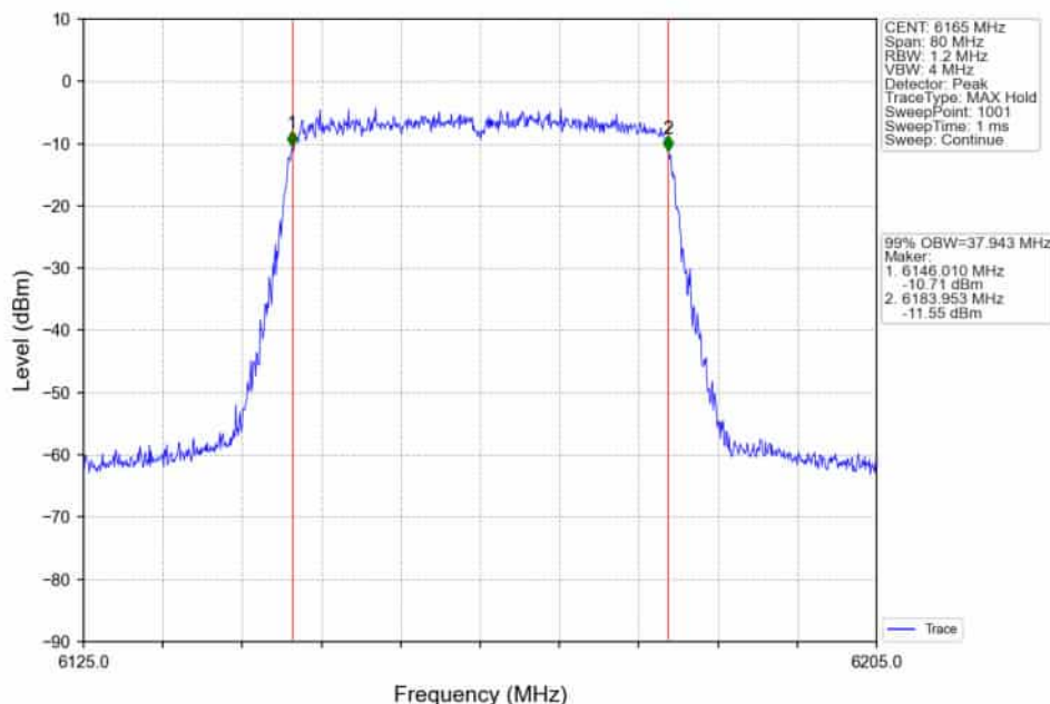
802.11ax(HEW40)_MCH_6165MHz_RU484_Left_Ant2_NTNV
