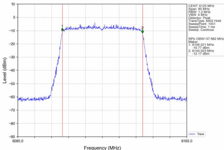
802.11ax(HEW40)_LCH_6125MHz_RU484_Left_Ant2_NTNV
