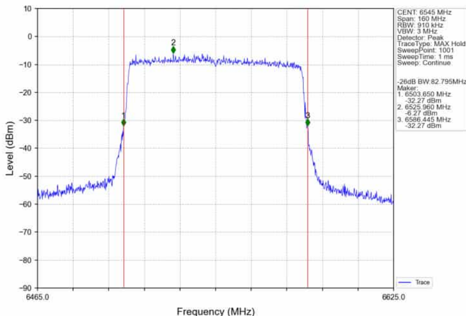
802.11ax(HEW80)_HCH_6545MHz_RU996_Left_Ant2_NTNV
