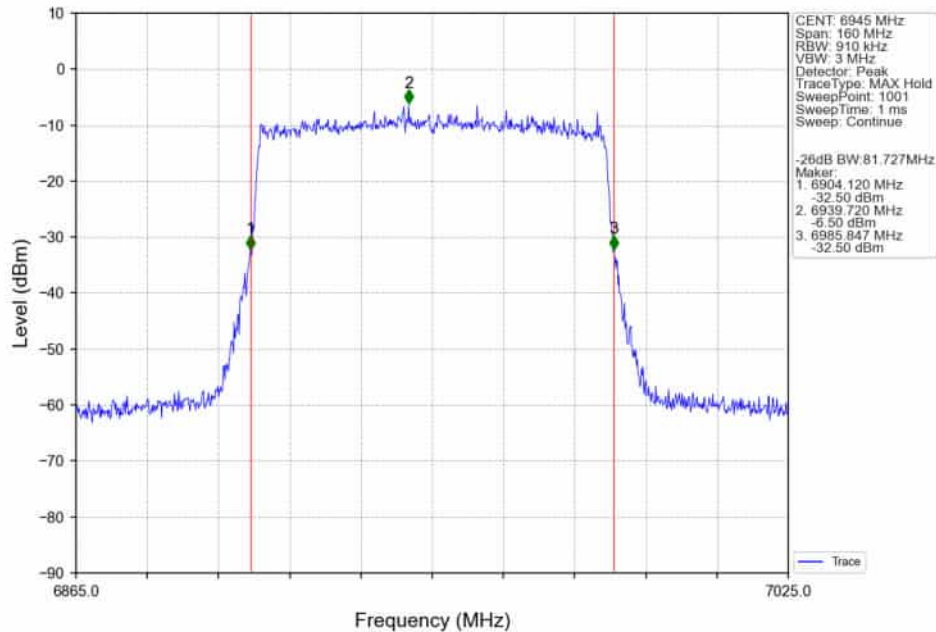
802.11ax(HEW80)_LCH_6945MHz_RU996_Left_Ant2_NTNV
