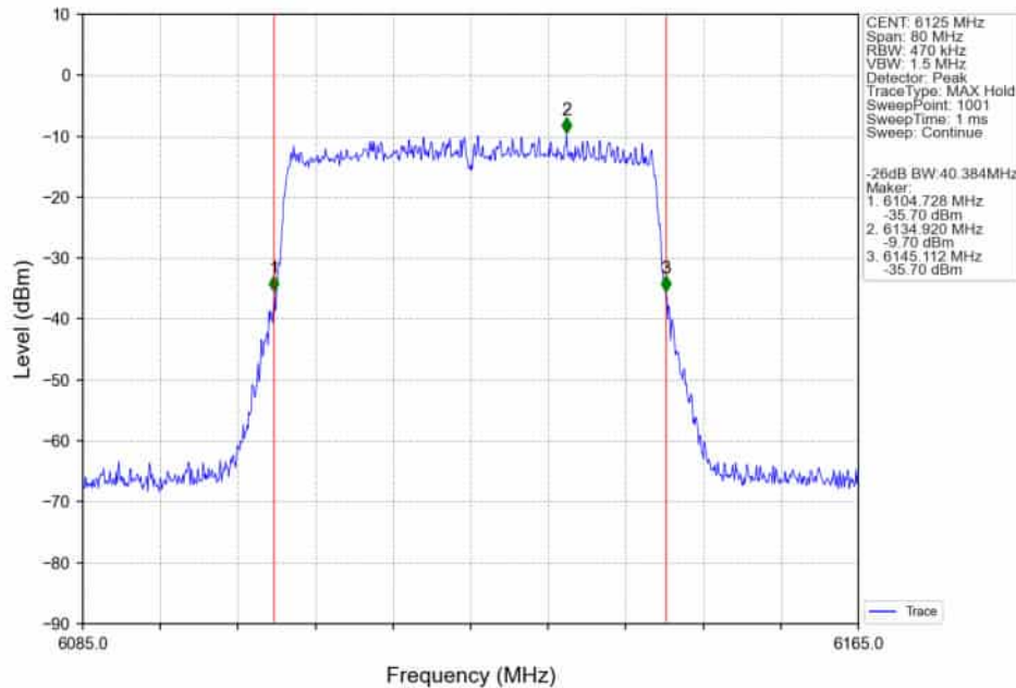
802.11ax(HEW40)_LCH_6125MHz_RU484_Left_Ant2_NTNV
