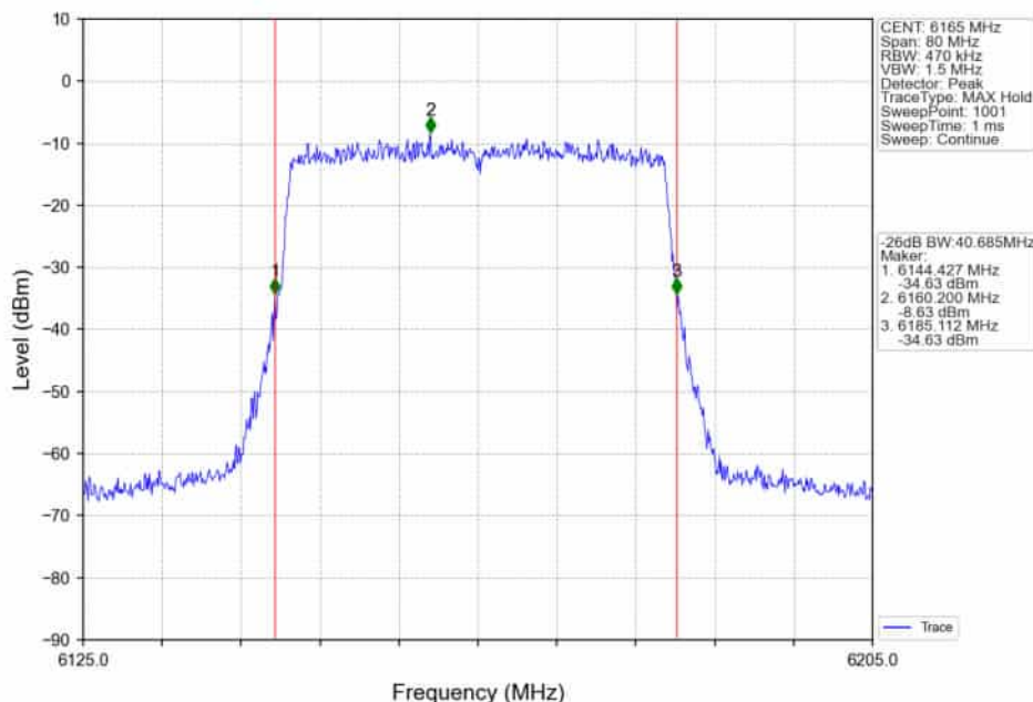
802.11ax(HEW40)_MCH_6165MHz_RU484_Left_Ant2_NTNV
