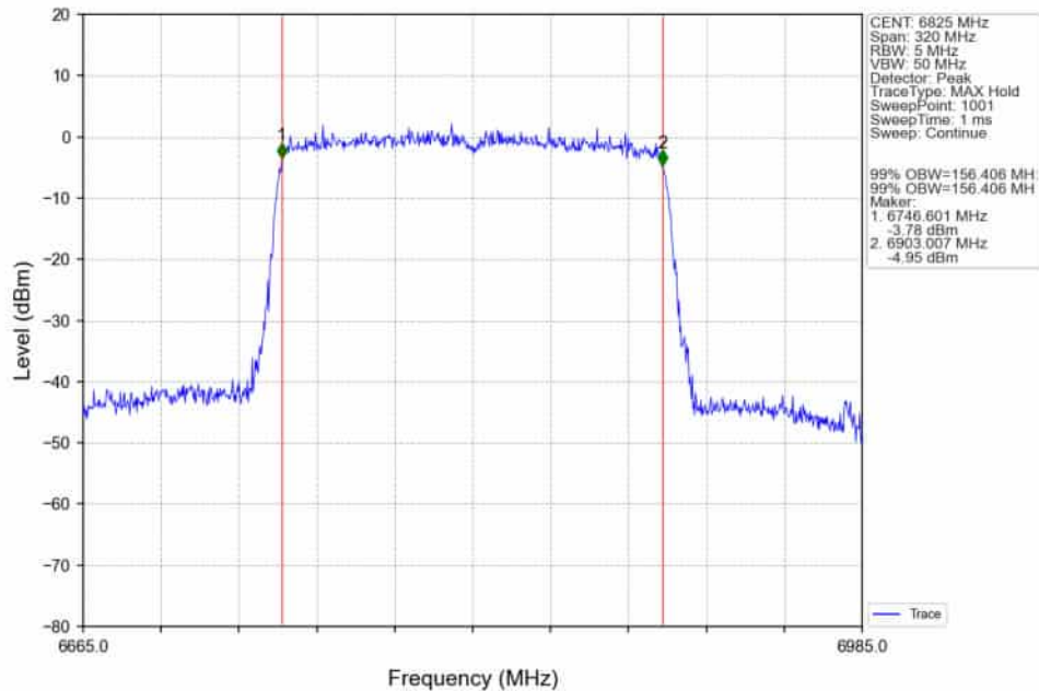
802.11ax(HEW160)_HCH_6825MHz_2xRU996_Left_Ant2_NTNV
