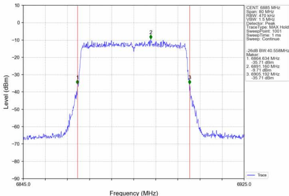
802.11ax(HEW40)_HCH_6885MHz_RU484_Left_Ant2_NTNV
