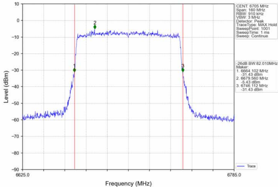
802.11ax(HEW80)_MCH_6705MHz_RU996_Left_Ant2_NTNV
