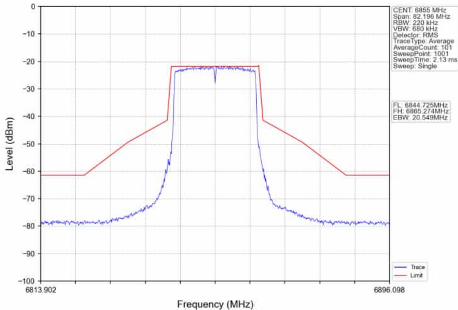
802.11ax(HEW20)_HCH_6855MHz_RU242_Left_Ant2_NTNV
