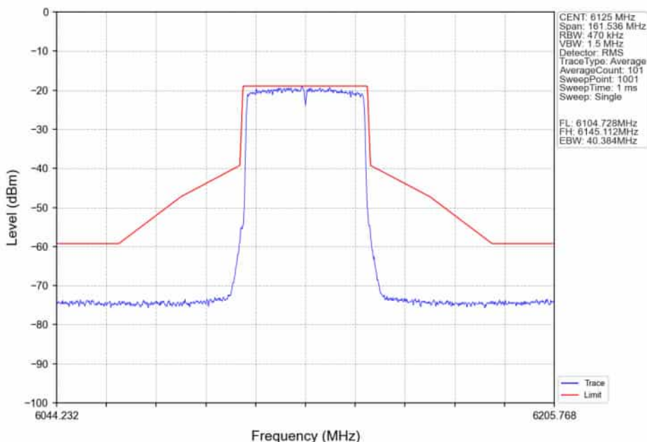
802.11ax(HEW40)_LCH_6125MHz_RU484_Left_Ant2_NTNV
