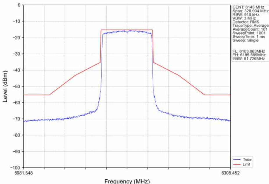
802.11ax(HEW80)_LCH_6145MHz_RU996_Left_Ant2_NTNV
