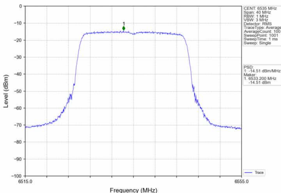
802.11ax(HEW20)_LCH_6535MHz_RU242_Left_Ant2_NTNV
