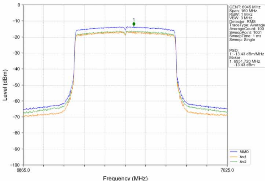
802.11ax(HEW80)_HCH_7025MHz_RU996_Left_Ant1_NTNV
