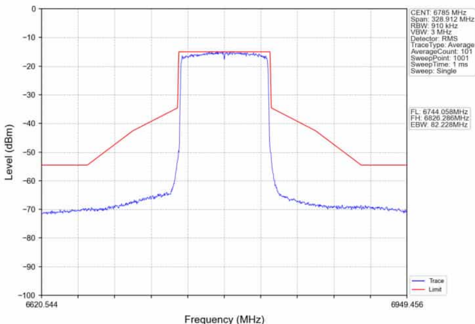
802.11ax(HEW80)_HCH_6785MHz_RU996_Left_Ant2_NTNV
