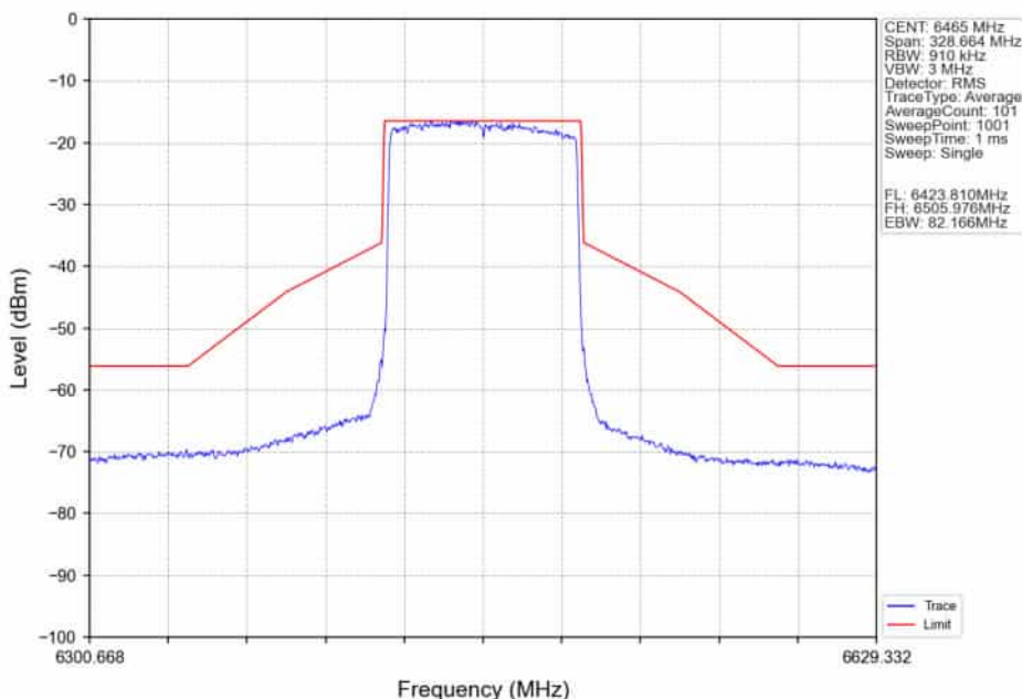
802.11ax(HEW80)_LCH_6465MHz_RU996_Left_Ant2_NTNV
