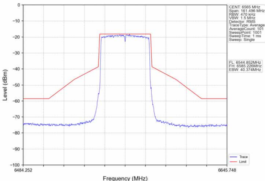
802.11ax(HEW40)_LCH_6565MHz_RU484_Left_Ant2_NTNV
