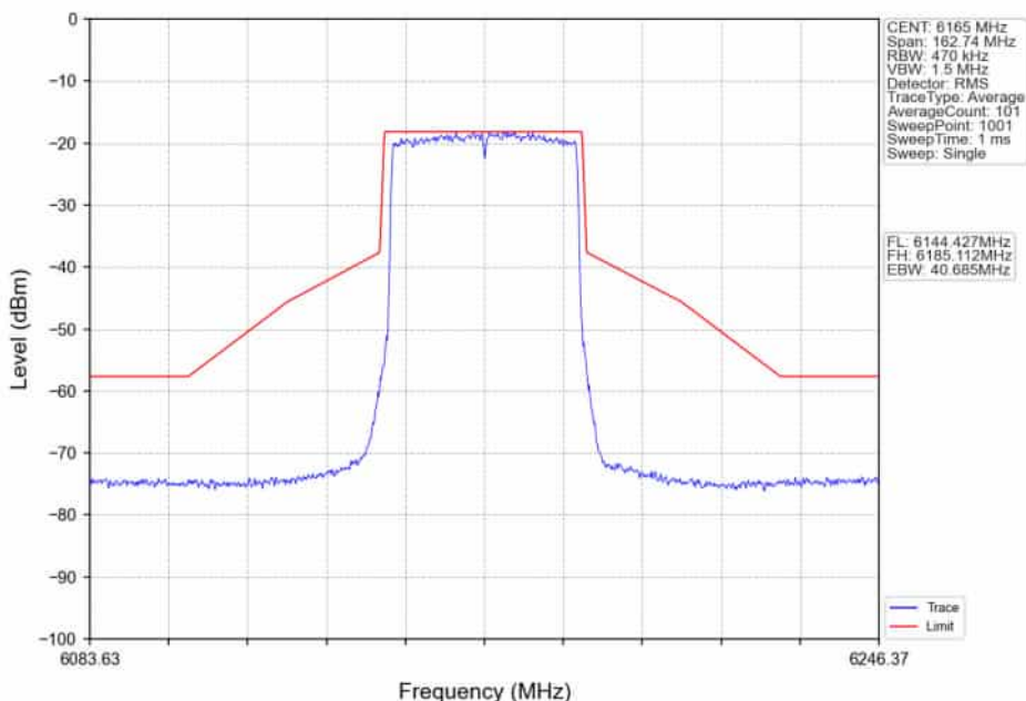
802.11ax(HEW40)_MCH_6165MHz_RU484_Left_Ant2_NTNV
