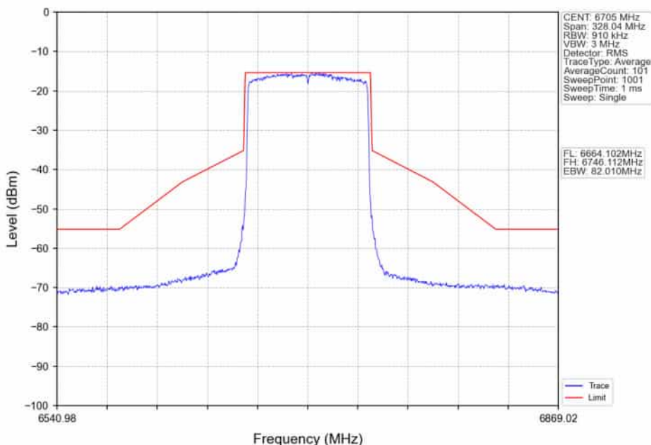
802.11ax(HEW80)_MCH_6705MHz_RU996_Left_Ant2_NTNV
