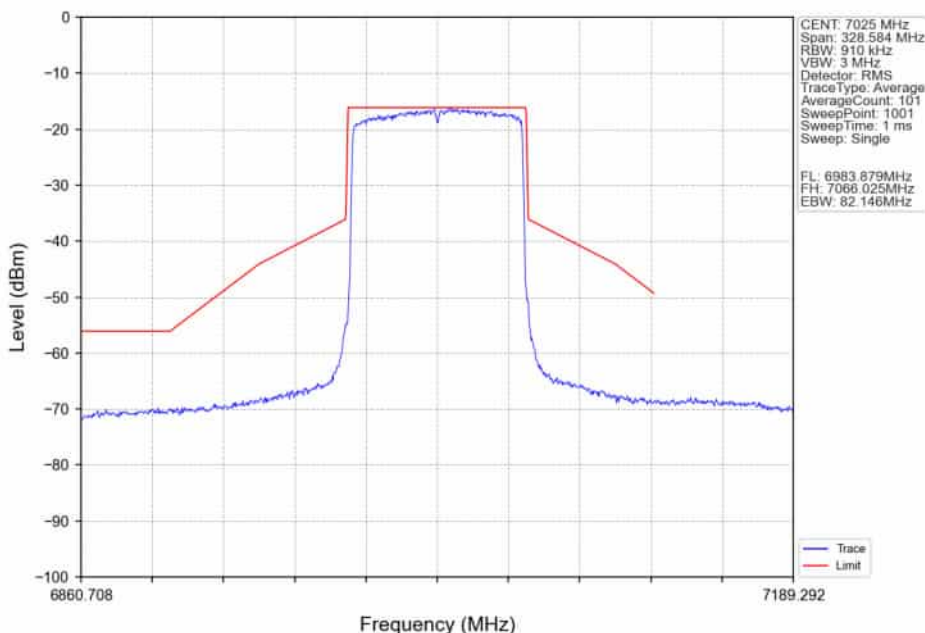
802.11ax(HEW80)_HCH_7025MHz_RU996_Left_Ant2_NTNV
