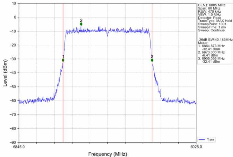
802.11ax(HEW40)_HCH_6885MHz_RU484_Left_Ant2_NTNV
