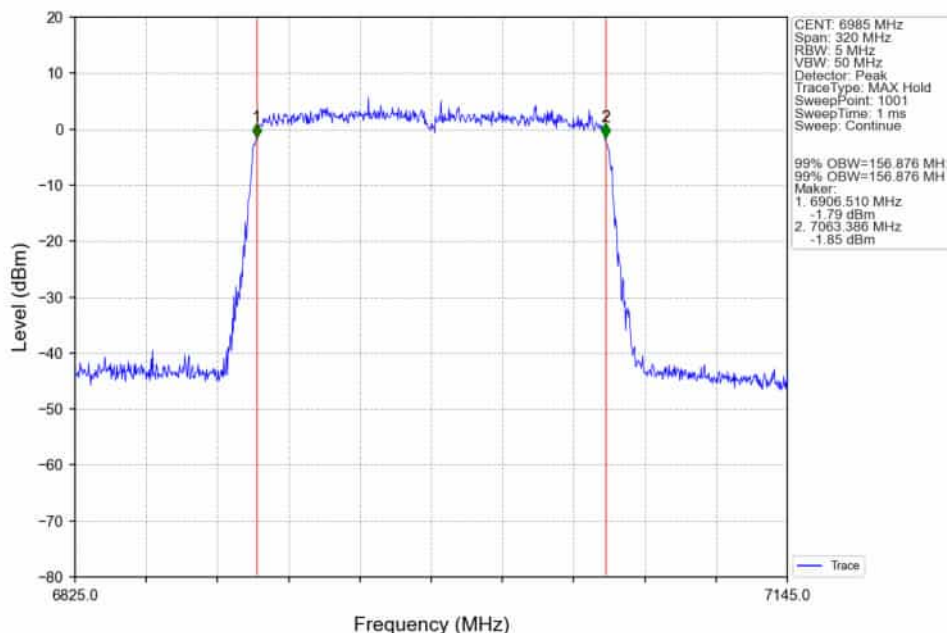
802.11ax(HEW160)_MCH_6985MHz_2xRU996_Left_Ant2_NTNV
