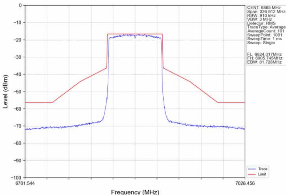
802.11ax(HEW80)_HCH_6865MHz_RU996_Left_Ant2_NTNV
