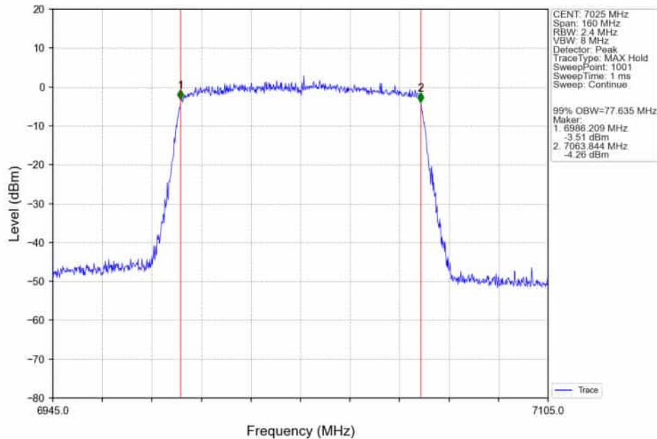
802.11ax(HEW80)_HCH_7025MHz_RU996_Left_Ant2_NTNV
