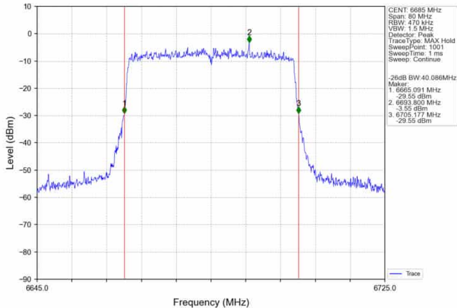
802.11ax(HEW40)_MCH_6685MHz_RU484_Left_Ant2_NTNV
