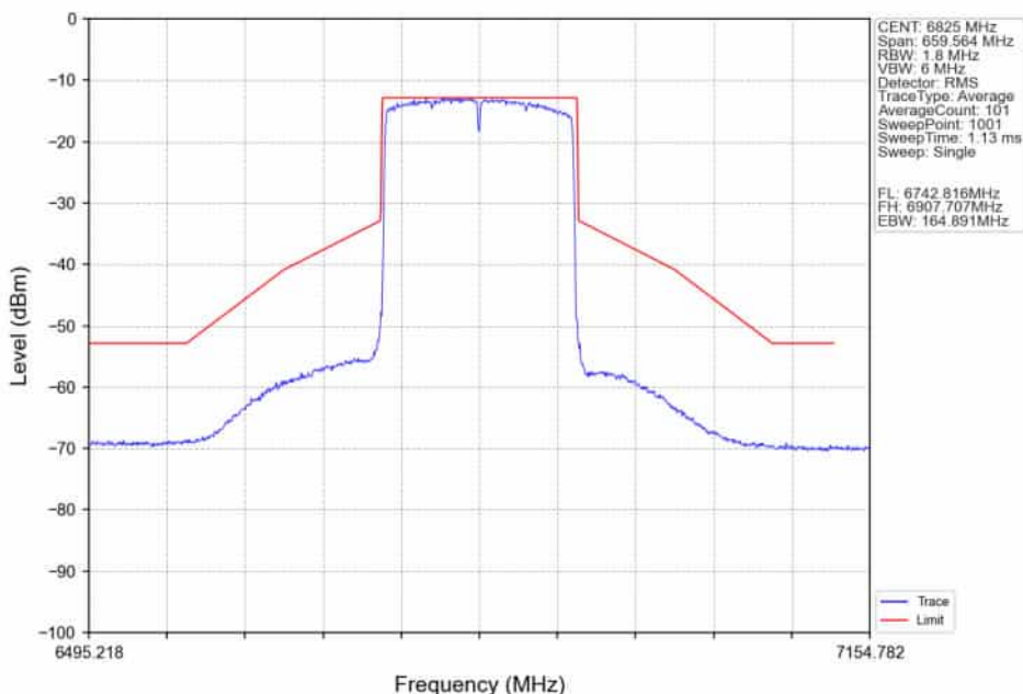
802.11ax(HEW160)_HCH_6825MHz_2xRU996_Left_Ant2_NTNV
