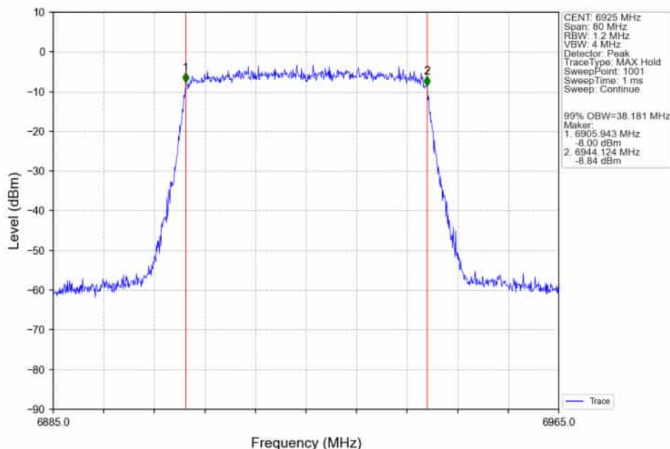
802.11ax(HEW40)_LCH_6925MHz_RU484_Left_Ant2_NTNV
