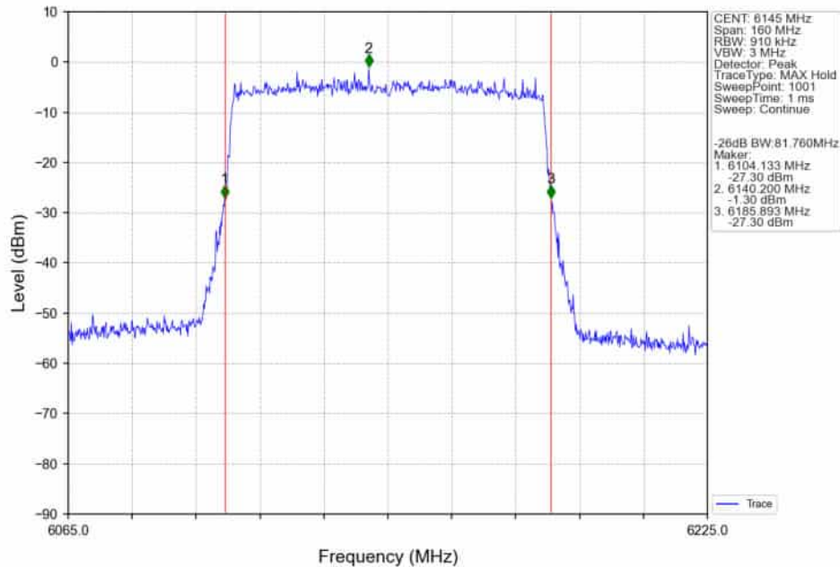
802.11ax(HEW80)_LCH_6145MHz_RU996_Left_Ant2_NTNV
