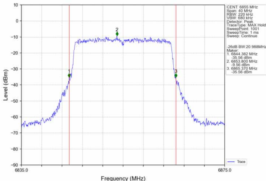
802.11ax(HEW20)_HCH_6855MHz_RU242_Left_Ant2_NTNV
