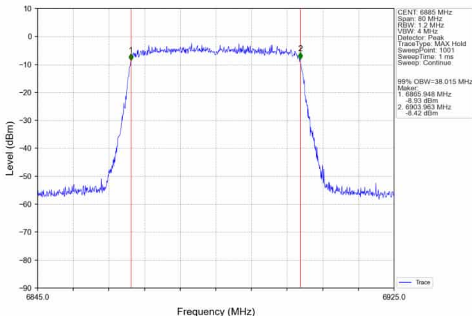
802.11ax(HEW40)_HCH_6885MHz_RU484_Left_Ant2_NTNV
