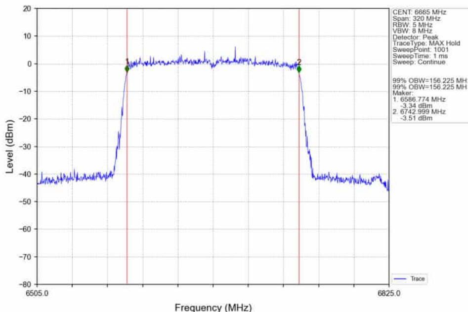
802.11ax(HEW160)_MCH_6665MHz_2xRU996_Left_Ant2_NTNV
