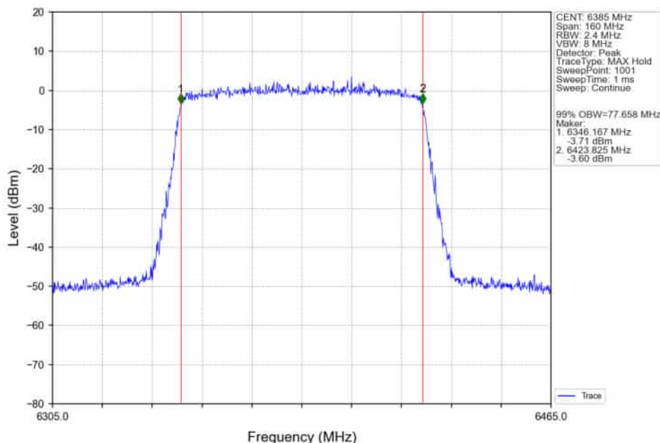
802.11ax(HEW80)_HCH_6385MHz_RU996_Left_Ant2_NTNV
