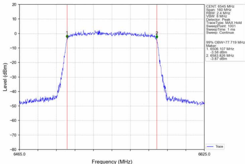
802.11ax(HEW80)_HCH_6545MHz_RU996_Left_Ant2_NTNV
