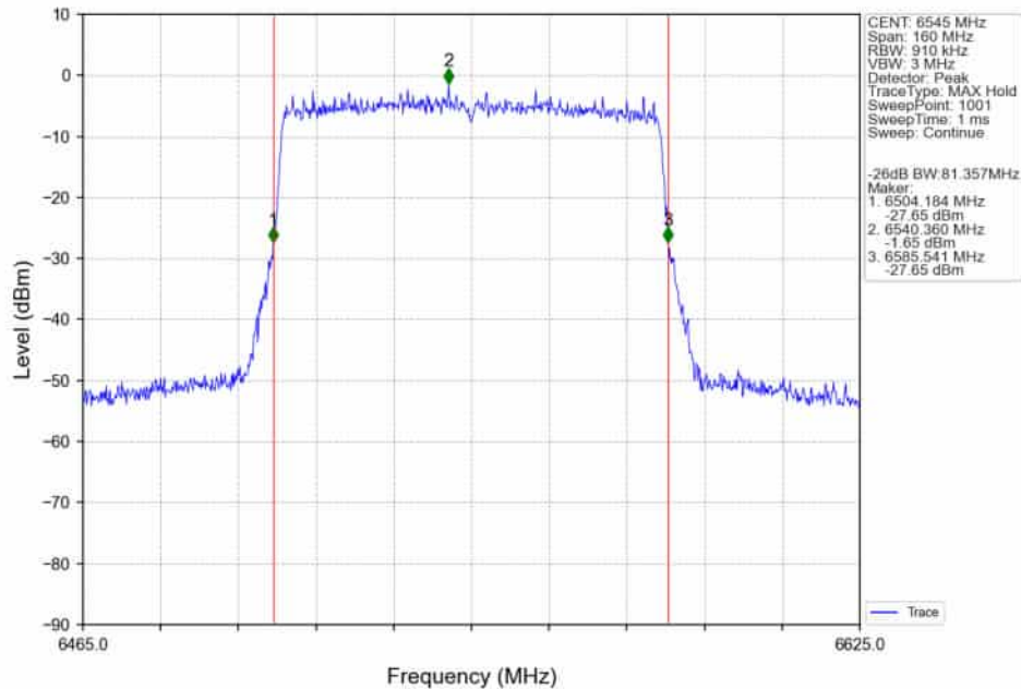
802.11ax(HEW80)_HCH_6545MHz_RU996_Left_Ant2_NTNV
