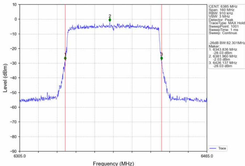
802.11ax(HEW80)_HCH_6385MHz_RU996_Left_Ant2_NTNV
