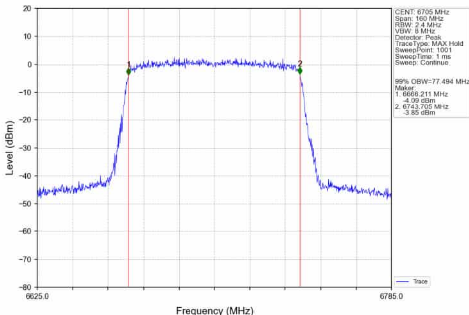
802.11ax(HEW80)_MCH_6705MHz_RU996_Left_Ant2_NTNV
