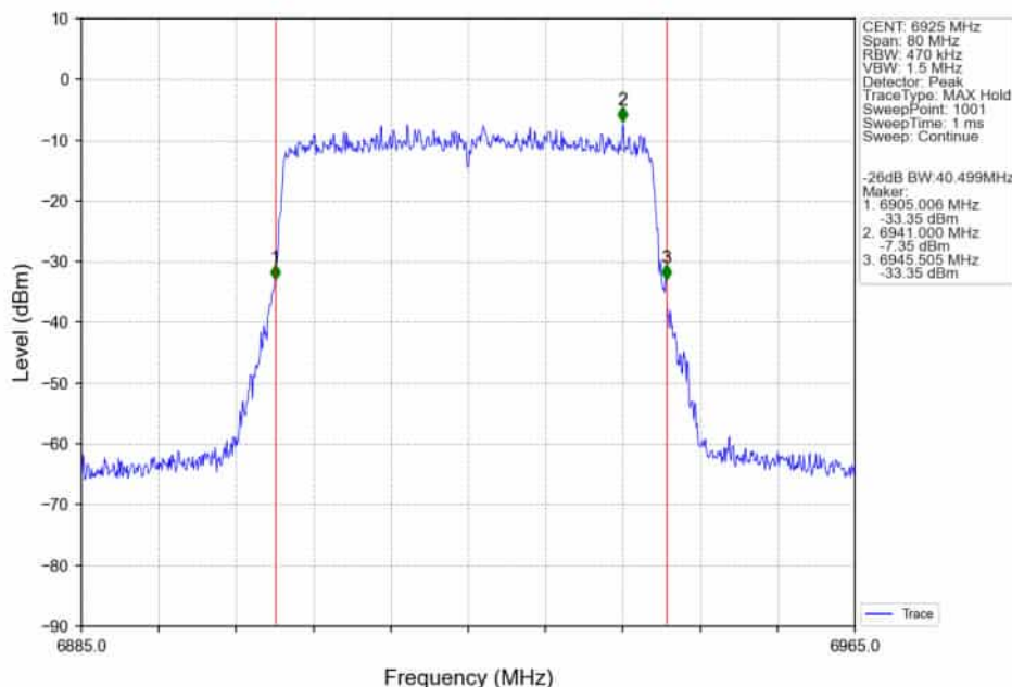
802.11ax(HEW40)_LCH_6925MHz_RU484_Left_Ant2_NTNV
