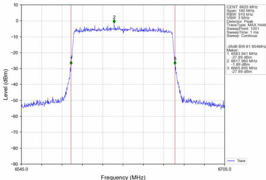
802.11ax(HEW80)_LCH_6625MHz_RU996_Left_Ant2_NTNV
