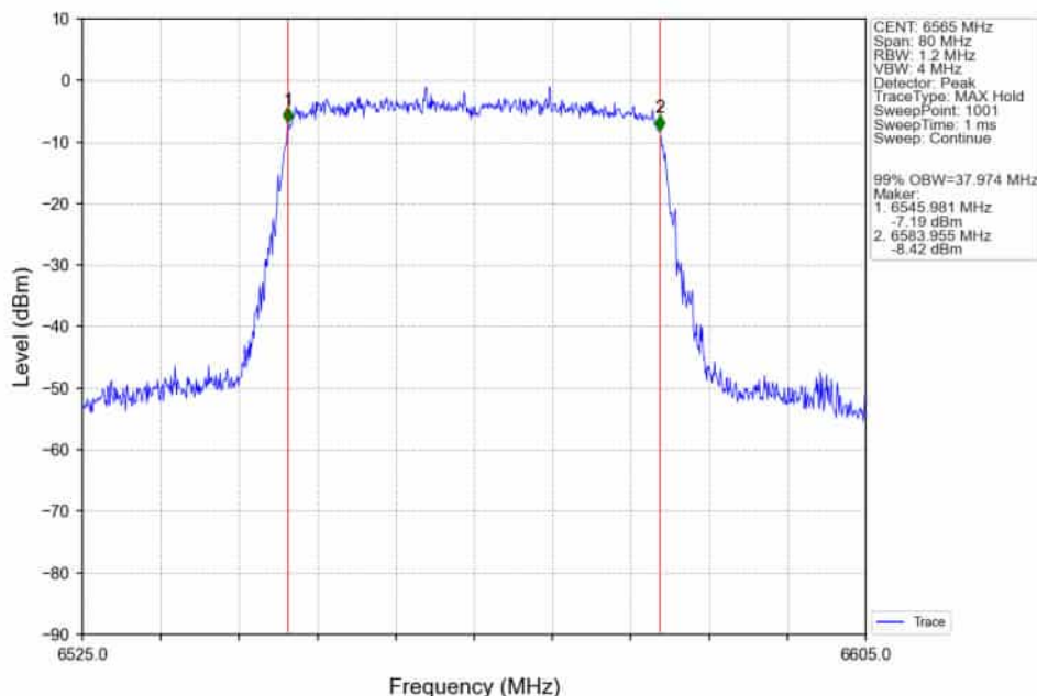
802.11ax(HEW40)_LCH_6565MHz_RU484_Left_Ant2_NTNV
