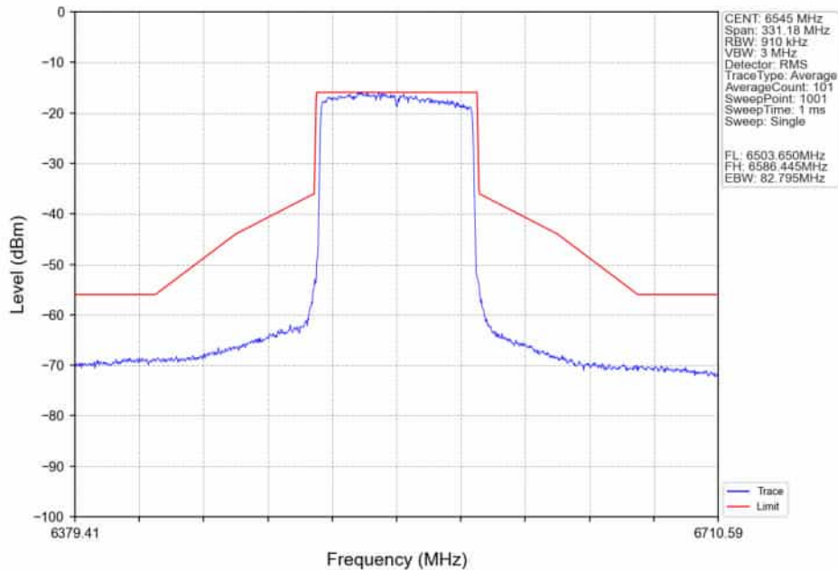
802.11ax(HEW80)_HCH_6545MHz_RU996_Left_Ant2_NTNV
