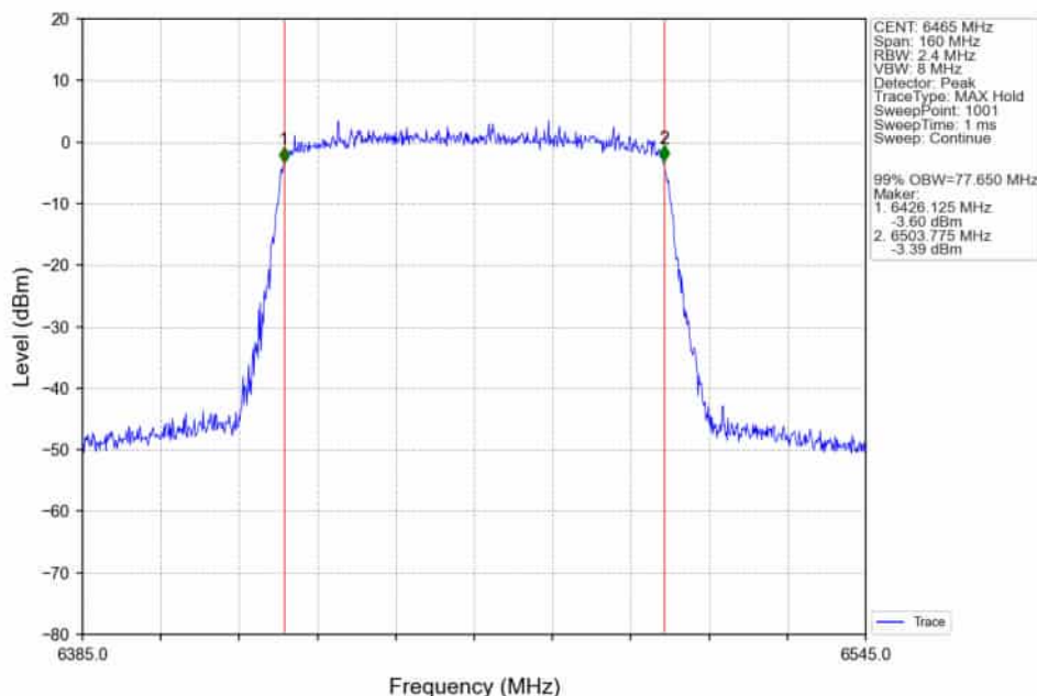
802.11ax(HEW80)_LCH_6465MHz_RU996_Left_Ant2_NTNV
