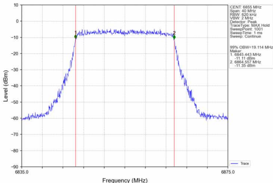
802.11ax(HEW20)_HCH_6855MHz_RU242_Left_Ant2_NTNV
