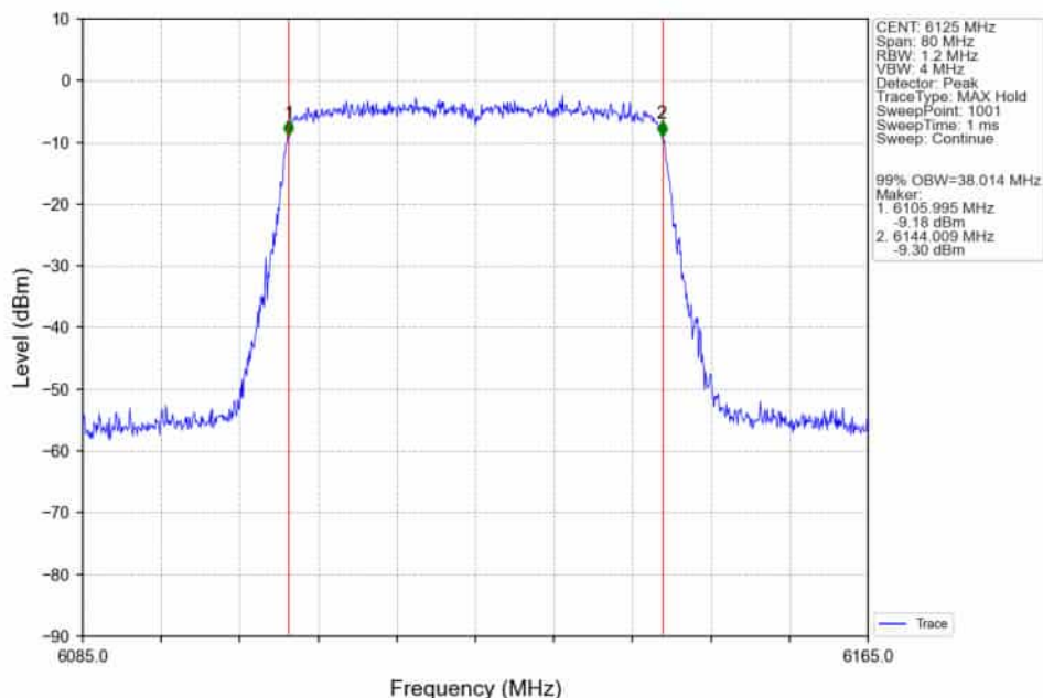
802.11ax(HEW40)_LCH_6125MHz_RU484_Left_Ant2_NTNV
