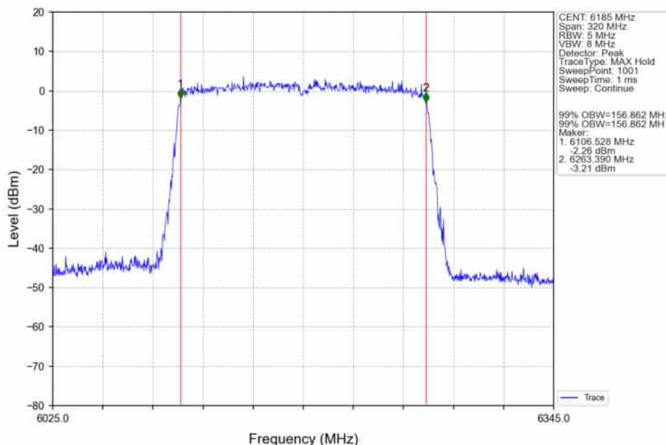
802.11ax(HEW160)_MCH_6185MHz_2xRU996_Left_Ant2_NTNV
