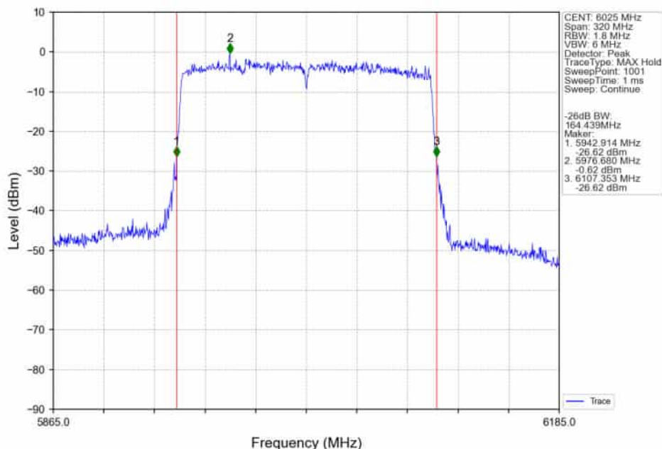
802.11ax(HEW160)_LCH_6025MHz_2xRU996_Left_Ant2_NTNV
