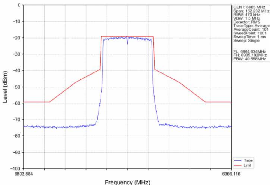
802.11ax(HEW40)_HCH_6885MHz_RU484_Left_Ant2_NTNV
