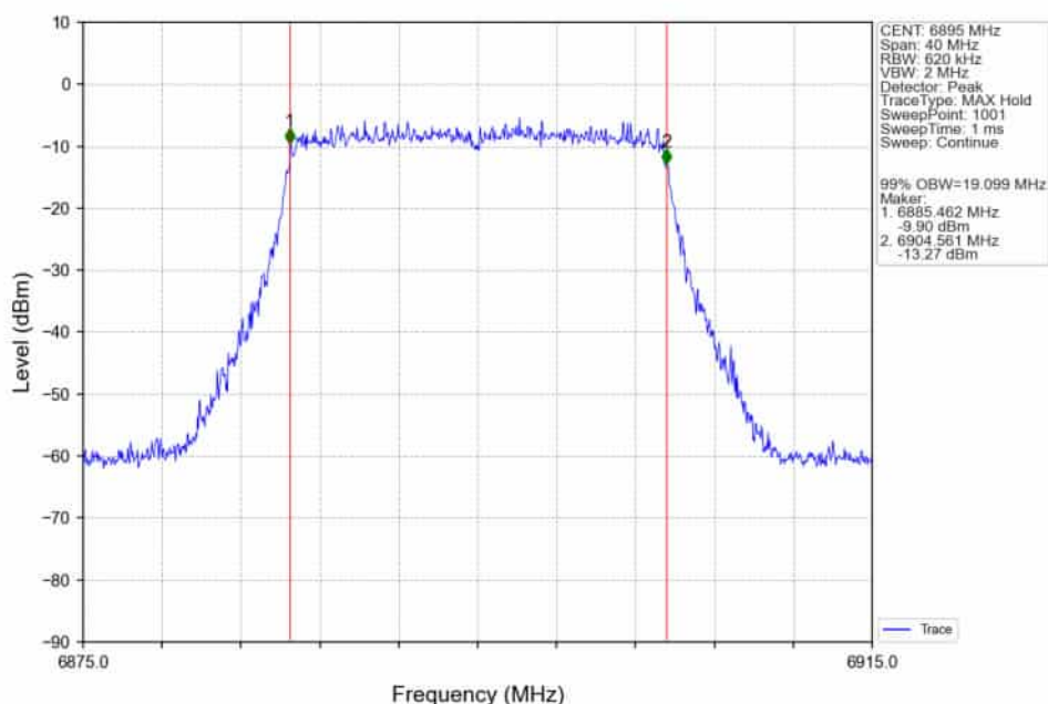
802.11ax(HEW20)_LCH_6895MHz_RU242_Left_Ant2_NTNV
