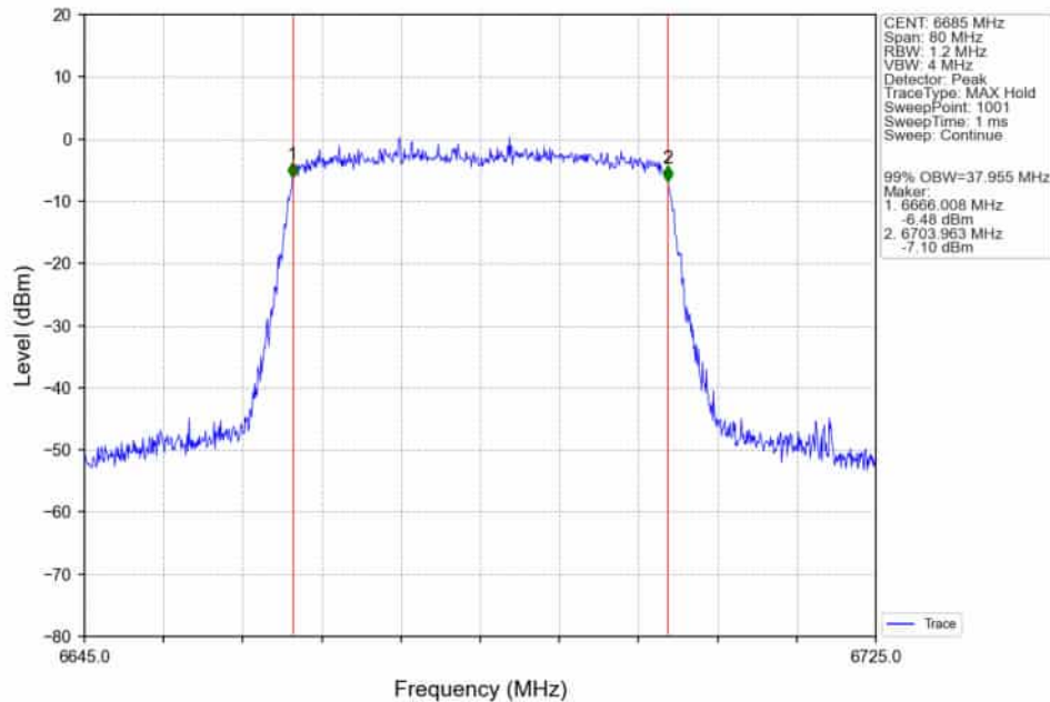
802.11ax(HEW40)_MCH_6685MHz_RU484_Left_Ant2_NTNV
