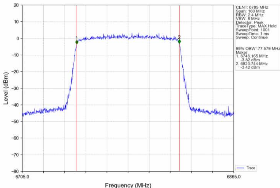
802.11ax(HEW80)_HCH_6785MHz_RU996_Left_Ant2_NTNV
