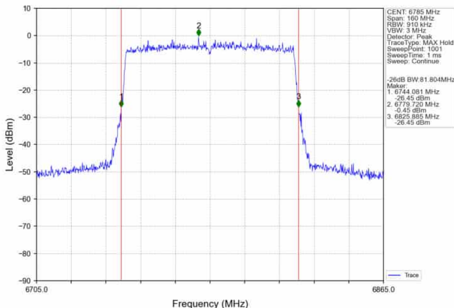
802.11ax(HEW80)_HCH_6785MHz_RU996_Left_Ant2_NTNV
