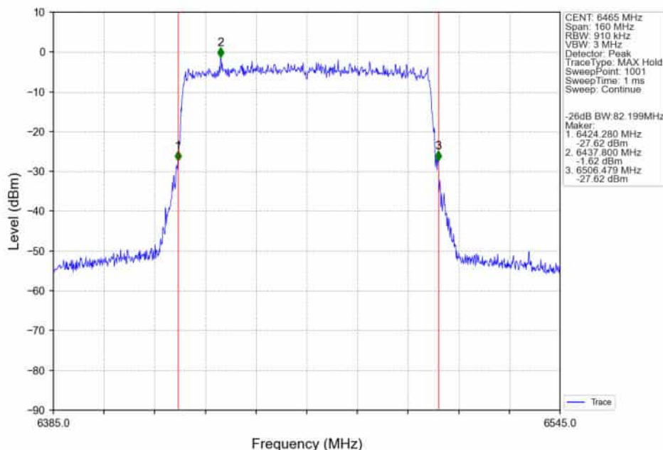
802.11ax(HEW80)_LCH_6465MHz_RU996_Left_Ant2_NTNV
