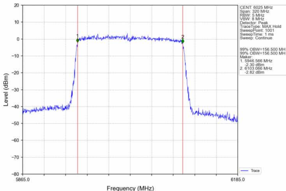
802.11ax(HEW160)_LCH_6025MHz_2xRU996_Left_Ant2_NTNV
