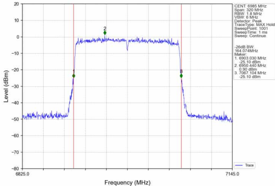
802.11ax(HEW160)_MCH_6985MHz_2xRU996_Left_Ant2_NTNV
