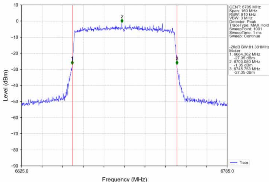
802.11ax(HEW80)_MCH_6705MHz_RU996_Left_Ant2_NTNV
