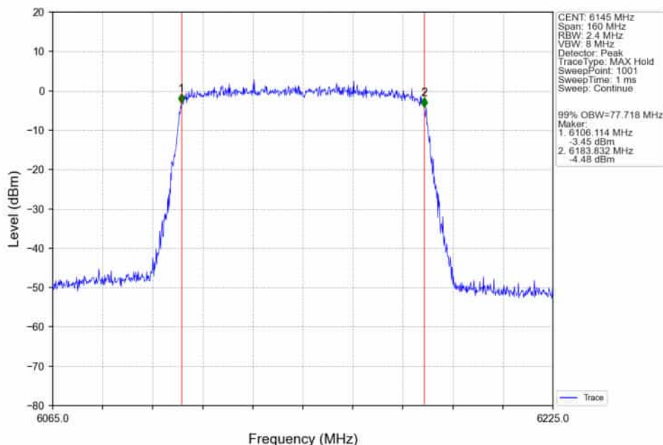
802.11ax(HEW80)_LCH_6145MHz_RU996_Left_Ant2_NTNV
