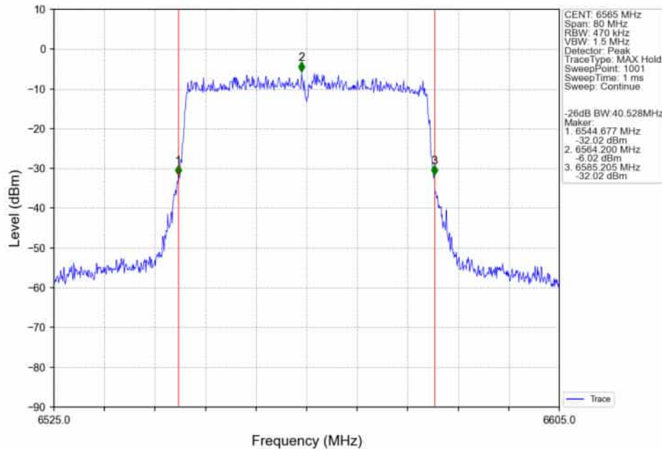
802.11ax(HEW40)_LCH_6565MHz_RU484_Left_Ant2_NTNV
