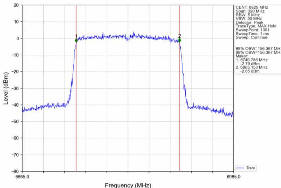
802.11ax(HEW160)_HCH_6825MHz_2xRU996_Left_Ant2_NTNV
