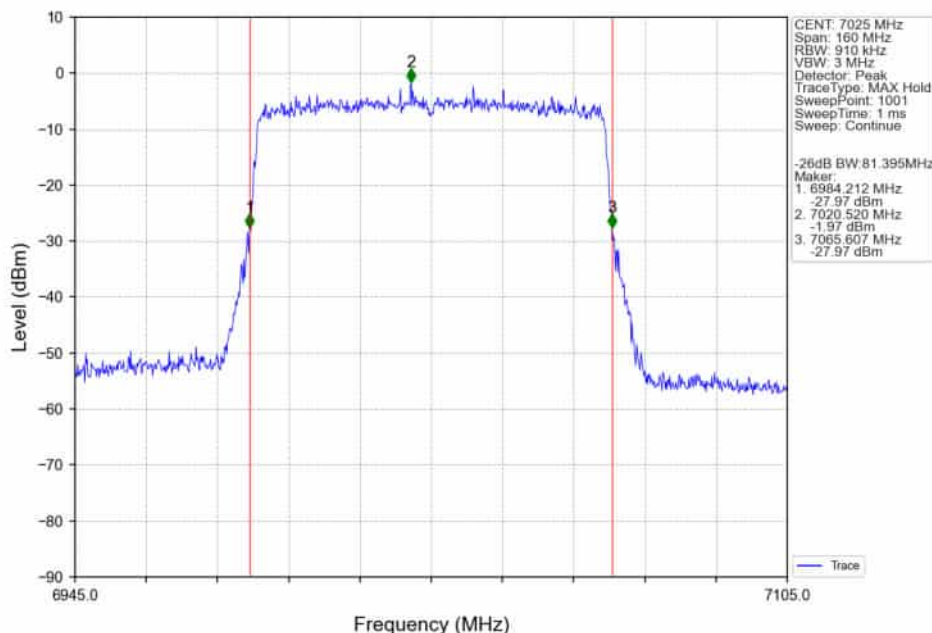
802.11ax(HEW80)_HCH_7025MHz_RU996_Left_Ant2_NTNV
