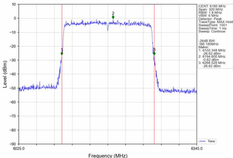
802.11ax(HEW160)_MCH_6185MHz_2xRU996_Left_Ant2_NTNV
