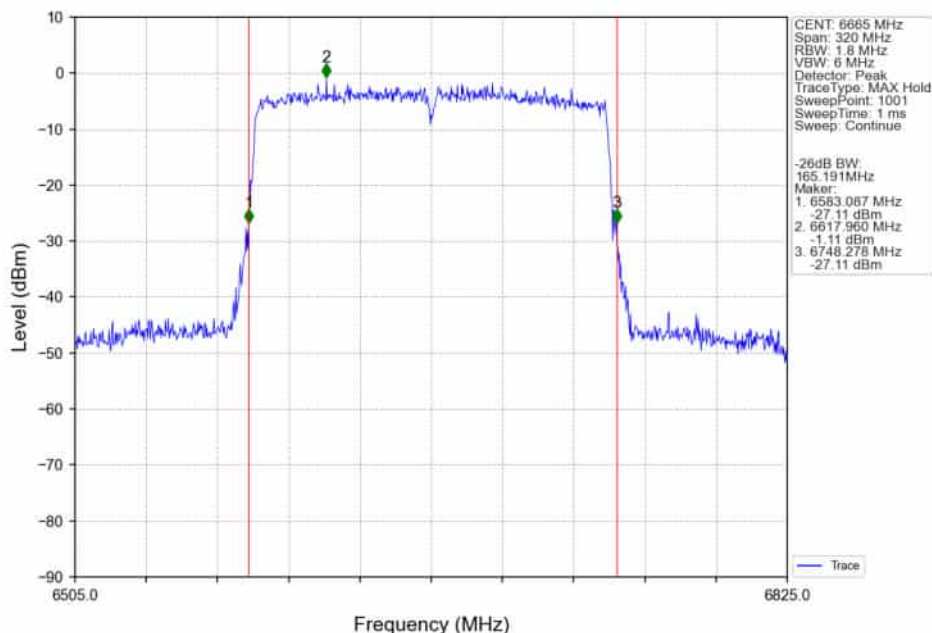
802.11ax(HEW160)_MCH_6665MHz_2xRU996_Left_Ant2_NTNV
