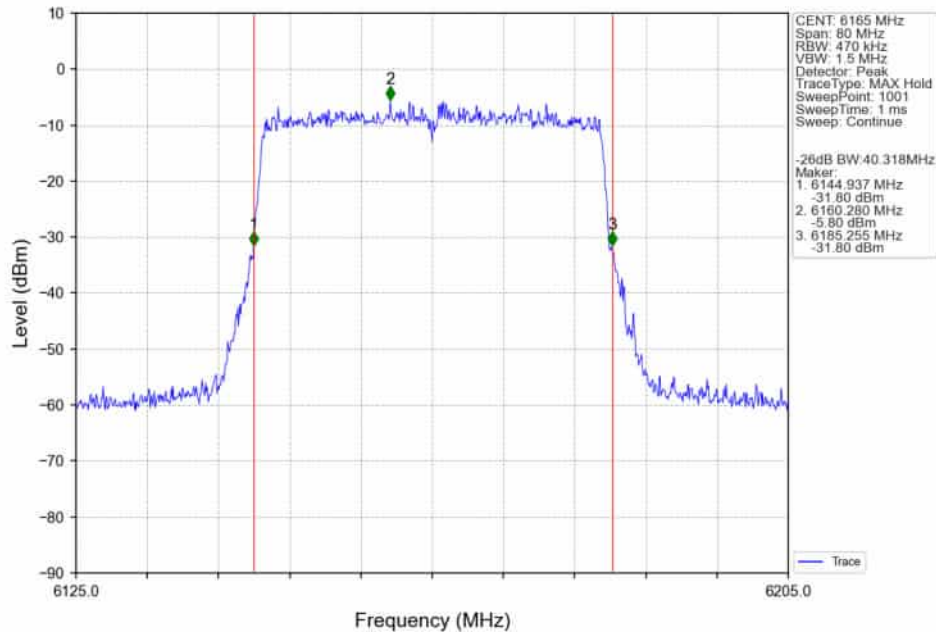
802.11ax(HEW40)_MCH_6165MHz_RU484_Left_Ant2_NTNV
