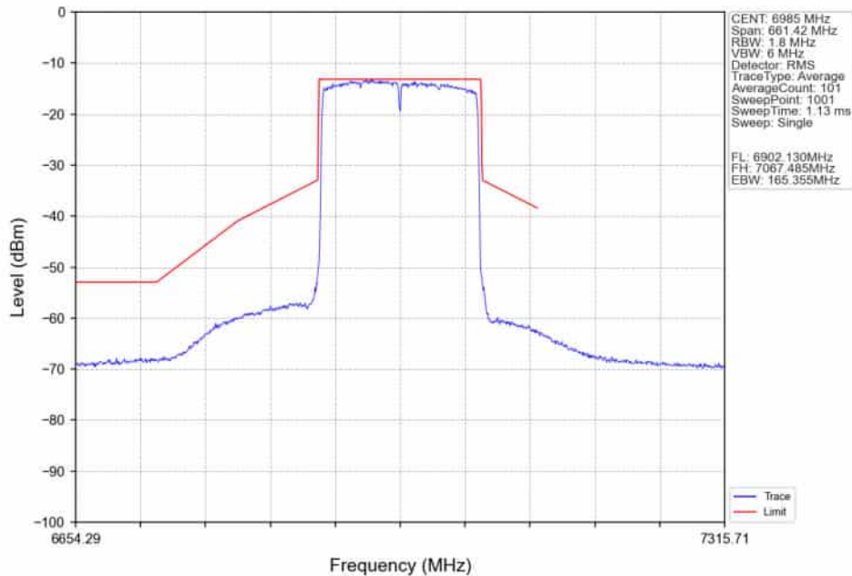
802.11ax(HEW160)_MCH_6985MHz_2xRU996_Left_Ant2_NTNV
