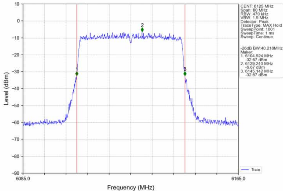
802.11ax(HEW40)_LCH_6125MHz_RU484_Left_Ant2_NTNV
