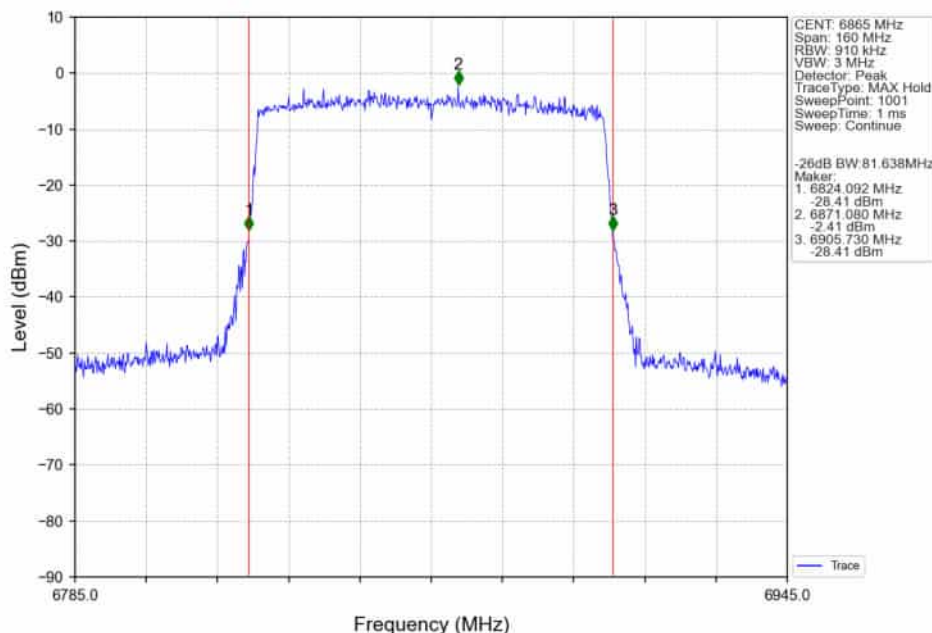
802.11ax(HEW80)_HCH_6865MHz_RU996_Left_Ant2_NTNV
