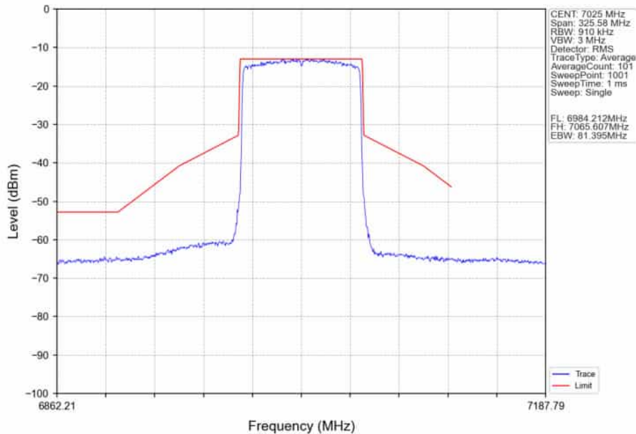
802.11ax(HEW80)_HCH_7025MHz_RU996_Left_Ant2_NTNV
