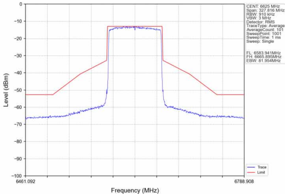
802.11ax(HEW80)_LCH_6625MHz_RU996_Left_Ant2_NTNV
