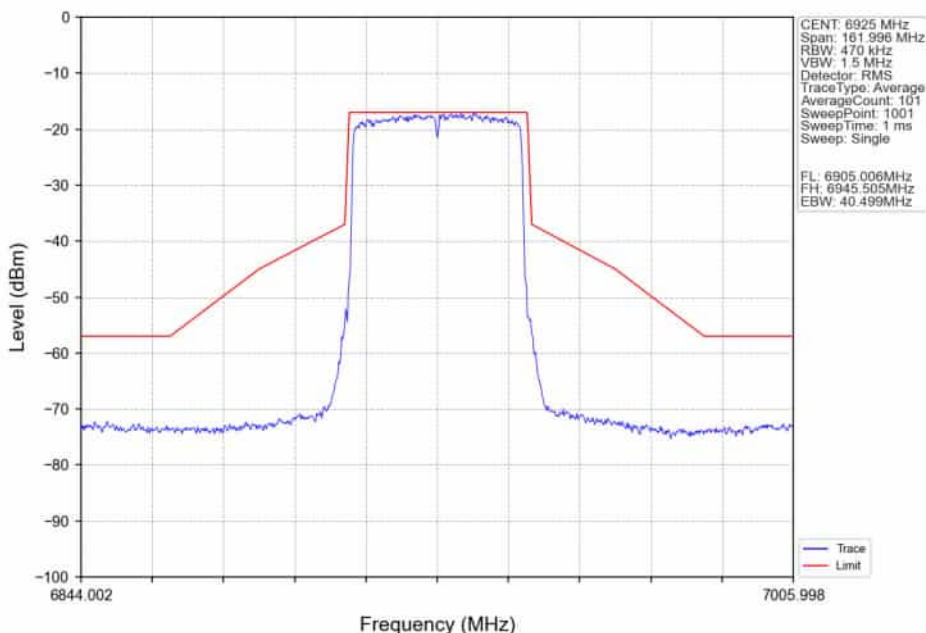
802.11ax(HEW40)_LCH_6925MHz_RU484_Left_Ant2_NTNV
