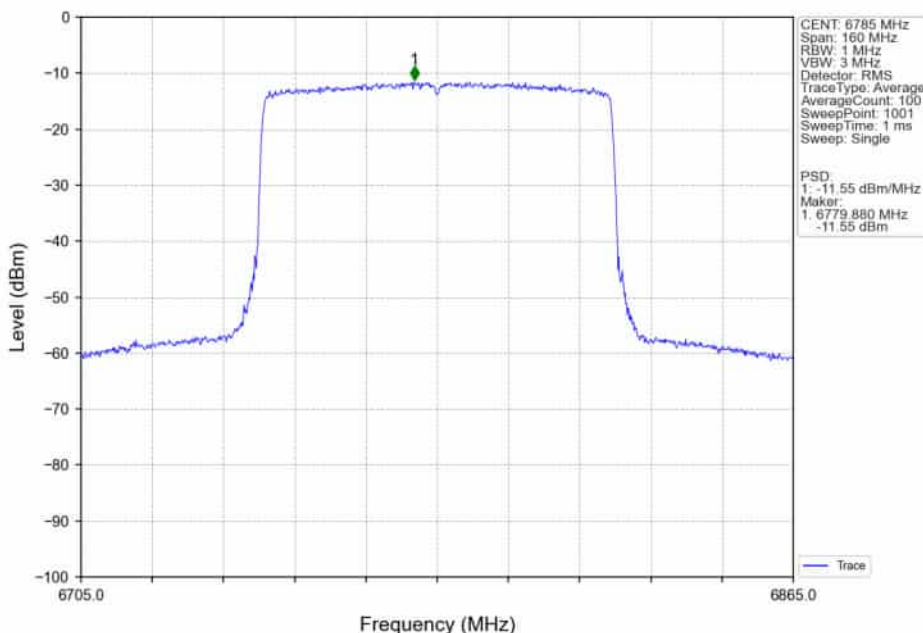
802.11ax(HEW80)_HCH_6785MHz_RU996_Left_Ant2_NTNV
