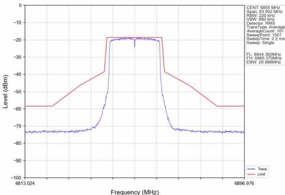
802.11ax(HEW20)_HCH_6855MHz_RU242_Left_Ant2_NTNV
