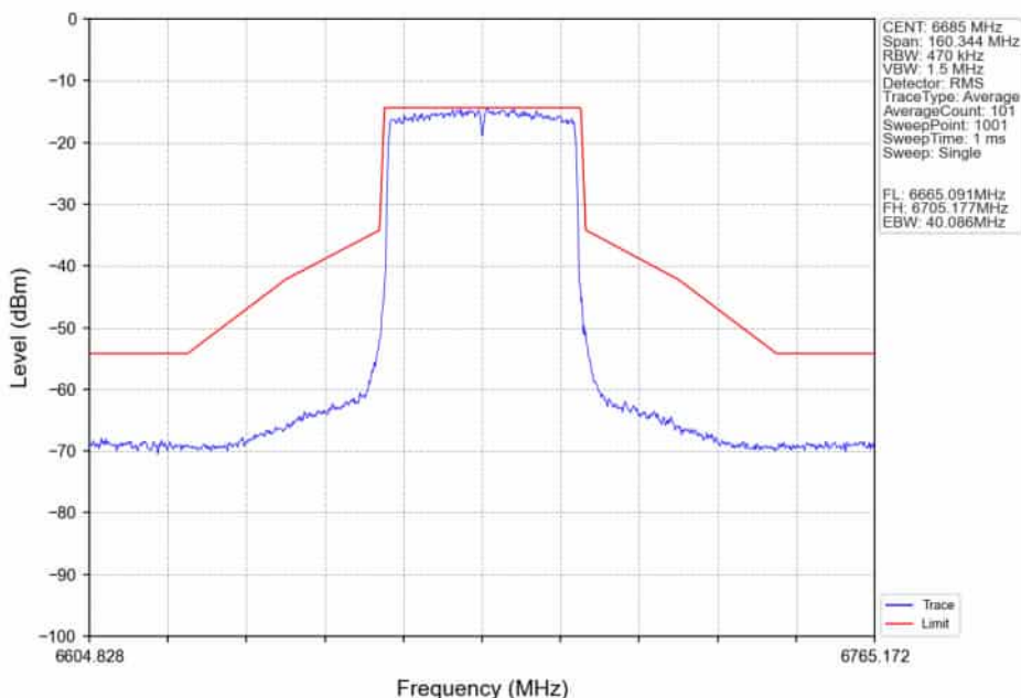
802.11ax(HEW40)_MCH_6685MHz_RU484_Left_Ant2_NTNV
