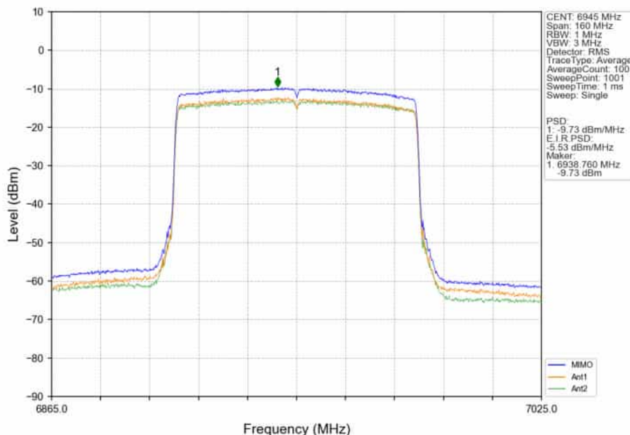
802.11ax(HEW80)_HCH_7025MHz_RU996_Left_Ant1_NTNV
