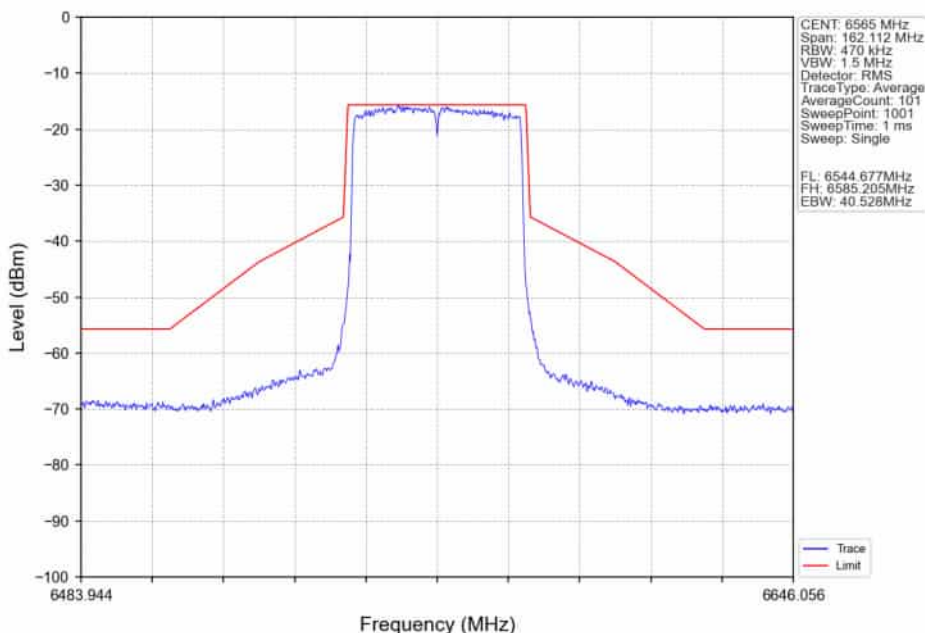
802.11ax(HEW40)_LCH_6565MHz_RU484_Left_Ant2_NTNV
