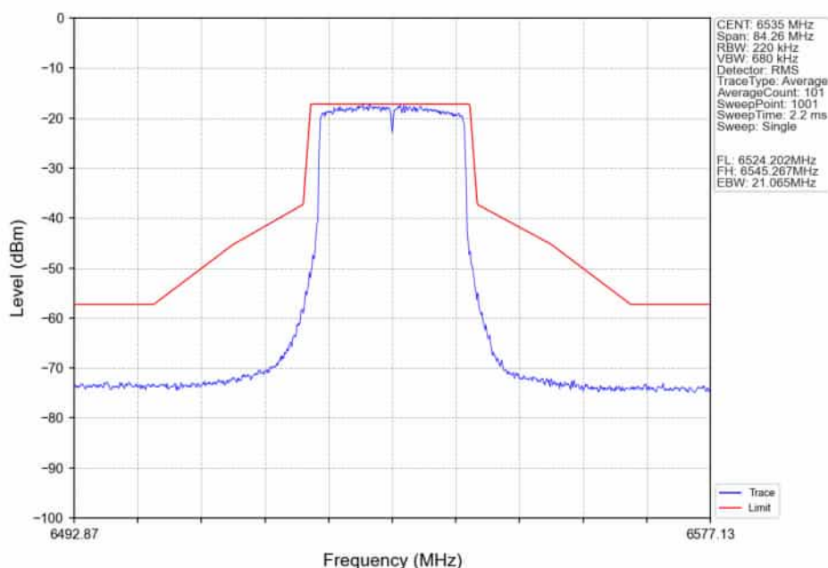
802.11ax(HEW20)_LCH_6535MHz_RU242_Left_Ant2_NTNV
