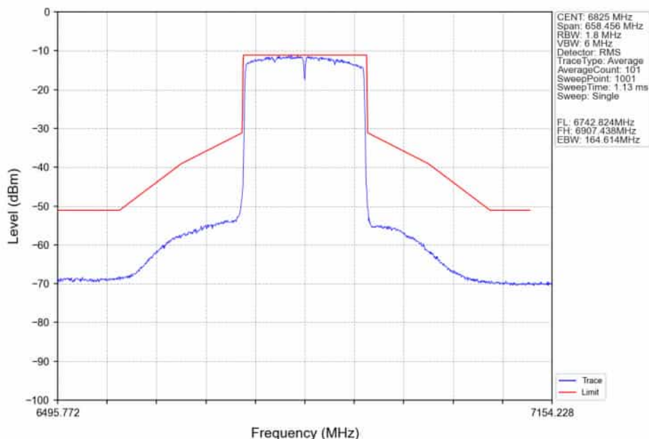
802.11ax(HEW160)_HCH_6825MHz_2xRU996_Left_Ant2_NTNV
