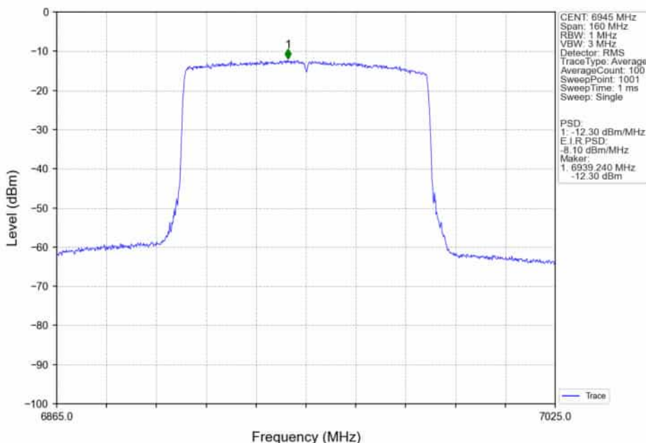
802.11ax(HEW80)_LCH_6945MHz_RU996_Left_Ant2_NTNV
