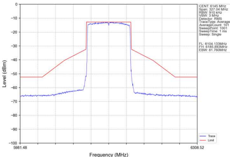
802.11ax(HEW80)_LCH_6145MHz_RU996_Left_Ant2_NTNV
