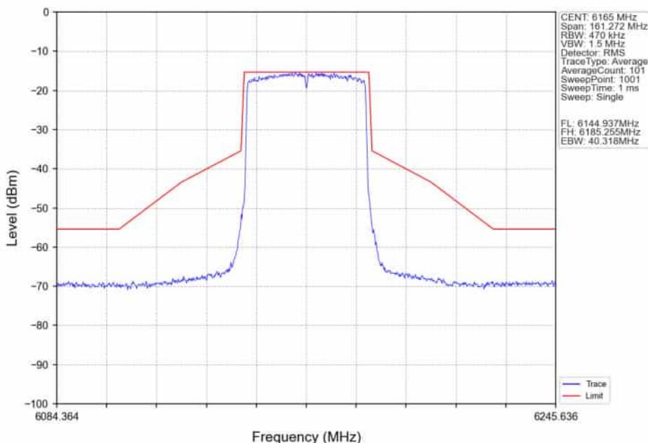
802.11ax(HEW40)_MCH_6165MHz_RU484_Left_Ant2_NTNV
