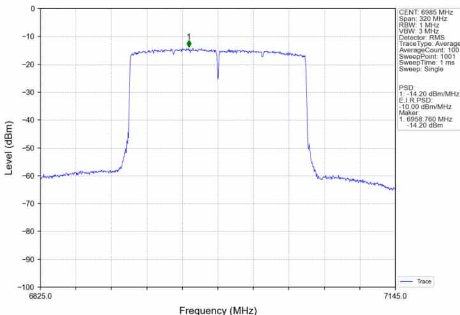
802.11ax(HEW160)_MCH_6985MHz_2xRU996_Left_Ant2_NTNV
