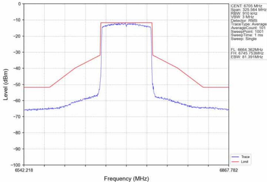
802.11ax(HEW80)_MCH_6705MHz_RU996_Left_Ant2_NTNV
