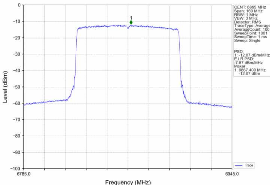
802.11ax(HEW80)_HCH_6865MHz_RU996_Left_Ant2_NTNV
