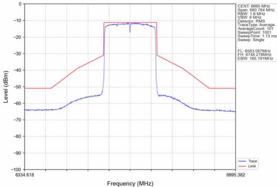
802.11ax(HEW160)_MCH_6665MHz_2xRU996_Left_Ant2_NTNV
