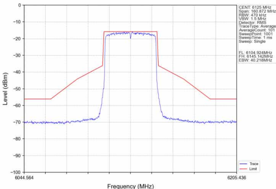
802.11ax(HEW40)_LCH_6125MHz_RU484_Left_Ant2_NTNV
