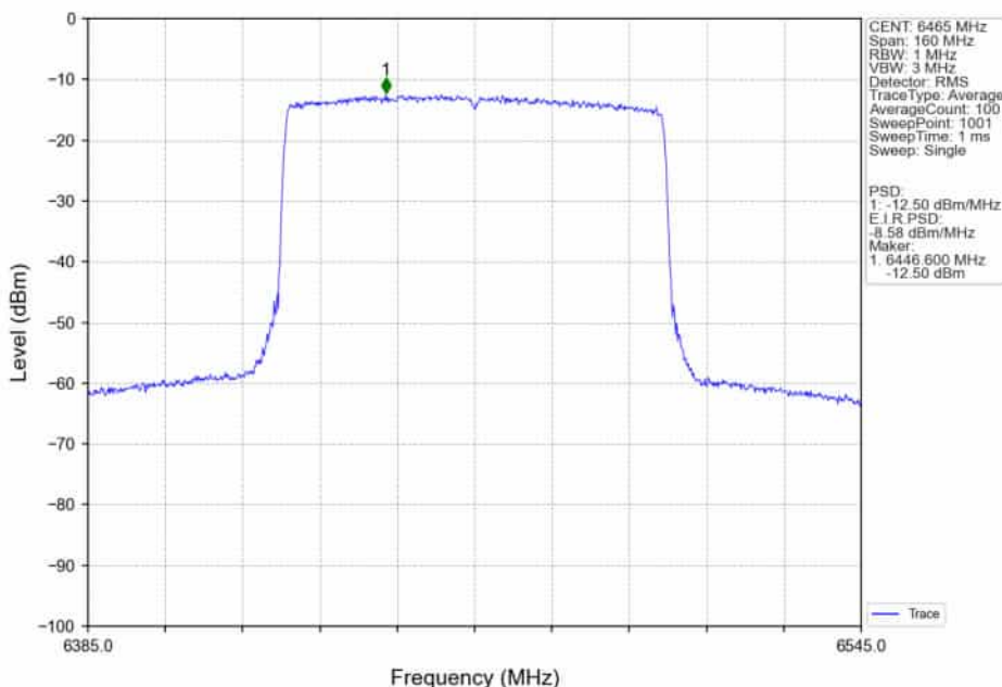
802.11ax(HEW80)_LCH_6465MHz_RU996_Left_MIMO_NTNV
