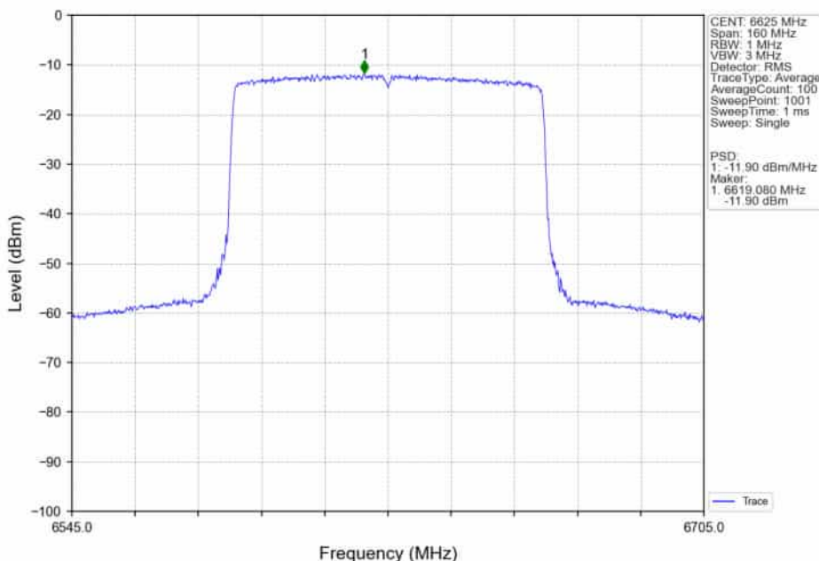
802.11ax(HEW80)_LCH_6625MHz_RU996_Left_Ant2_NTNV
