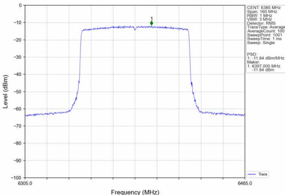
802.11ax(HEW80)_HCH_6385MHz_RU996_Left_Ant2_NTNV
