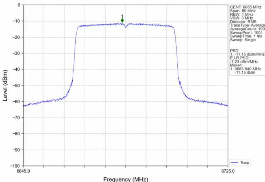
802.11ax(HEW40)_MCH_6685MHz_RU484_Left_Ant2_NTNV
