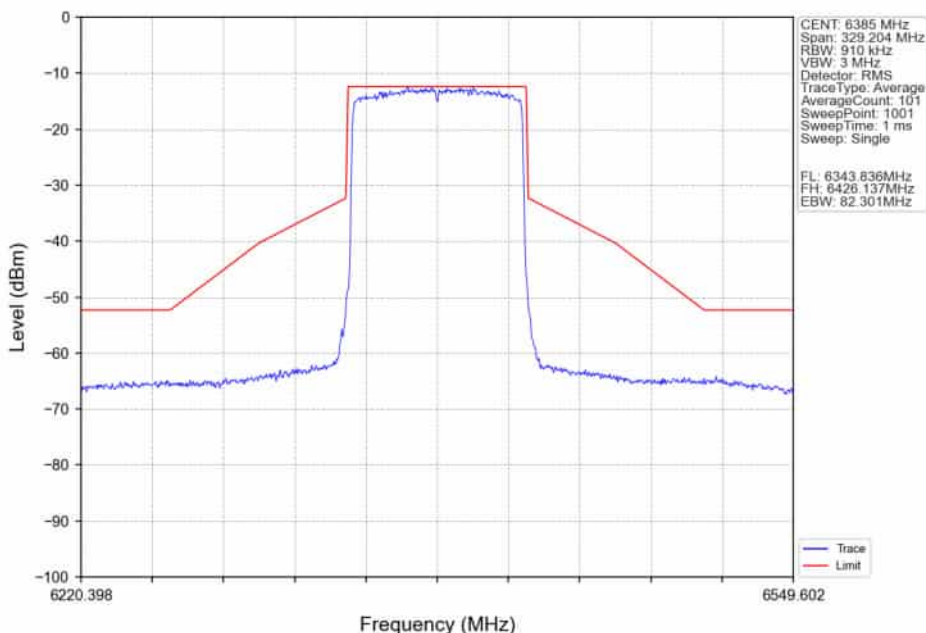
802.11ax(HEW80)_HCH_6385MHz_RU996_Left_Ant2_NTNV
