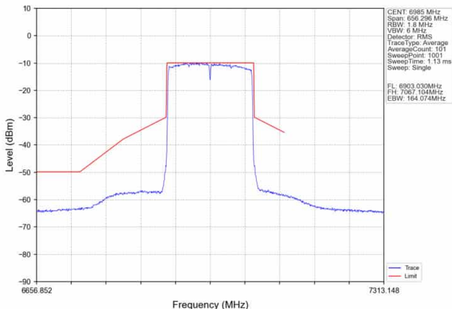
802.11ax(HEW160)_MCH_6985MHz_2xRU996_Left_Ant2_NTNV
