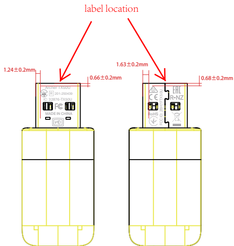
尺寸图
