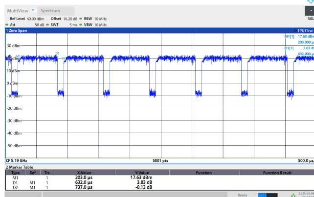
802.11ac(VHT40)
