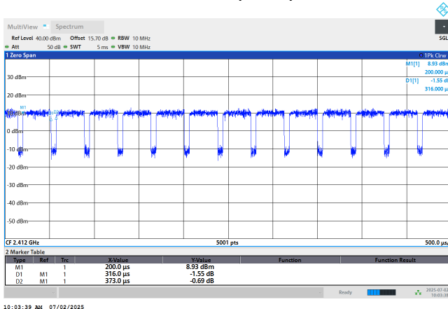
802.11ax(HE20)
