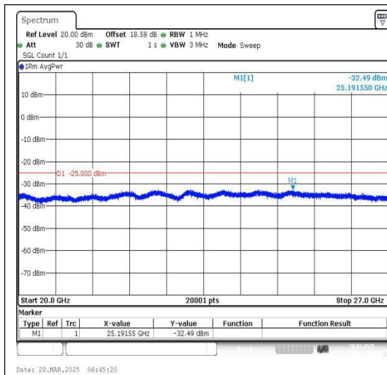
Band7_20MHz_QPSK_20850_1RB#0_20000~27000_000_20000~27000
