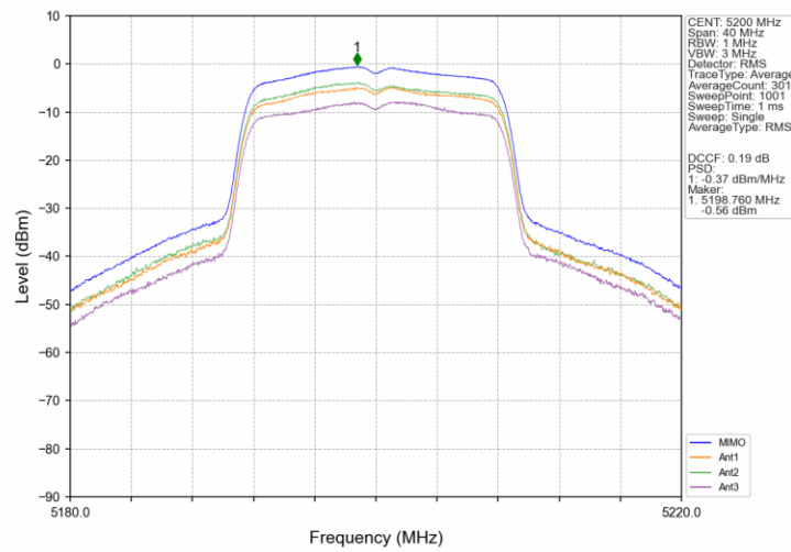
802.11a_MCH_5200MHz_MIMO_NTNV
