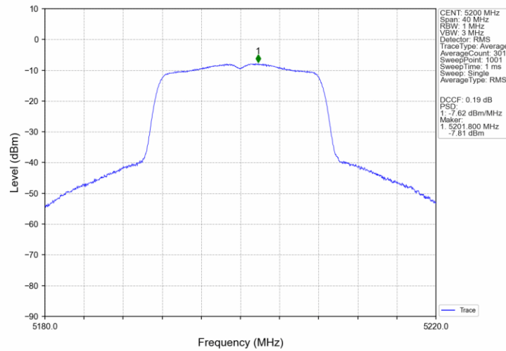
802.11a_MCH_5200MHz_MIMO_NTNV
