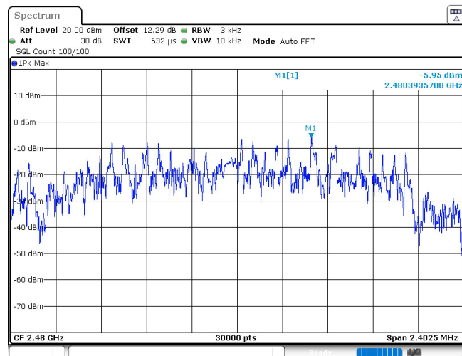
Thread_Ant1_2480
