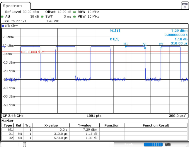
Thread_Ant1_2480
