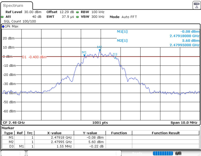
Thread_Ant1_2480
