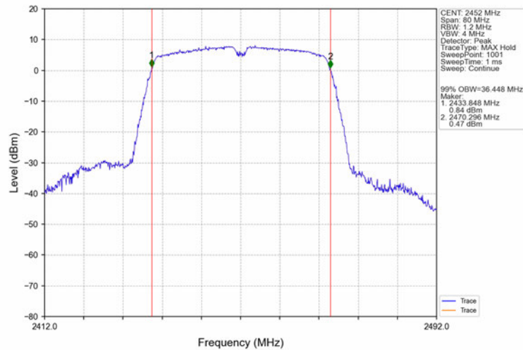
802.11n(HT40)_HCH_2452MHz_Ant1 (SISO)_NTNV
