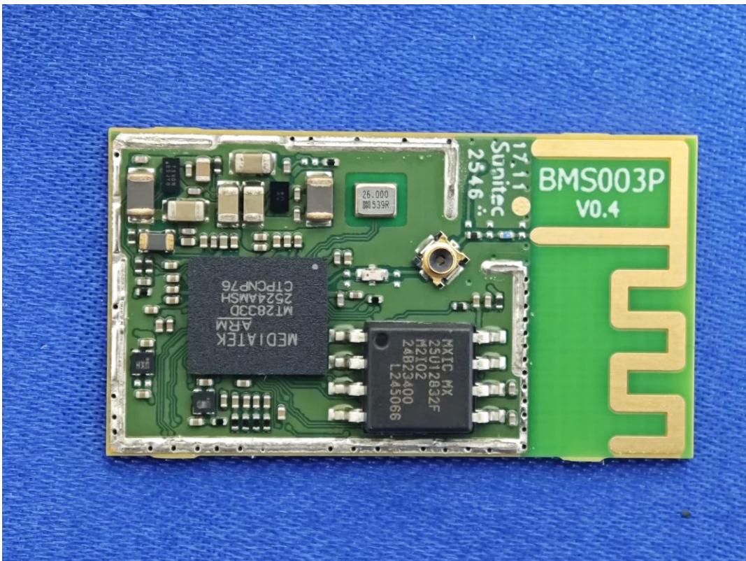
4) EUT Photo
