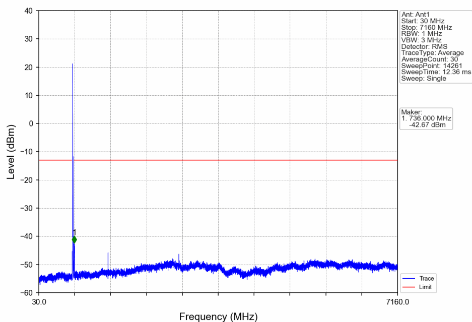
Band12_10MHz_QPSK_MCH_707.5MHz_RB_1_0_NTNV
