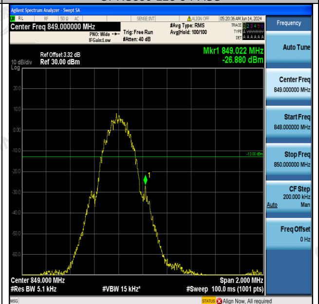
GPRS850-251-5-PASS
