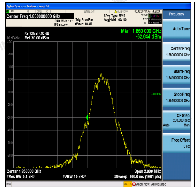
GPRS1900-512-0-PASS
