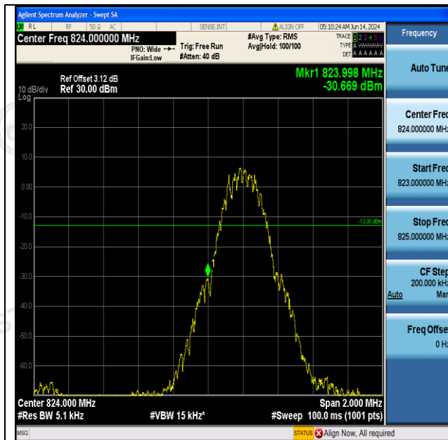
GSM850-128-5-PASS
