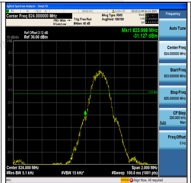
GPRS850-128-5-PASS
