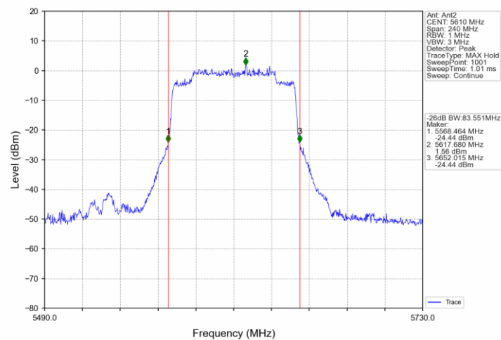
802.11ax(HEW80)_HCH_5610MHz_Ant2_NTNV
