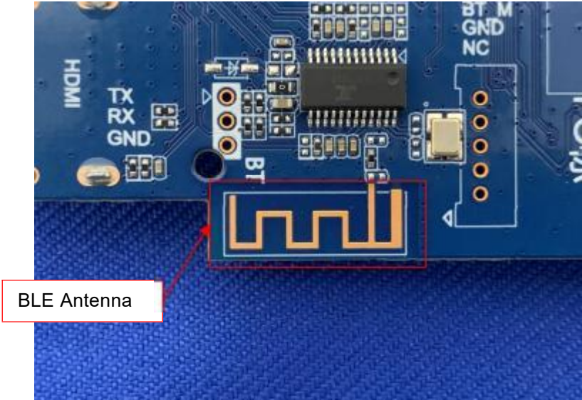
EUT Photo
