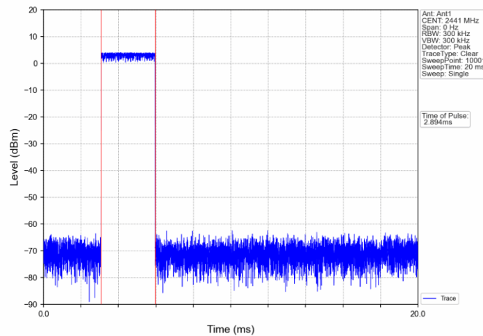
GFSK_DH5_HOPP_Ant1_NTNV
