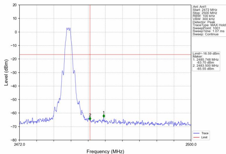
1M_HCH_2480MHz_ANT_1_NTNV
