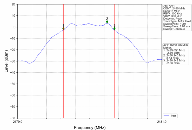
1M_HCH_2480MHz_ANT_1_NTNV
