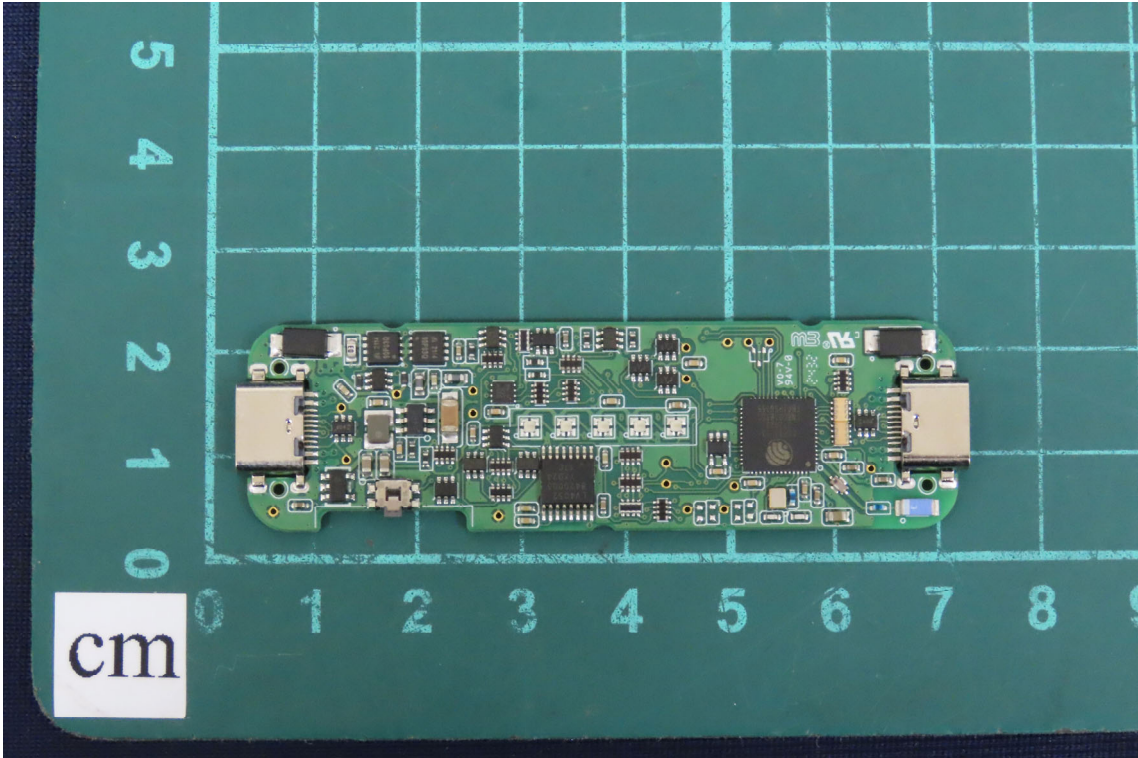
(5) EUT Photo
