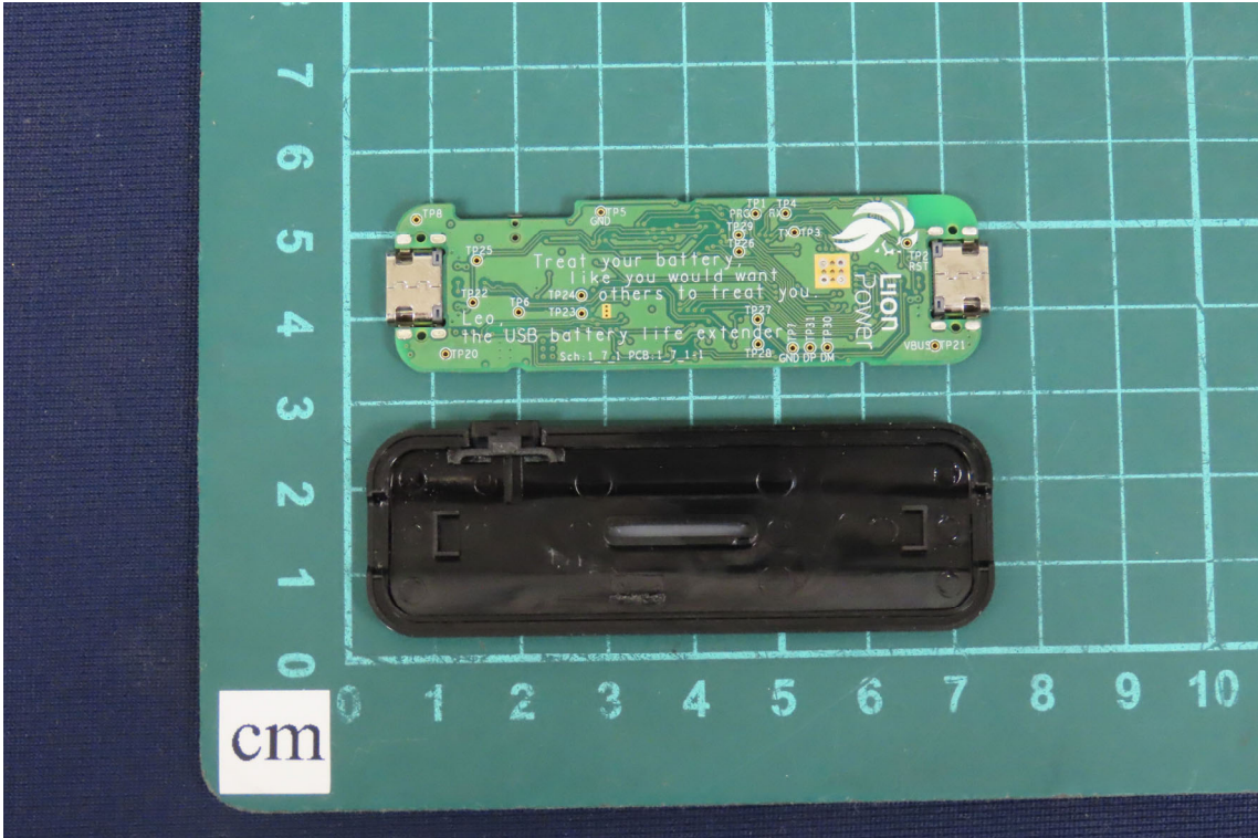
(3) EUT Photo
