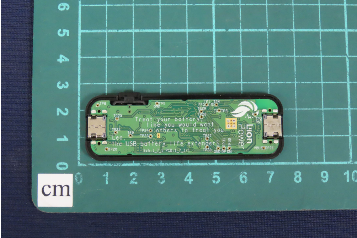
(2) EUT Photo
