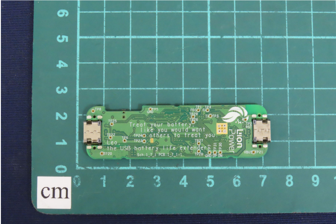
(4) EUT Photo
