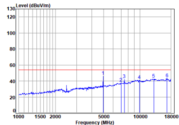
BLE_1M_TX_CH_39_Vertical-Avg
