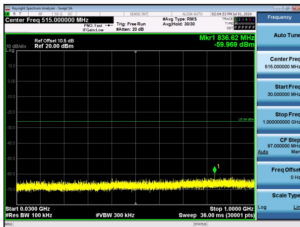
11G-Ant1-2462-30~1000-PASS
