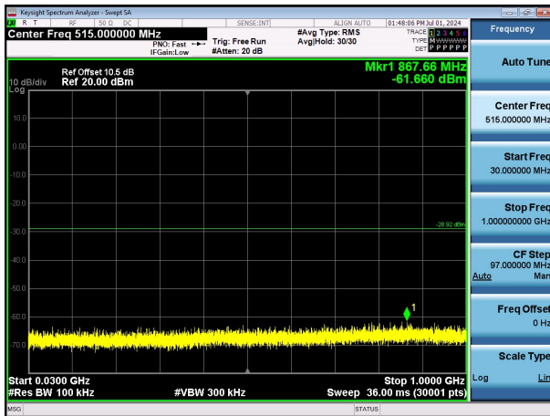
11G-Ant1-2412-30~1000-PASS
