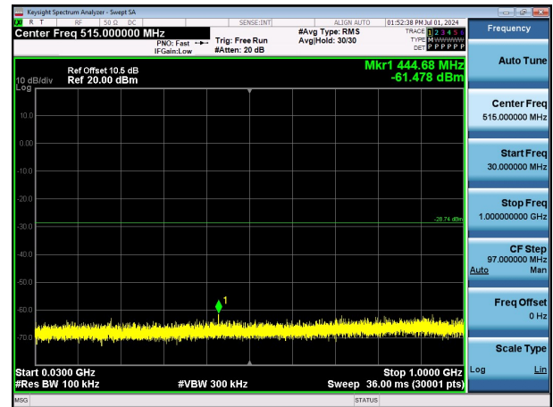
11G-Ant1-2437-30~1000-PASS
