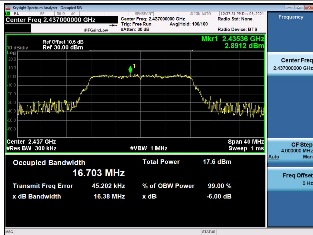
11G-Ant1-2437
