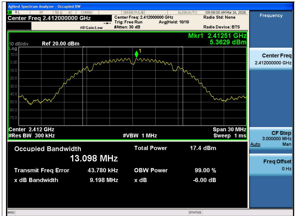
Test_Graph_802.11b_ANT2_2412_1Mbps_DTSSBW
