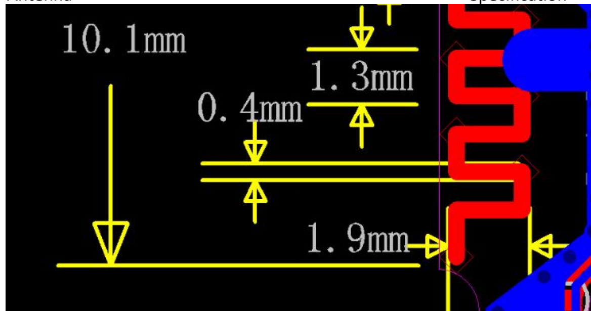
Antenna
