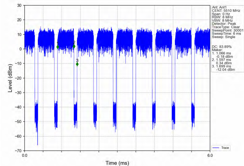
802.11ax(HE40)_LCH_5510MHz_RU484_Left_Ant1_NTNV
