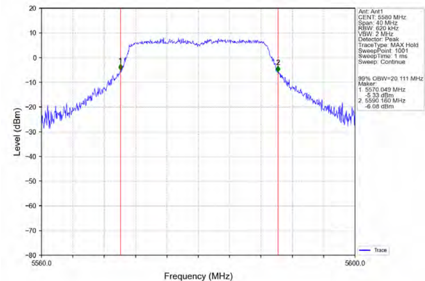
802.11n(HT20)_MCH_5580MHz_Ant1_NTNV
