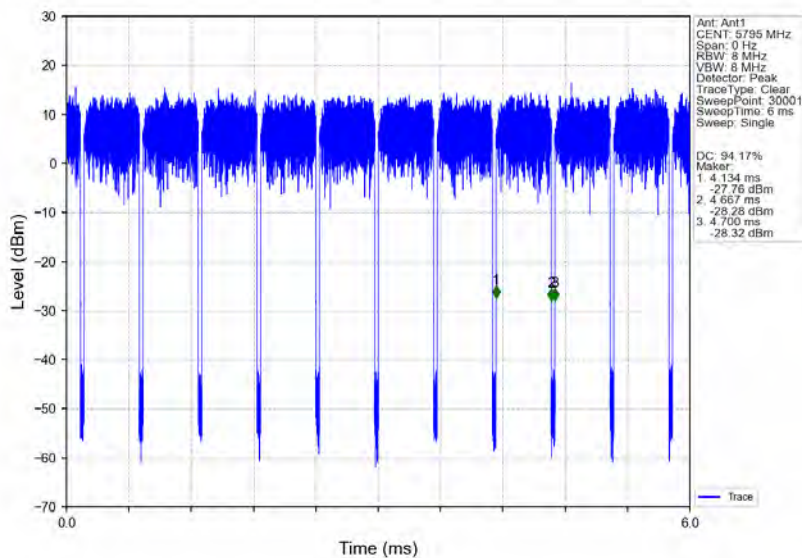
802.11ax(HE40)_HCH_5795MHz_RU484_Left_Ant1_NTNV
